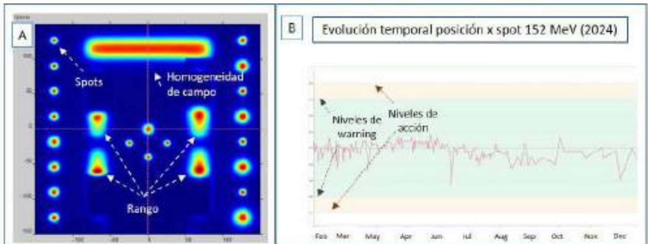
Figura 1. (A) Imagen representativa del mapa de spots que se obtiene en el QA diario, tomada con el detector Lynx y analizada con el software MyQA (IBA Dosimetry). (B) Control chart generado con la aplicación QATrack+ del parámetro posición x del spot 152 MeV. Se puede ver los niveles de warning (franjas naranjas) y niveles de acción, y la estabilidad de este parámetro a lo largo del 2024.
