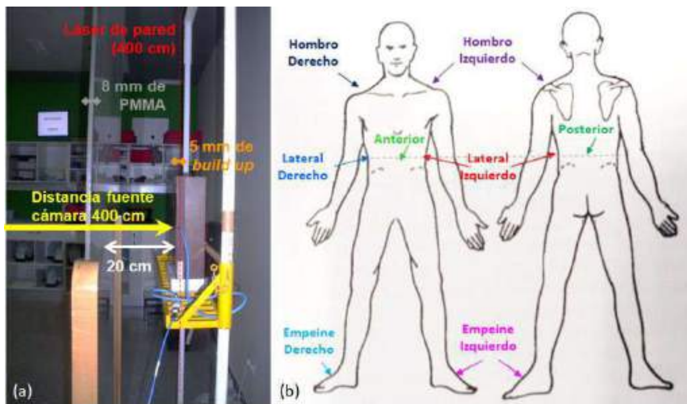
Figura 1. Montaje experimental utilizado para la calibración de diodos (a) y localización de puntos anatómicos de medida (b) para tratamientos TSET.
