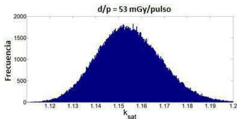
Figura FIGURA 1 : Distribución del \sqrt{dpi100/fn_cm/smallk_{sat}} para la cámara de ionización plano-paralela (PPC40)
