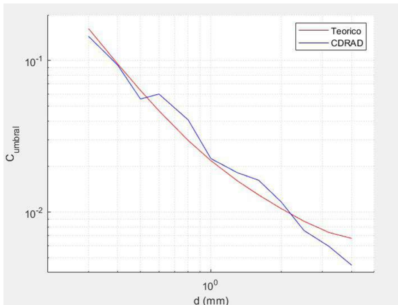
FIGURA 1. Comparación de la curva contraste-detalle obtenida con el maniquí CDRAD y con el método alternativo (NPWE). Discusión
