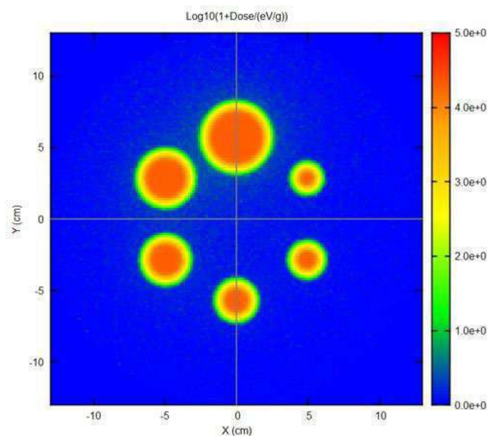
Figura 1. Distribución de dosis absorbida en el plano de las esferas.
