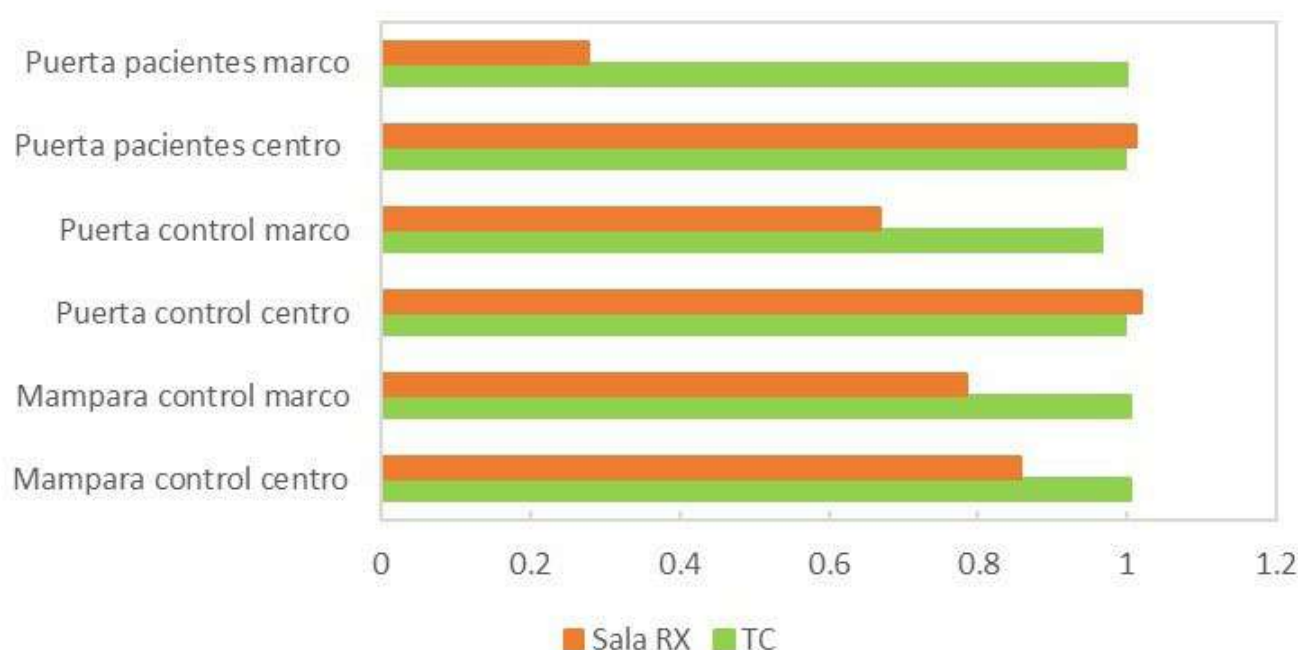
FIG. 2 Se representa el cociente de las tasas medidas con ambos detectores, en las dosimetrías de área realizadas en la sala de RX convencional (con tiempos de disparo de 0.5 s) y en la sala del TC (con tiempos de disparo de 5 s).
