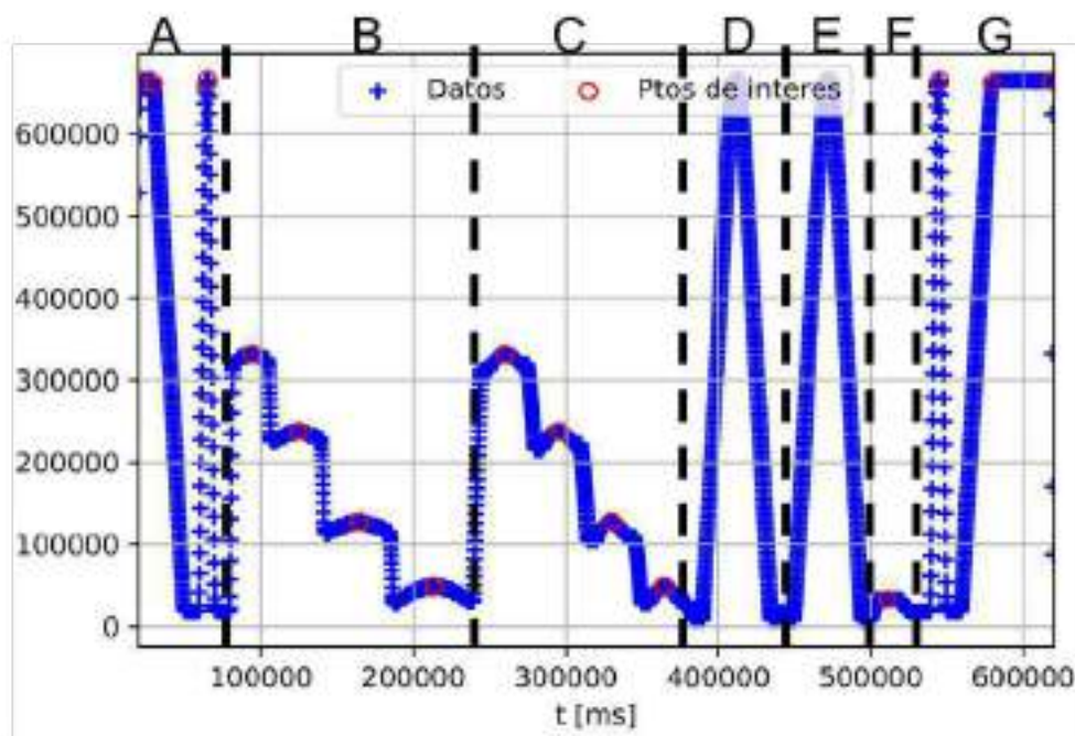
Imagen 1: Prueba Barrido de Mordaza – Mordaza Dinámica. Los puntos rojos son los máximos locales que se usarán para el análisis de las diferentes pruebas, a destacar el A y G (Precisión temporal) y D y E (Barrido de mordaza trasera y delantera, respectivamente).
