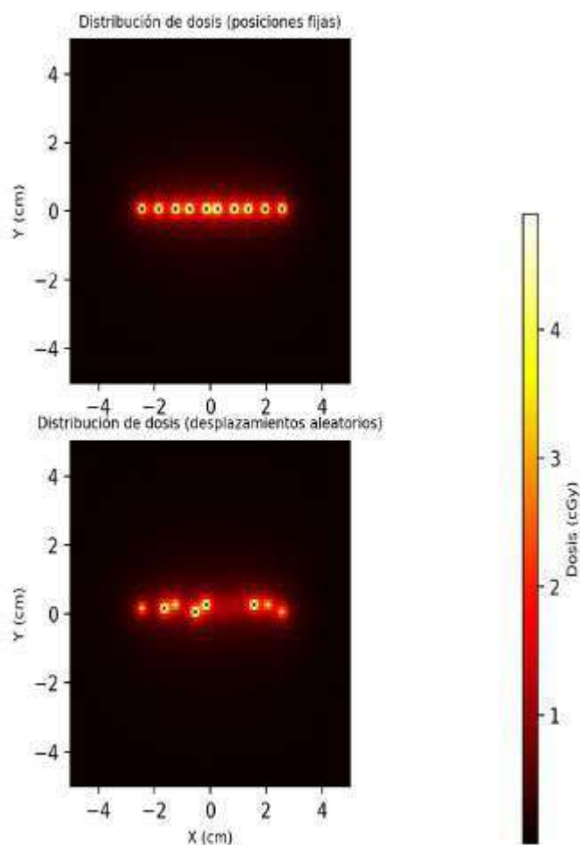
Fig1-Generación de las matrices de dosis, la original y la modificada en los puntos de parada de fuente, en una distancia aleatoria de 0.5 mm
