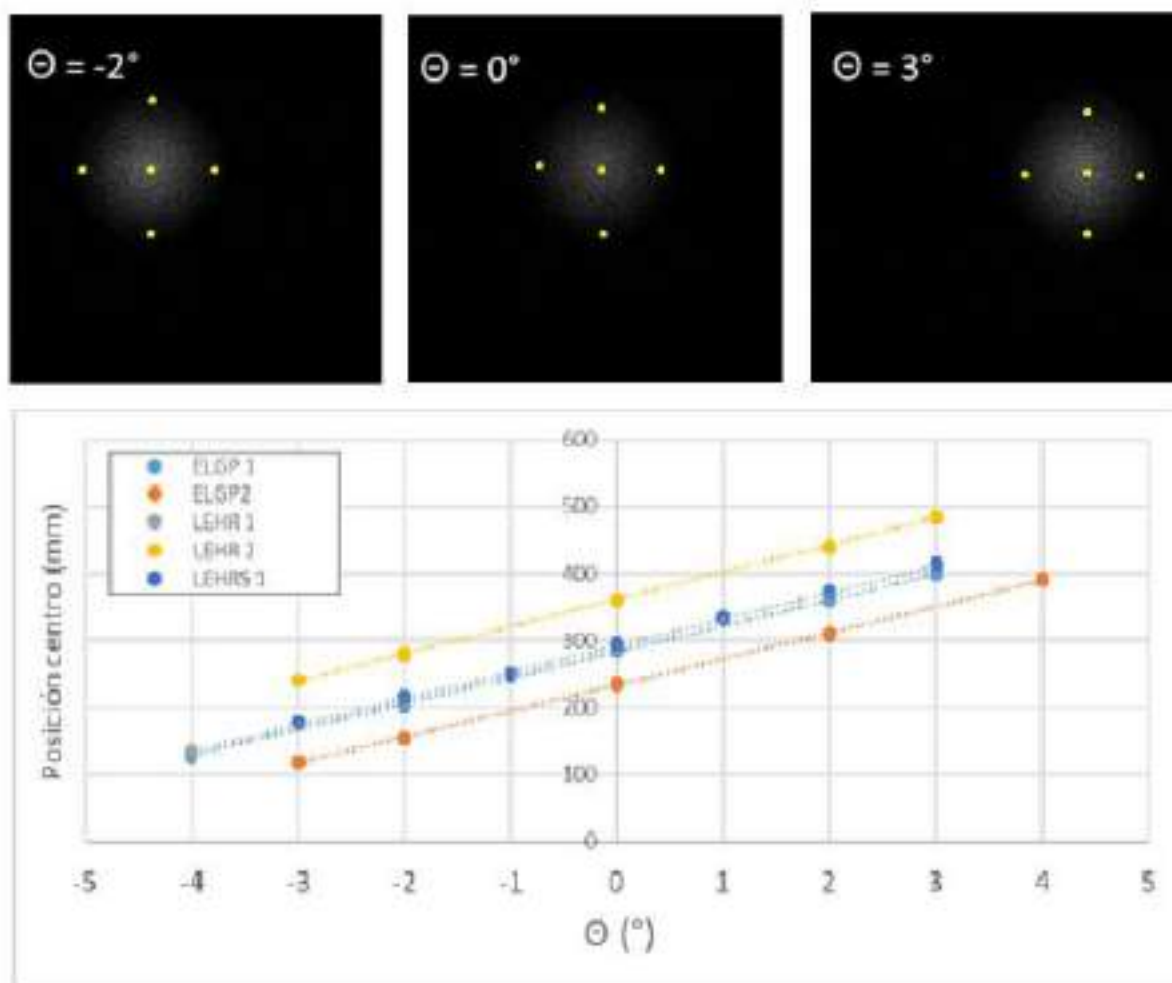
Figura 2. Coordenadas del máximo de la distribución respecto al ángulo de giro.
