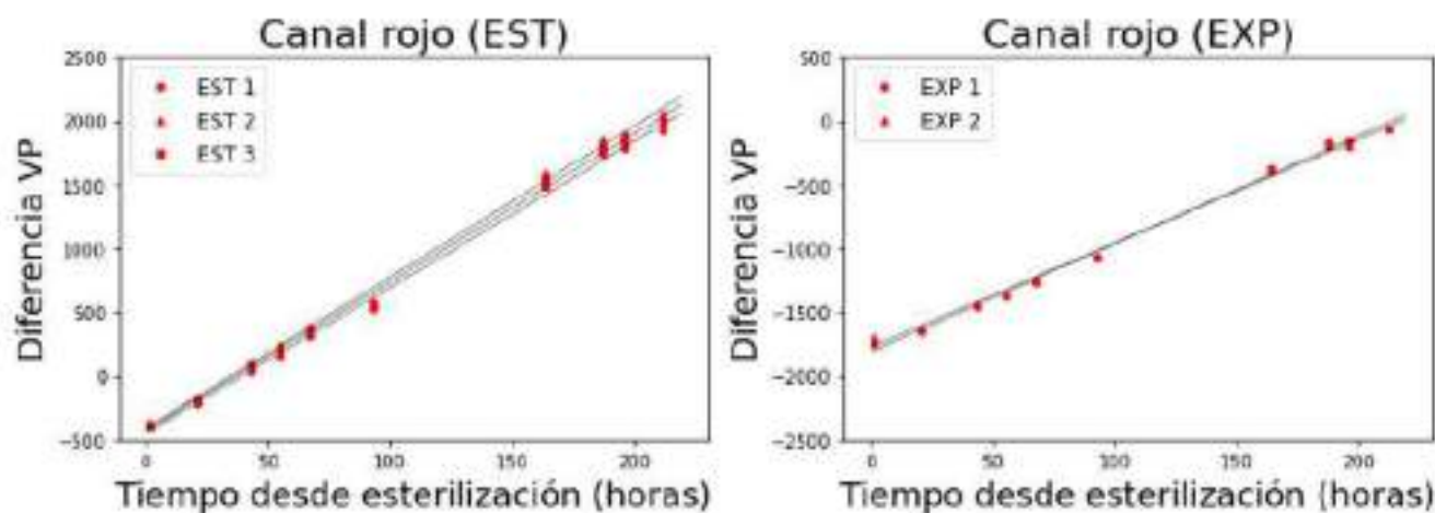
Figura 1. Evolución temporal de la diferencia del VP del canal rojo entre las películas esterilizadas y la película control, para diferentes ciclos estándar (EST 1, EST 2 y EST 3) a la izquierda y ciclos exprés (EXP 1 y EXP 2) a la derecha. Las barras de error no se muestran para facilitar la visualización, con valores entre 40 y 70 PV. La discrepancia entre el rango de valores de ambas gráficas se debe al uso de dos lotes distintos.
