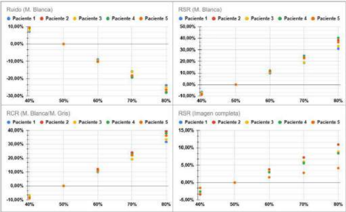
FIGURA 1. Resultados del análisis cuantitativo. Eje vertical, valores normalizados a los obtenidos para el ASiR50%. Eje horizontal, %ASiR.
