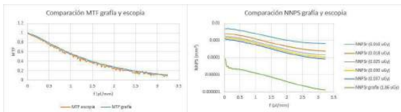
FIGURA 2. MTF y NNPS en modo gráfia y en modo escopía.
