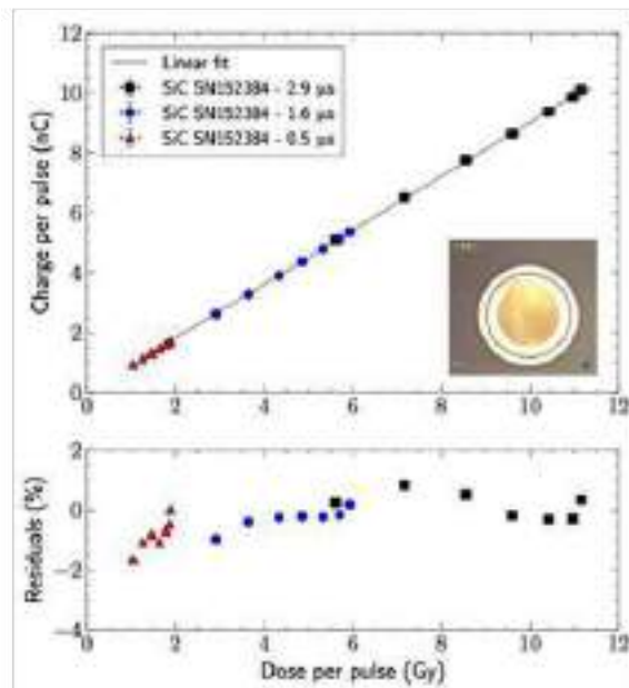
Figura 1. Izquierda: Linealidad de la sensibilidad demostrada por un diodo de SiC producido en el IMB-CNM probado con pulsos de electrones de 6 MeV [3]. Derecha: Perfil de un haz de protones no-homogéneo de 7 MeV obtenido con una matriz de 2x2 píxeles.
