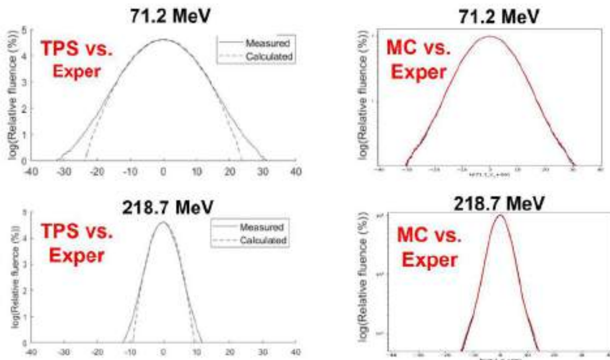
Fig.1 Perfiles transversales en aire
