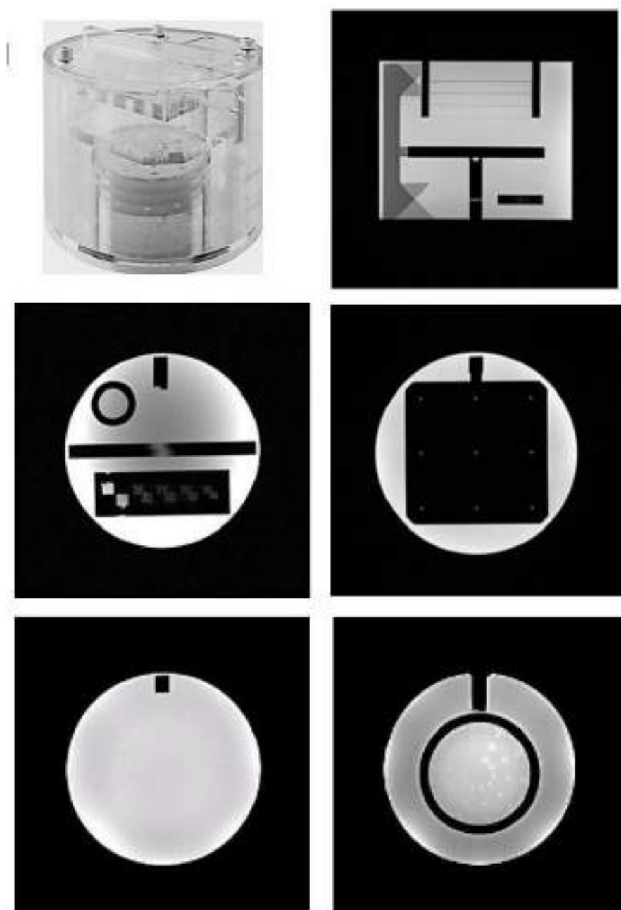
Figura 1. Fantoma ACR médium. Cortes de los objetos de test para evaluación de la resolución espacial, la distorsión geométrica, la uniformidad y la resolución a bajo contraste.
