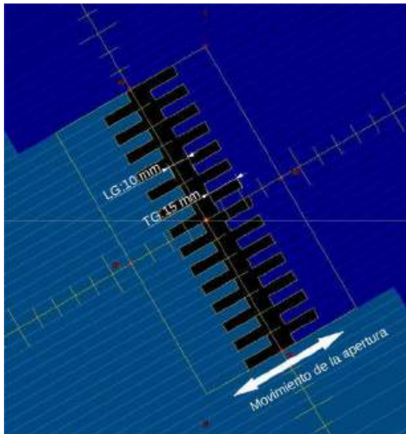
FIGURA 1: Imagen de una apertura de prueba con LG=10 mm y TG= 15 mm.
