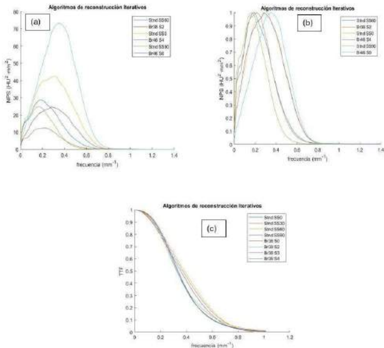
FIGURA 1. (a) Curvas NPS. (b) Curvas NPS normalizadas al máximo. (c) TTF calculada a partir del inserto de aire.
