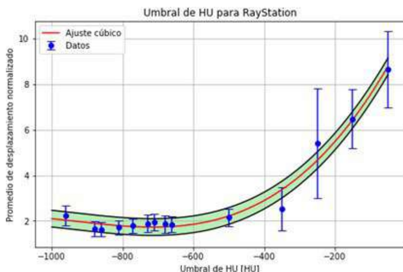
FIGURA 1: Análisis del umbral de HU con ajuste cúbico y nivel de confianza del 95% utilizado para generar los BODY en Raystation.
