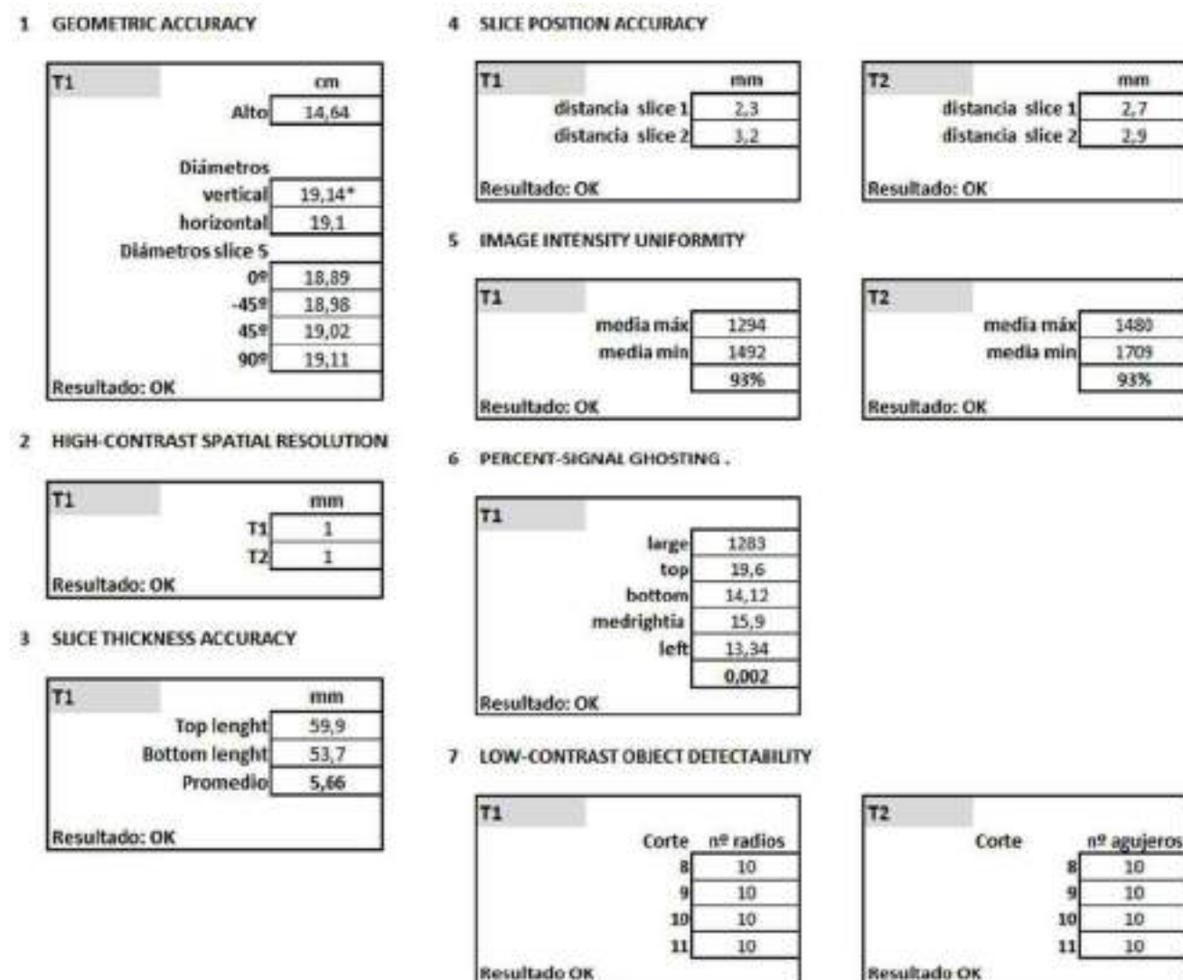
Figura 2. Resultados de las pruebas ACR para la aceptación de una resonancia magnética.
