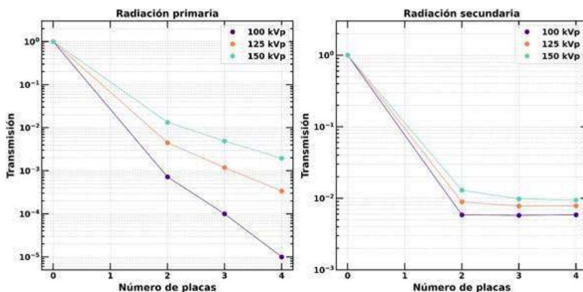
Fig. 1. Medidas de la transmisión para diferentes espesores (número) de placas.
