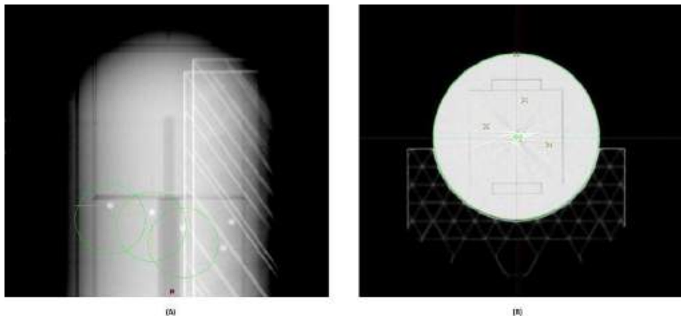
FIGURA 2: (A) Imagen kV de la detección de fiduciales con el Stereophan sobre el maniquí. (B) Imagen CBCT del Stereophan sobre el maniquí.
