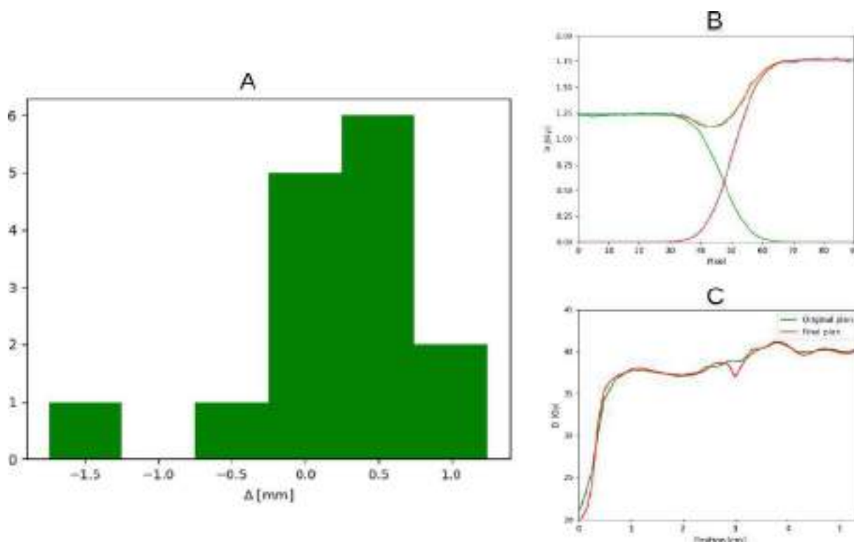
FIGURA 1. (A) \Delta obtenido para todas las sesiones de tratamiento. (B) Ejemplo del ajuste (línea sólida) obtenido a partir de una medición con película radiocrómica (puntos) y la suma de las penumbras (líneas discontinuas). (C) Gráfico de dos perfiles del plan: el verde corresponde al plan original y el rojo al plan suma que considera los diferentes valores de \Delta encontrados.
