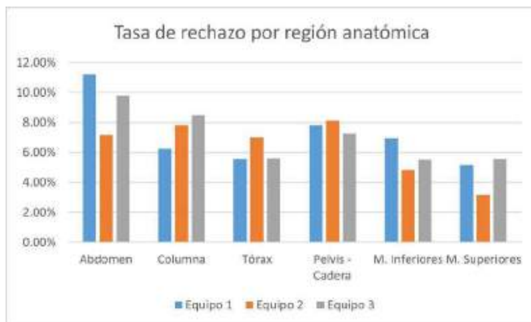
Figura 1. Tasa de rechazo en tanto por ciento por región anatómica para los tres equipos analizados.
