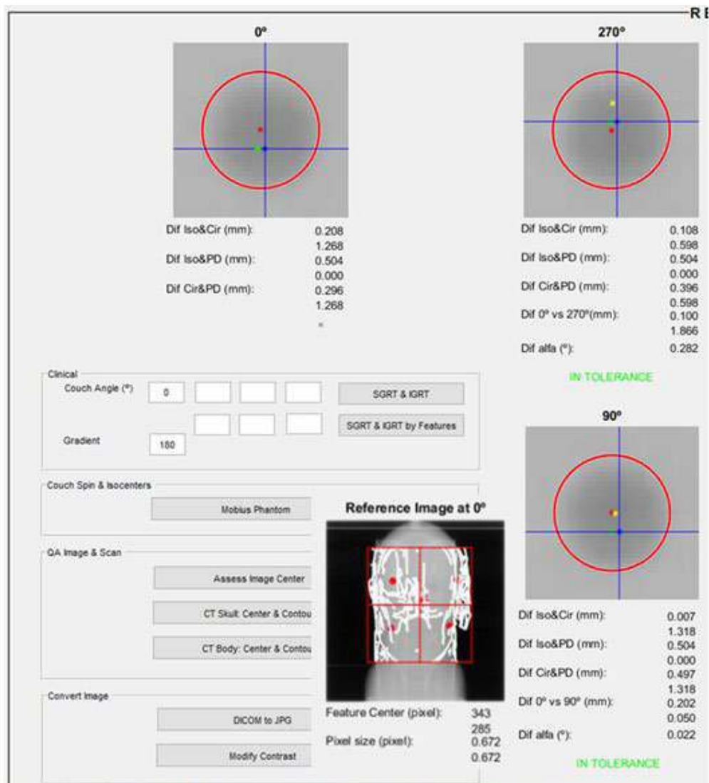
Figura 1. Parte de la vista general del software RESIS-ITS en el modo Couch Spin & Isocenters. La aplicación de software muestra las diferencias en milímetros para los ejes x e y y el ángulo de desviación en grados para cada rotación de mesa en comparación con la imagen de referencia (aquella tomada con mesa a 0°). Dif Iso&Cir es la diferencia entre el Isocentro de Radiación (punto verde) y el Centro del Círculo (punto rojo), Dif Iso&PD representa la diferencia entre el Isocentro de Radiación y el centro del Portal-Imager (línea azul y punto), Dif Cir&PD muestra la diferencia entre el centro del círculo y el centro del Portal-Imager. Dif 0° vs ángulo es la diferencia entre el ángulo de rotación específico de la mesa respecto a la mesa en 0°. Dif alfa (°) es la desviación en el ángulo de la posición de la mesa relacionada con 0°. El centro del círculo en 0° se muestra usando un punto amarillo para cada rotación de la mesa.
