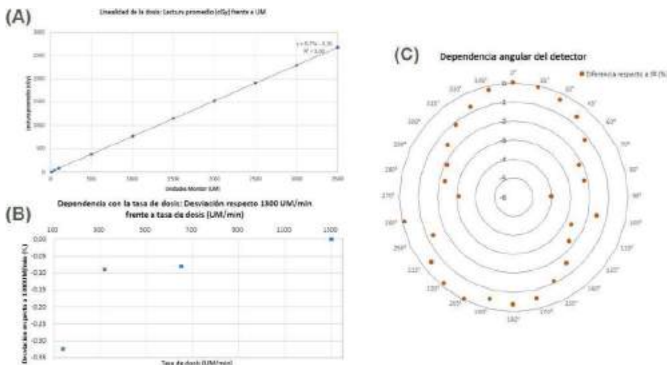
Fig. 1: (A) Linealidad de la dosis. (B) Dependencia de la tasa de dosis. (C) Dependencia angular.
