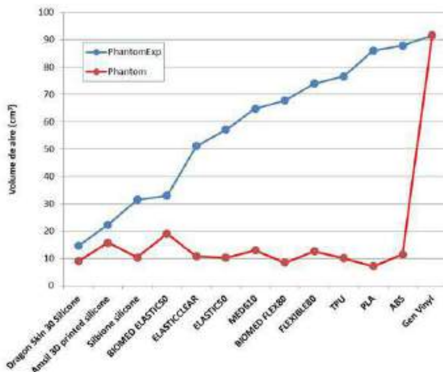
Figura 1. Resultados del test de adaptabilidad. Los valores en rojo representan el volumen de aire medido entre el bolus y el Phantom, mientras que los valores azules indican el volumen de aire entre el bolus y el PhantomExp (maniquí 3mm más grande que el Phantom).
