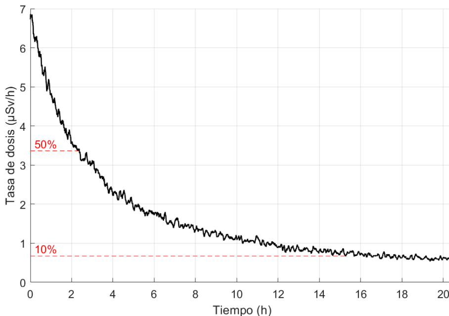
FIGURA 1: Tasa de dosis equivalente frente al tiempo
