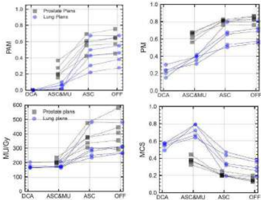
Figura 1: Valores de complejidad para planes de próstata y SBRT de pulmón según la métrica Plan Aperture Modulation (PAM), la relación UM/Gy, Plan Modulation (PM) y Modulation Complexity Score (MCS). Los símbolos representan planes con diferente complejidad y las líneas conectan planes de los mismos casos clínicos. OFF: Sin control; ASC: Aperture Shape Controller en nivel moderado; ASC&MU: ASC en nivel moderado con restricción de UM; DCA: Técnica de Arco Conformal Dinámico.
