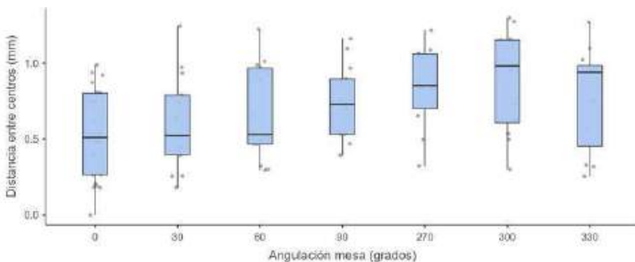
Figura 1: Distancia entre isocentro de radiación y centro de la bola para gantry inmóvil a 0° y diferentes ángulos de giro isocéntrico de mesa.
