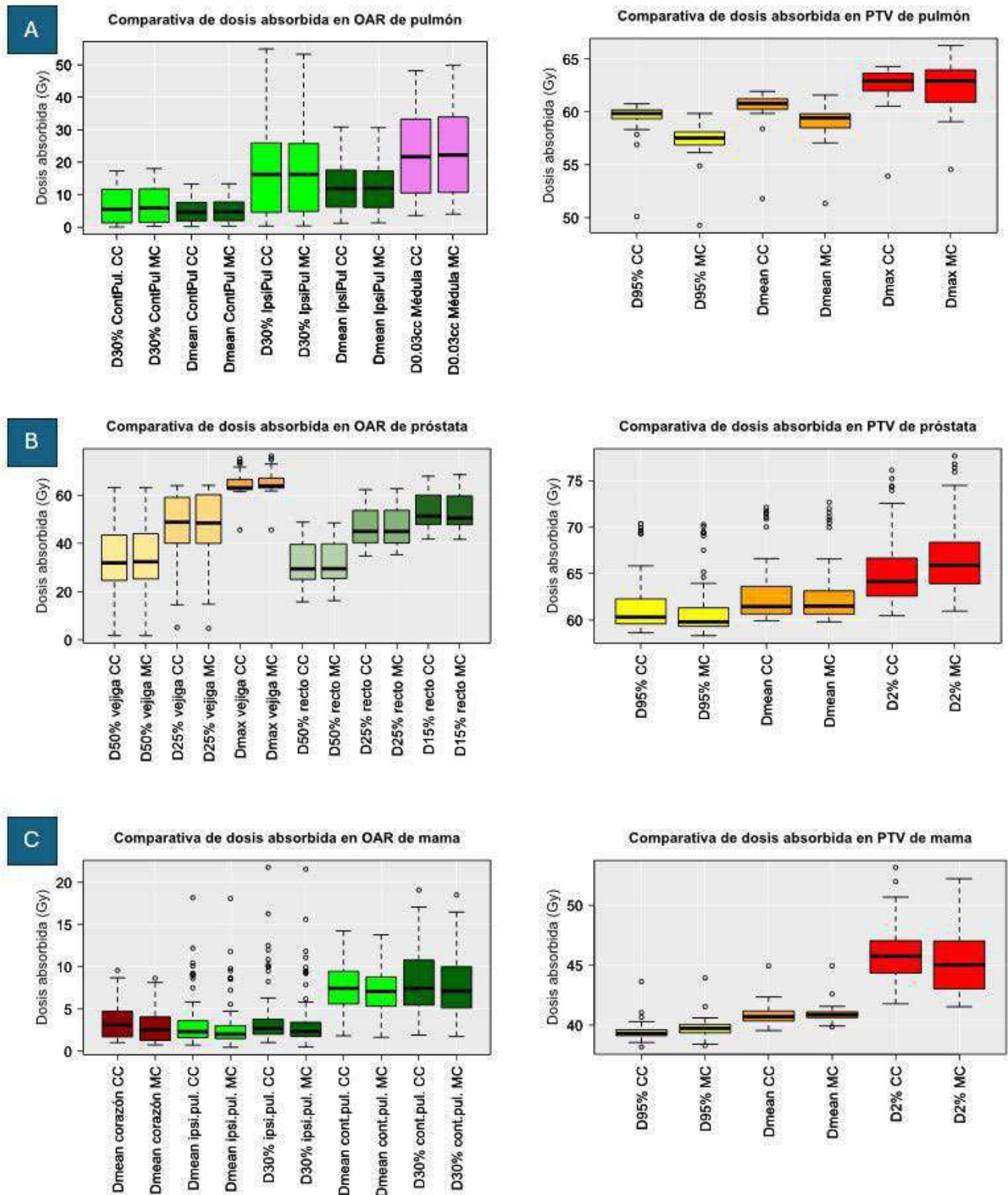
Gráfica 1. Diagrama de cajas de bigotes para comparar resultados obtenidos con algoritmo Collapsed Cone (CC) y algoritmo de Monte Carlo (MC) en tratamientos de pulmón, próstata y mama.
