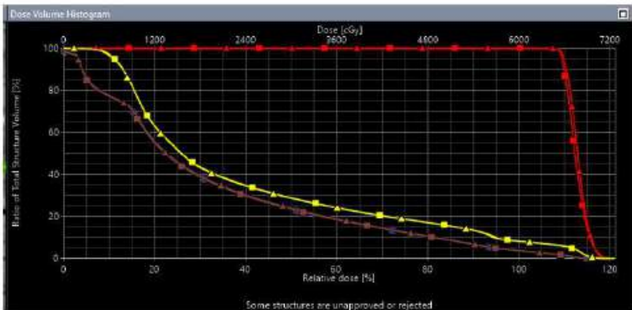
Figura2: HDV para la próstata, vejiga y recto contorneados en el paciente Rando. Plan calculado sobre el CT de planificación con su curva de calibración HU-DRE (triángulos) y sobre el iCBCT (cuadrados) obtenido en el TrueBeam utilizando la curva de calibración HU-DRE para el protocolo Pelvis en condiciones de dispersión estándar.
