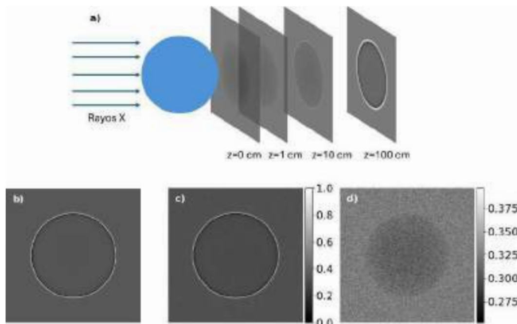
FIGURA 1: a) Esquema de la técnica PBI. Imagen obtenida con: b) cálculos utilizando la propagación de Fresnel, c) simulación MC con ley de Snell, d) simulación MC sin ley de Snell.
