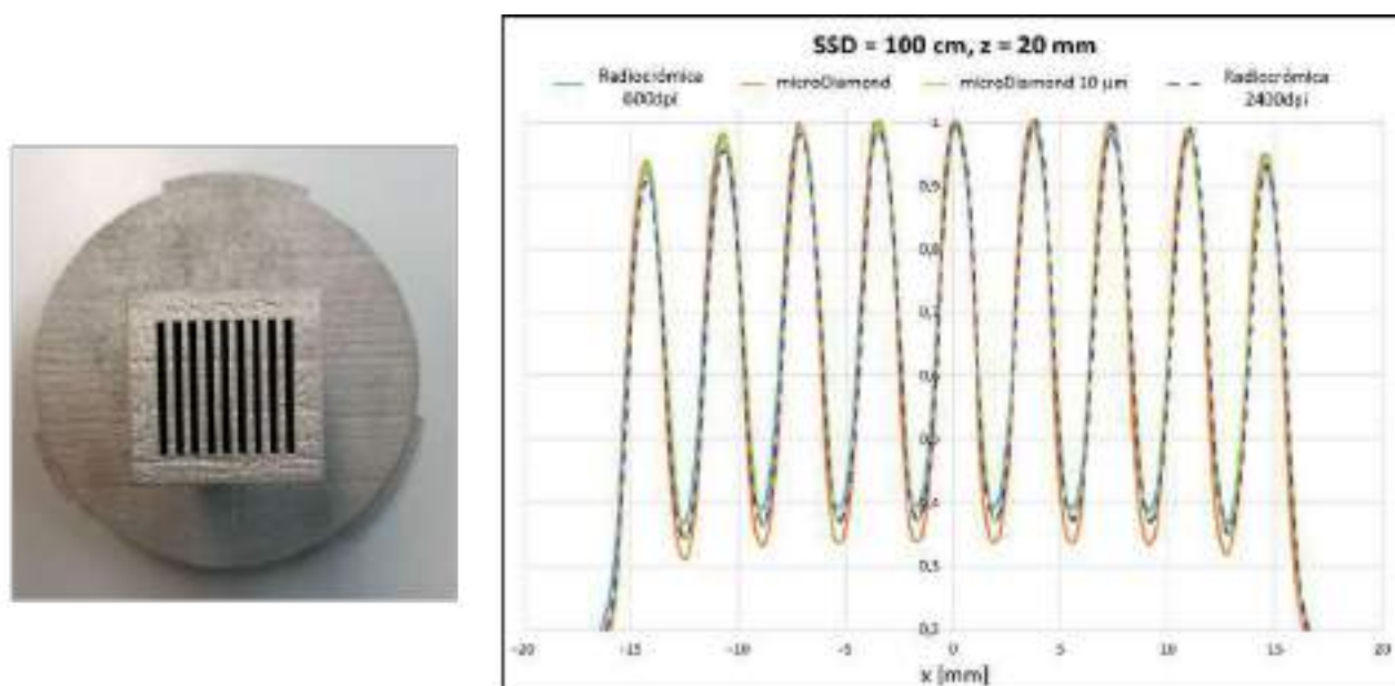
Figura 1: Colimador para conformar campo GRID y campo de radiación producido. Los FWHM de cada pico en isocentro son aproximadamente 1,7mm
