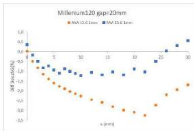
Figura 1: Diferencia de dosis relativa entre las medidas y las dosis calculadas con el TPS en versión 13.6 y 15.6 para el modelo de MLC Millenium120. Test tipo aSG con gap (distancia entre láminas opuestas) de 20mm.
