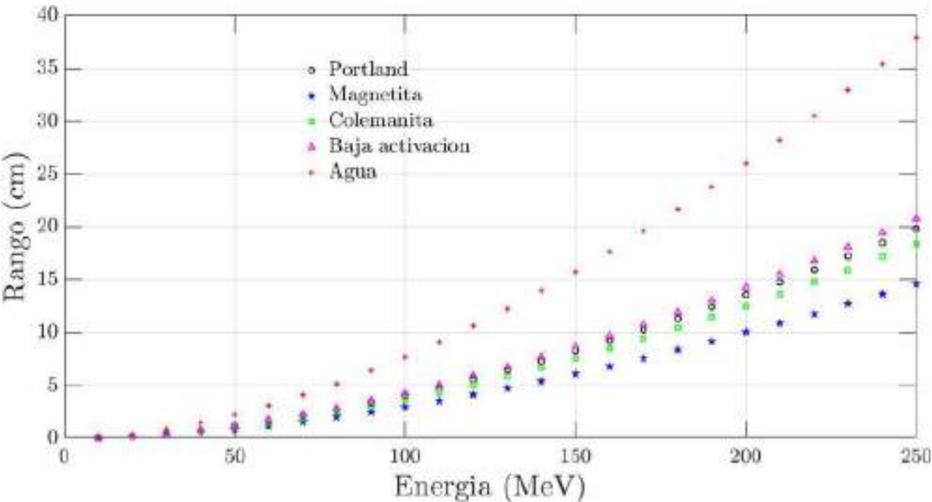
FIGURA 1: Rango (cm) para los hormigones de la tabla 1 hasta 250 MeV. Se representa también el rango del agua.
