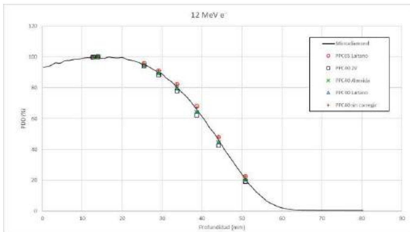
FIGURA 1. PDDs de las distintas cámaras de ionización, comparados con los del detector microDiamond.
