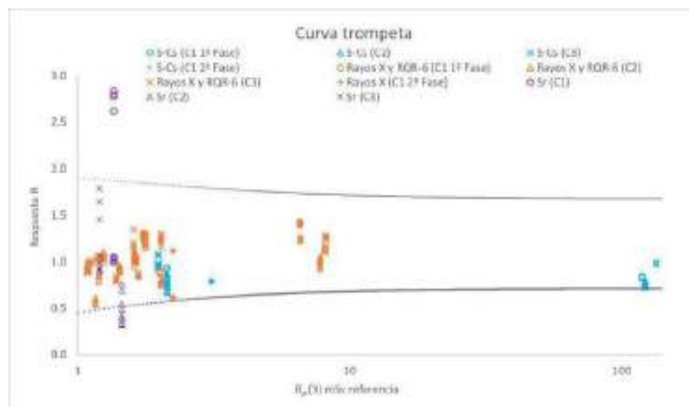
FIGURA 2. Resultado del análisis de la respuesta de todos los ensayos para los centros mediante las curvas trompeta
