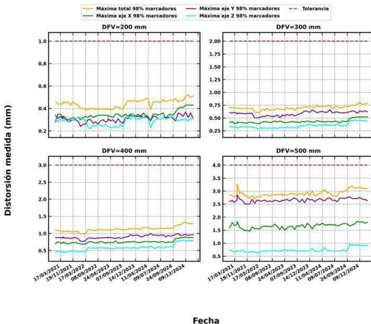
Fig. 2. Estabilidad en el tiempo de la distorsión geométrica.
