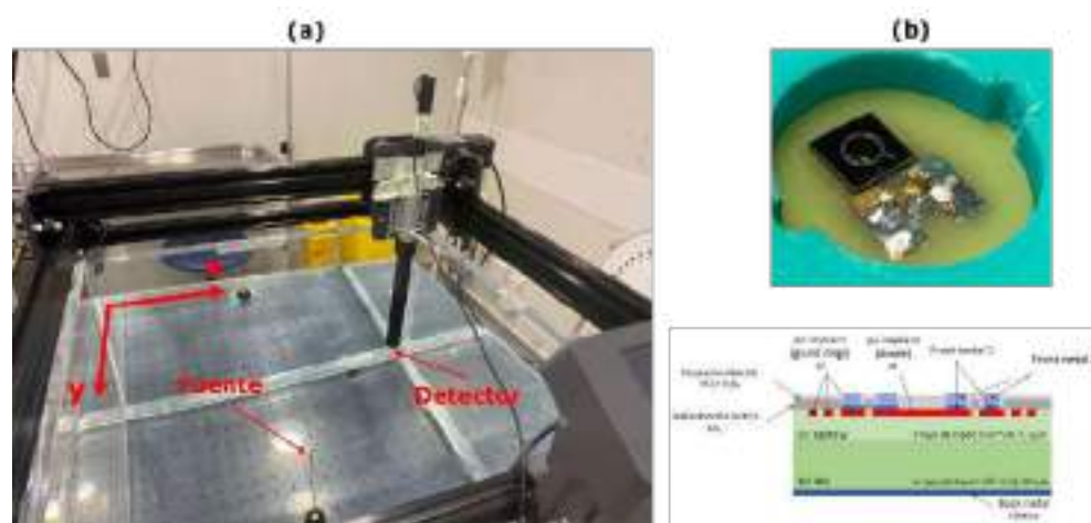
Fotografía del maniquí clínico desarrollado (a). Fotografía y esquema de la estructura del diodo de SiC estudiado (b).
