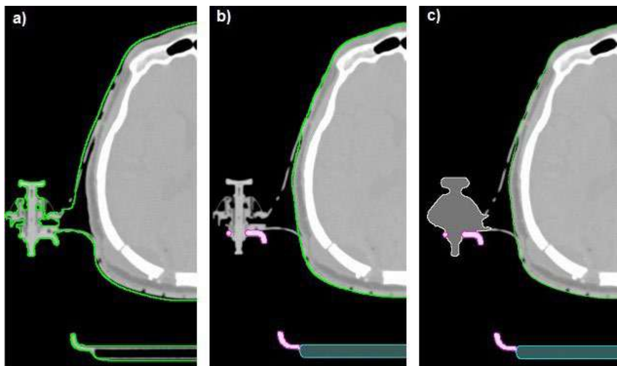
Figura 1. Vistas de los 3 supuestos: a) Encompass en el body , b) Encompass sin el marco, c) Encompass con marco.
