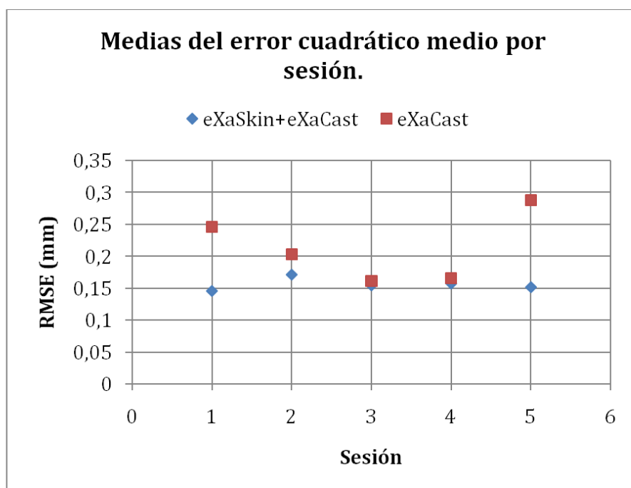
Figura 1: Evolución de la media de RMSE por sesión según tipo de inmovilización
