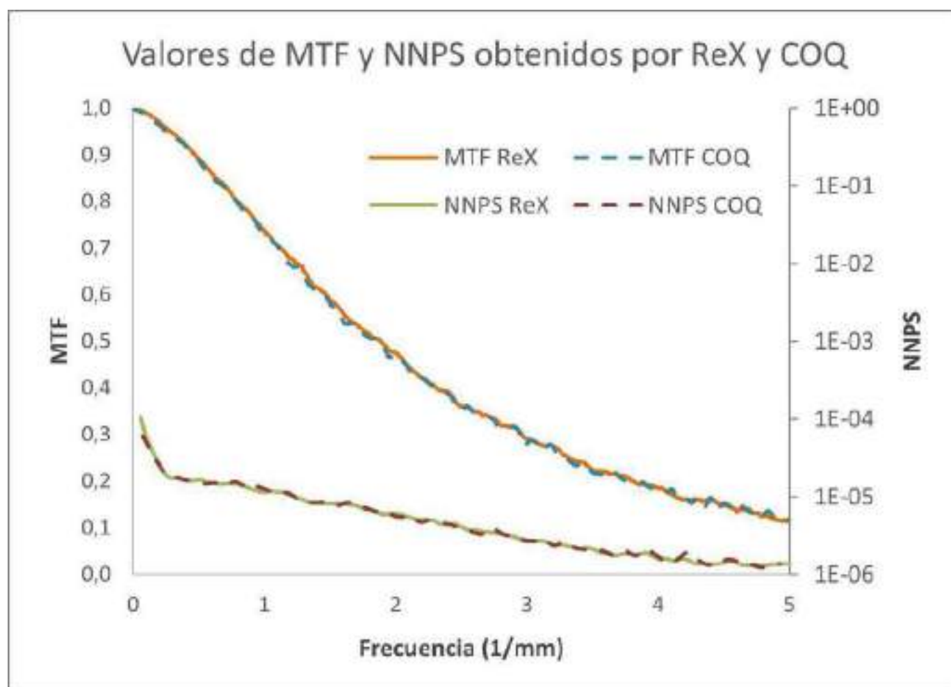
FIGURA 1. Comparación de los valores de MTF y NNPS (proyecciones horizontales) calculados por ReX y COQ.
