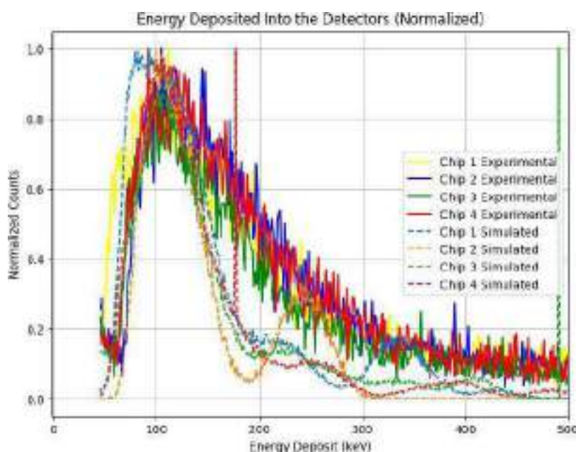
Fig 1. Histograma normalizado del espectro de energía experimental depositado en los chips para el caso que reproduce la dosis distal del 75%.
