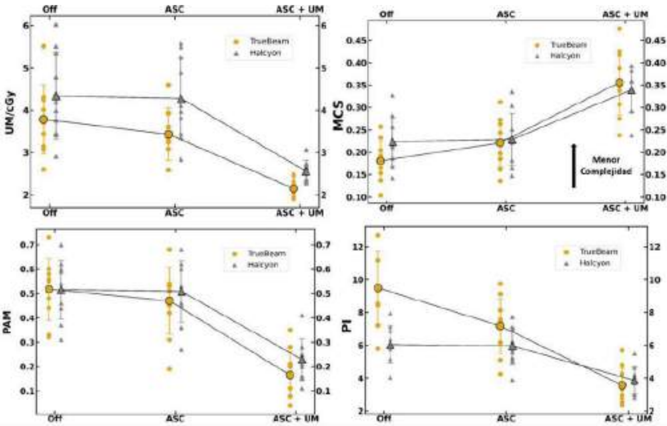
Figura 1. Evolución de las métricas de complejidad en cada una de las etapas de la optimización para las cuatro métricas analizadas: Unidades monitor por centriGray prescrito ( UM/cGy ), Plan Aperture Modulation ( PAM ), Modulation Complexity Score ( MCS ) y Plan Irregularity ( PI ).
