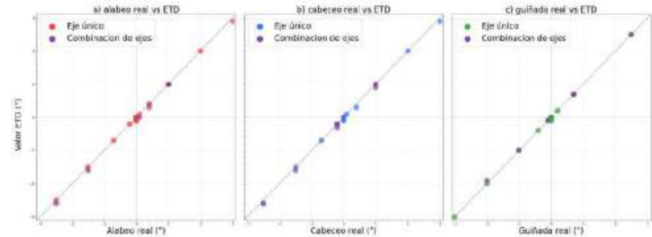
Figura 2: Relación entre el valor de rotación propuesto por ETD y el valor real impuesto en la imagen de referencia para alabeo (a), cabeceo (b) y guiñada (c). La línea recta corresponde a la perfecta identidad.
