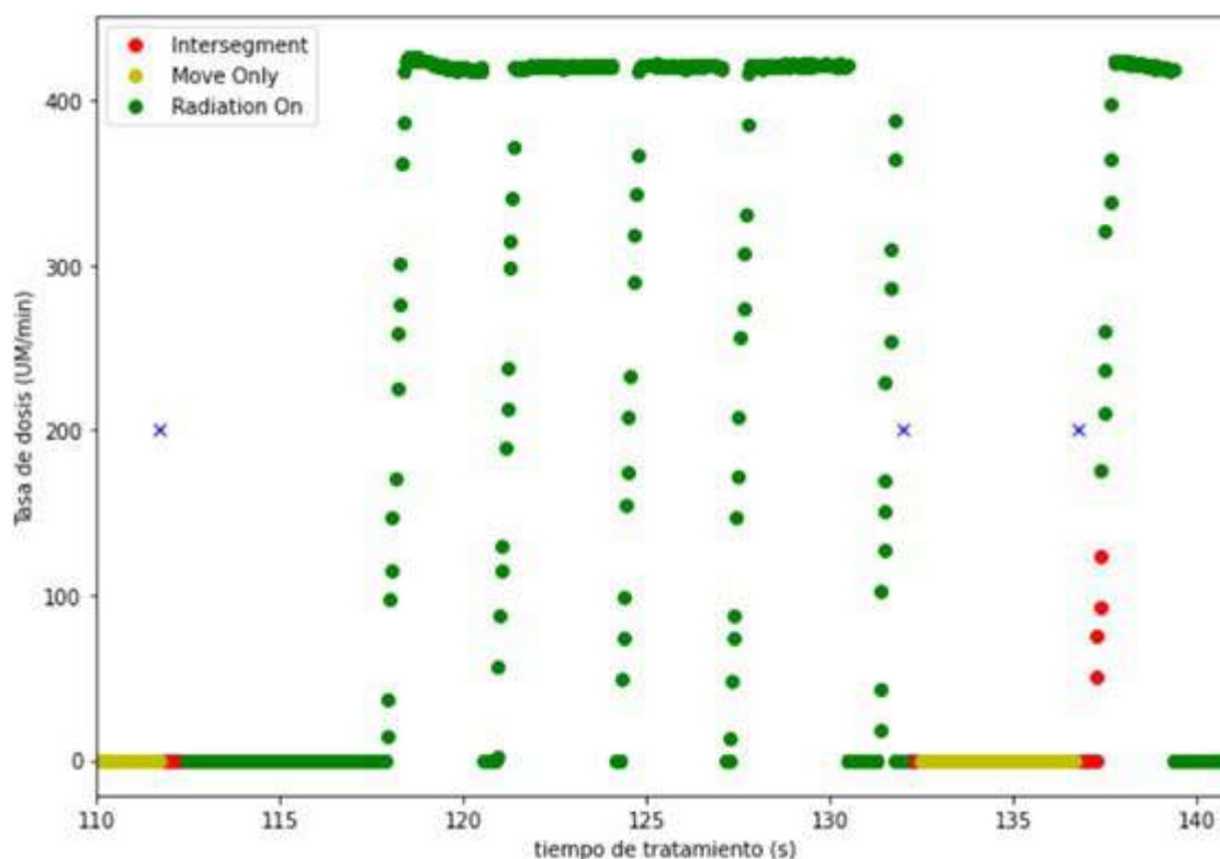
FIGURA 2. Tasa de dosis, distinguiendo los tres estados. Cruces azules: puntos de control.
