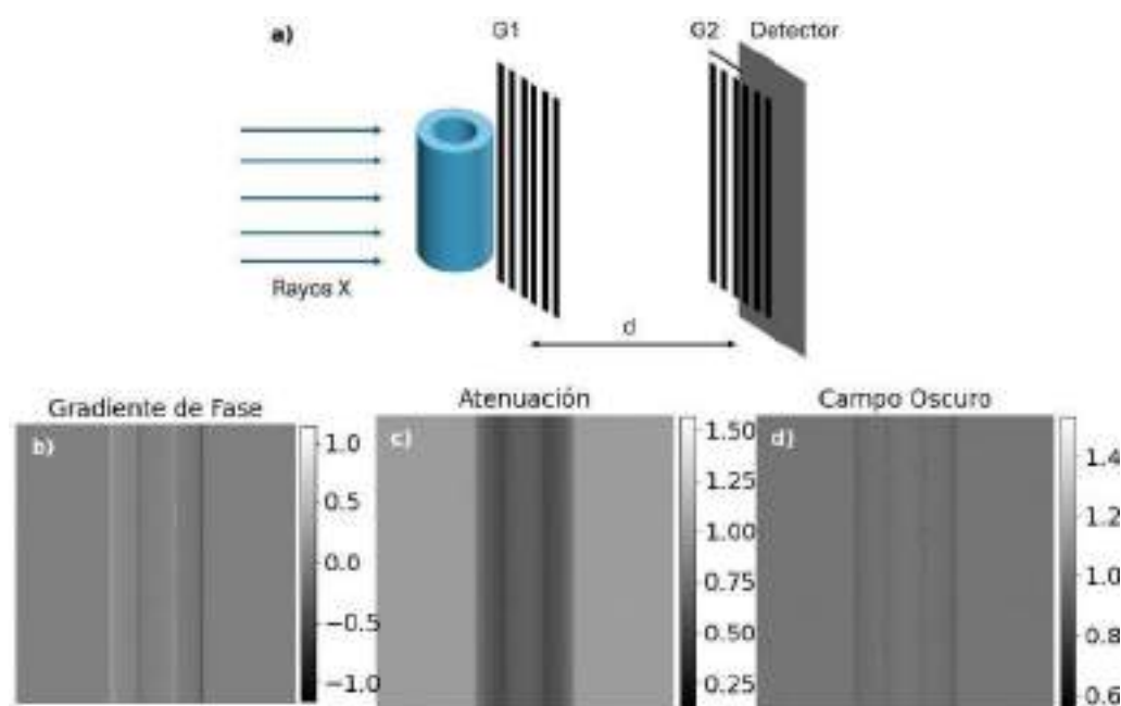
FIGURA 2: a) Esquema de la técnica GBI. Resultado de la simulación de la técnica GBI con el plug-in desarrollado (escala arbitraria).
