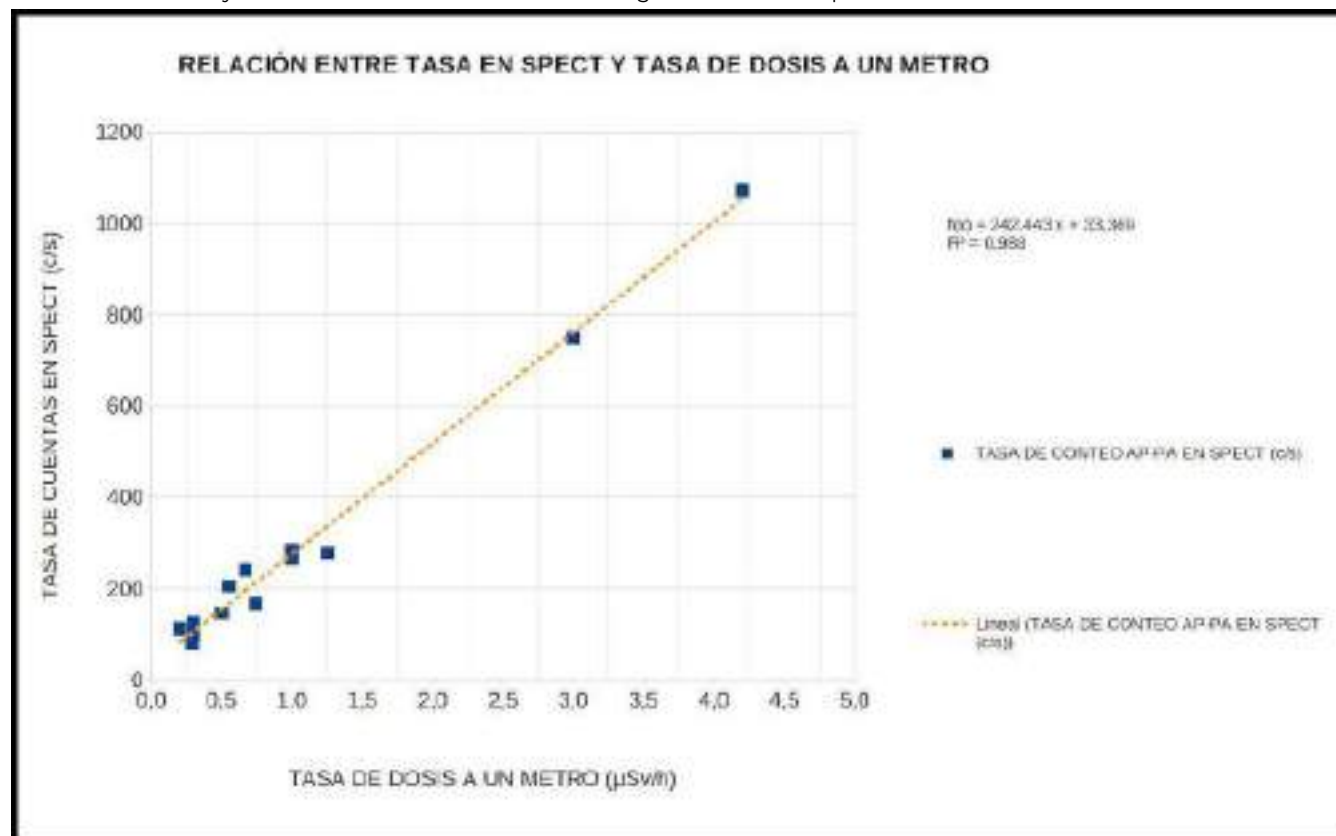
Gráfica 1. Relación entre las medida de tasa de dosis a un metro y la tasa de cuentas obtenida en la adquisición planar.
