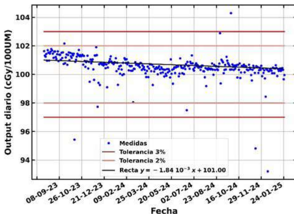
Fig. 2. Estabilidad del output diario.
