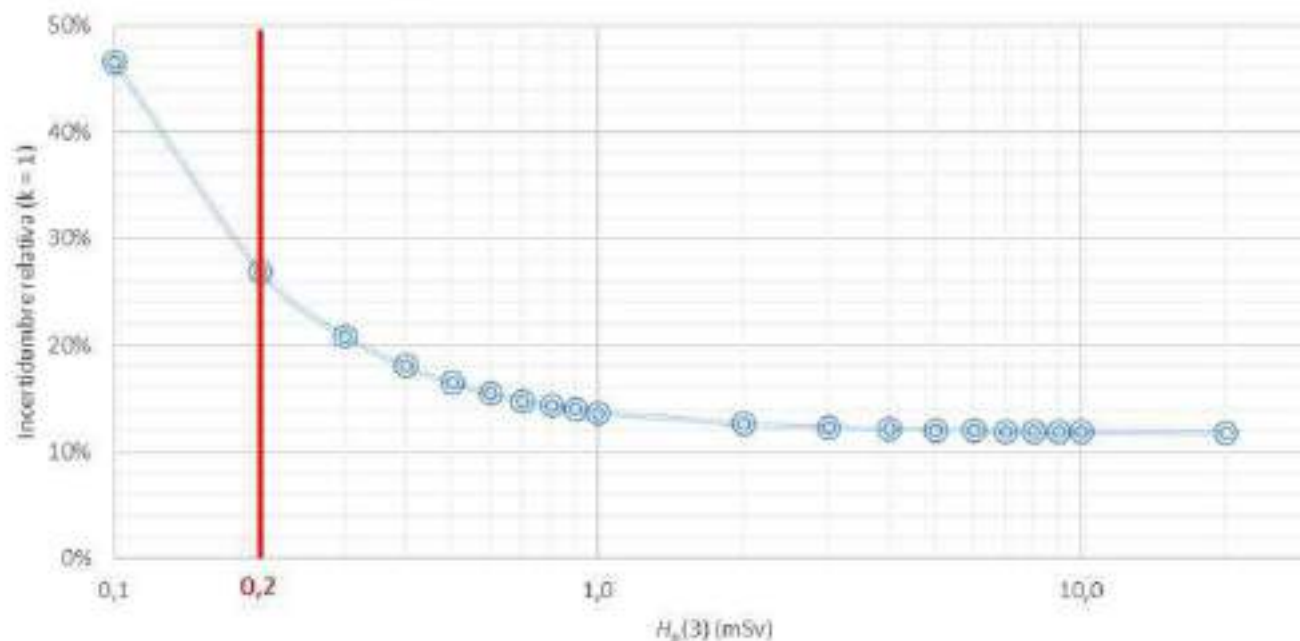
Incetidumbre típica combinada en función de la dosis neta asignada en cristalino
