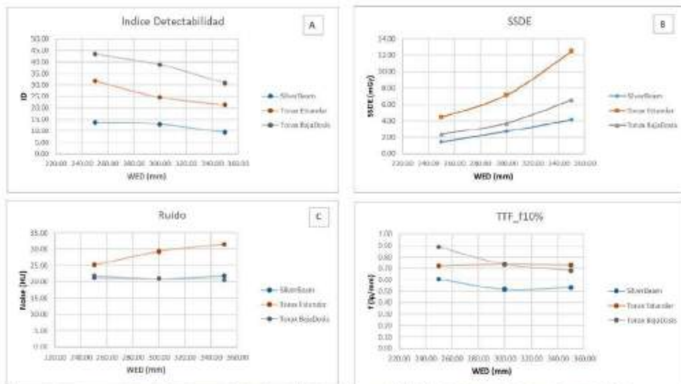
Figura 1. Representación gráfica de resultados de a) Índice de Detectabilidad, b) SSDE, c) Ruido y d) TTF al 10%
