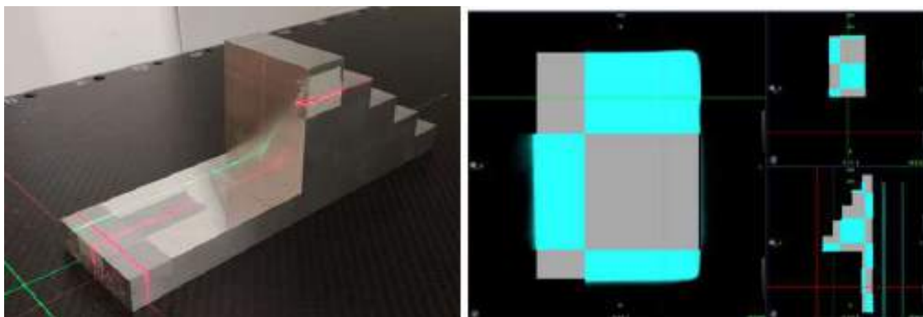
FIGURA 1: Maniquí en forma de cuña alineado con los láseres rojos (izquierda) y procedimiento de coincidencia entre la imagen realizada y la de referencia (derecha).
