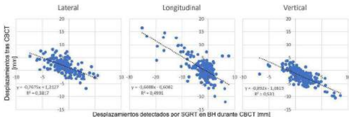
Figura 2: dispersión de posiciones calculadas por registro de superficies en BH de ETD durante el CBCT frente a desplazamientos realizados tras fusión.
