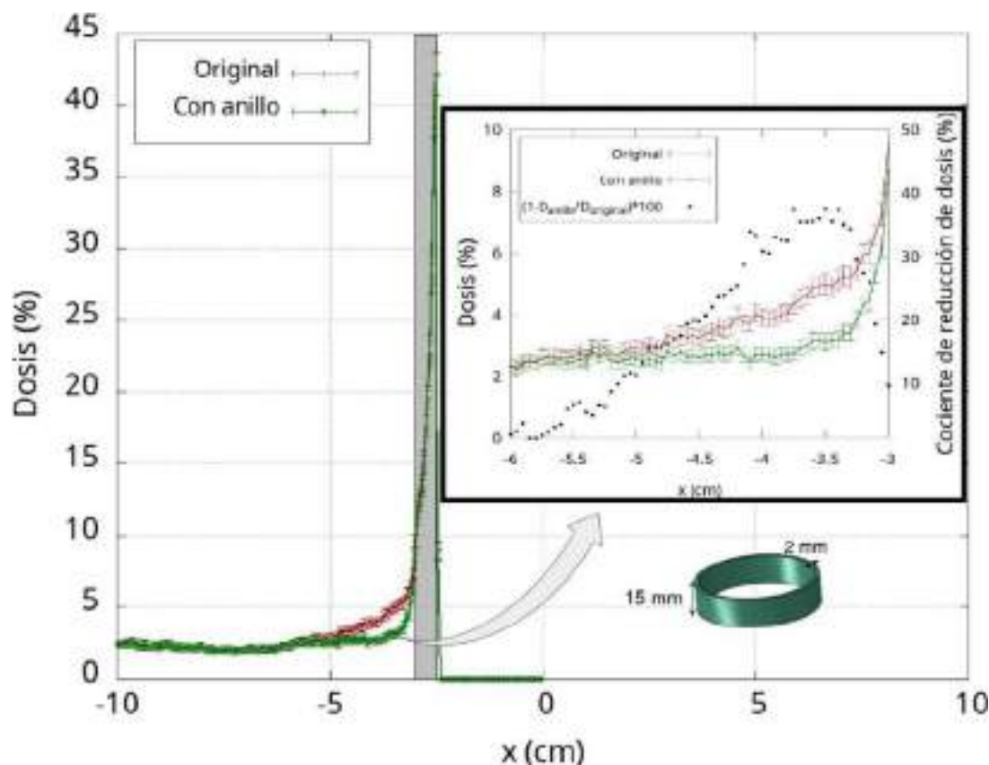
FIGURA 2: Semiperfil de dosis en superficie para la configuración original y con anillo de Pb y variación de dosis (haz de 12 MeV). Las barras de error corresponden a 2 y la zona sombreada a la pared del aplicador.
