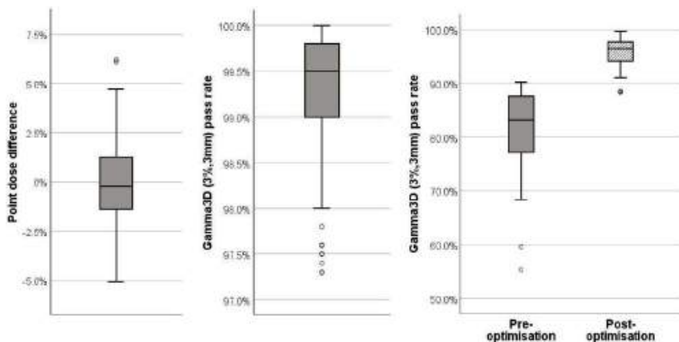
FIGURA 1: DD (izquierda) y %-paso gamma (centro) arrojadas por Mobius3D en planes Ethos. A la derecha, %-paso gamma pre y post-optimización para planes TrueBeam IMRT. Las cajas representan (Q3-Q1), y las líneas centrales, las medianas. Las colas indican los rangos, con outliers ( =\text{cuartil} \pm 1.5 \times [\text{Q3}-\text{Q1}] ) simbolizados como círculos.
