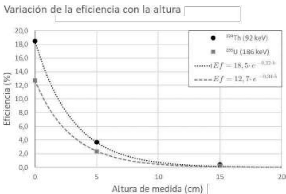
FIGURA 2. Eficiencia para los fotopicos de 92 keV del ^{234}\text{Th} y de 186 keV del ^{235}\text{U} .
