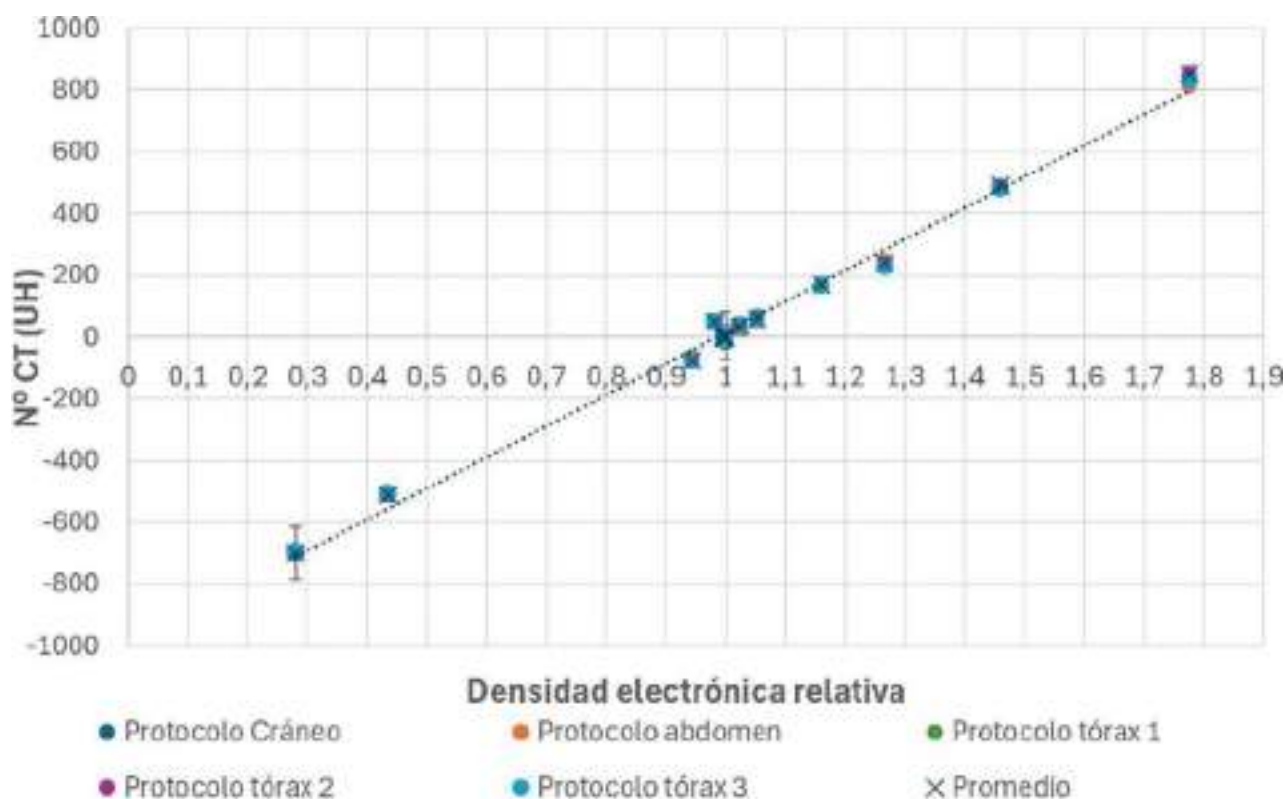
Gráfica 1: número CT medido frente a la densidad relativa. Valores y recta promedio.
