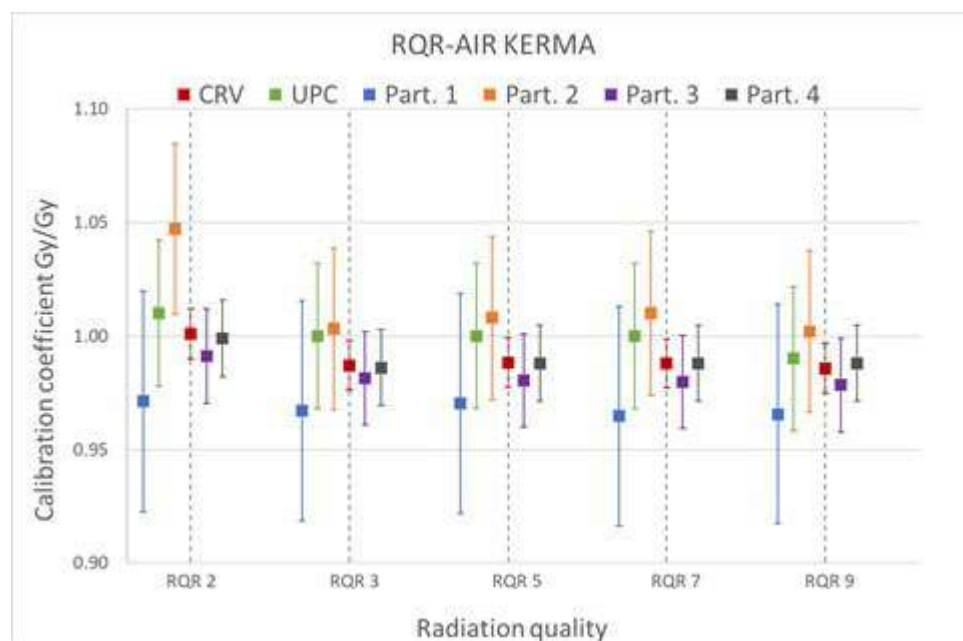
Figura: Valor de referencia (CRV) y factores de calibración, junto con su incertidumbre ( k = 2 ), obtenidos por los distintos participantes para el kerma en aire en las calidades RQR.
