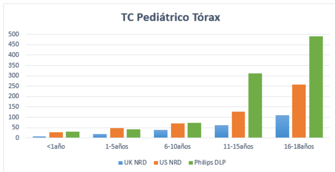
Figura 1. Gráfica tc tórax pediátrico
