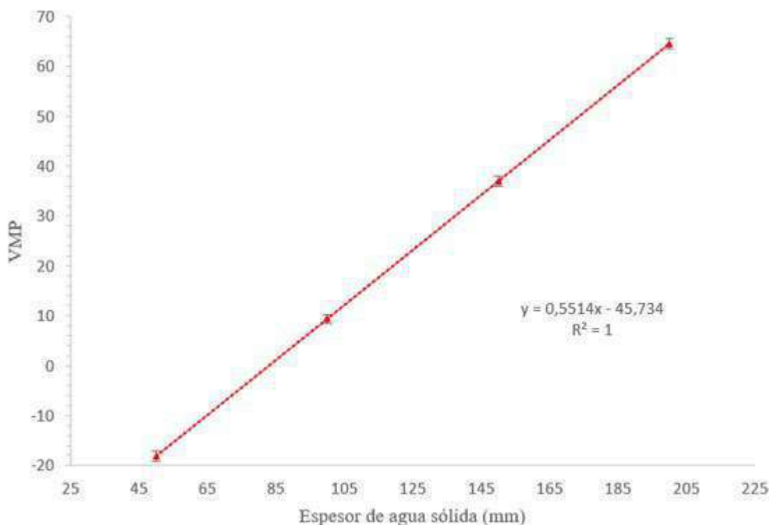
Figura 1. Relación entre espesor de agua sólida y valor medio del píxel
