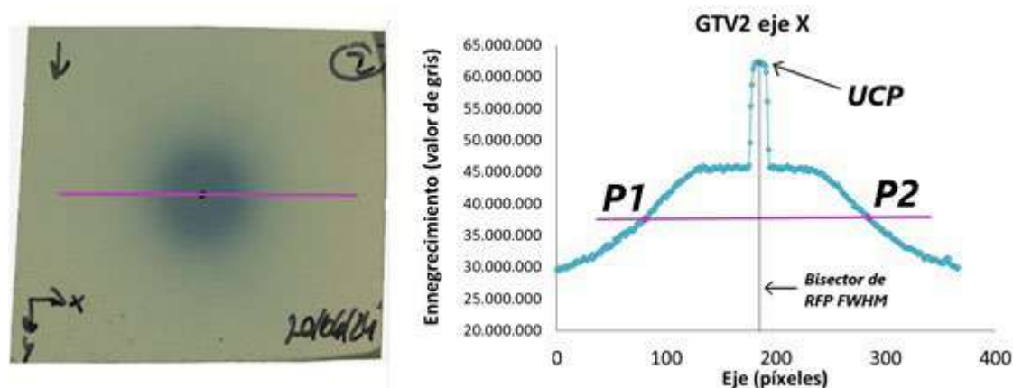
Figura: Ejemplo del método del TG 178 para obtener UCP y RFP a partir de una película radiocrómica irradiada.
