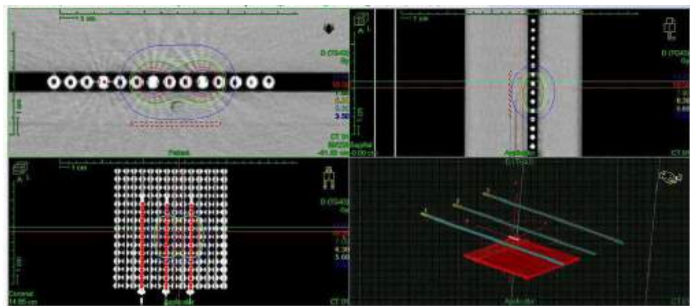
Figura 1. Montaje experimental del método 1. Consiste en un bloque de 5 cm de PMMA, película radiocrómica (línea discontinua roja), bloque de 2 cm de PMMA con inserto para la cámara PinPoint (la cual se contornea su volumen sensible en rosa), aplicadores Freiburg y bloque de 5 cm de PMMA. Se puede apreciar la distribución de dosis y las posiciones de parada activadas así como el montaje de las agujas, película y volumen sensible de cámara en 3D. Además, se miden dosis de forma puntual en cada volumen para posteriormente compararlos con los resultados experimentales.
