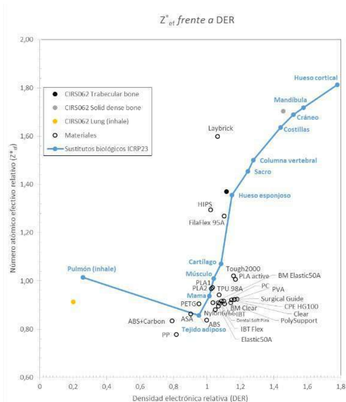
Figura 1.- Plano número atómico efectivo frente a DER de los materiales, sustitutos biológicos (ICRP 23) e insertos CIRS 062.
