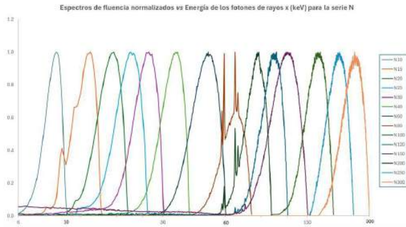
FIGURA 1. Espectros característicos de las calidades N caracterizados por el Laboratorio Nacional de Metrología de Radiaciones Ionizantes del CIEMAT
