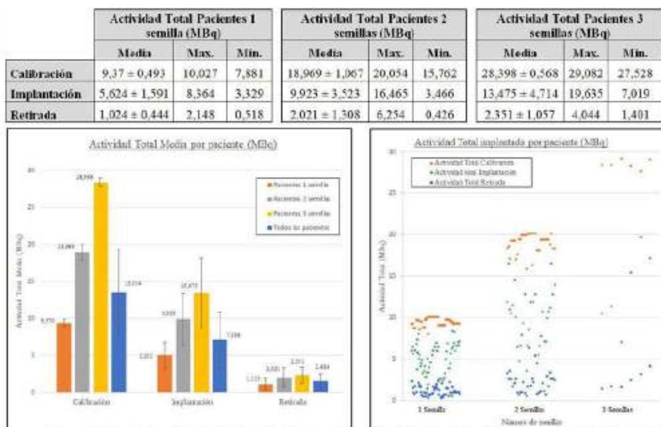
Figura 1: Caracterización de la Actividad Total por paciente en la calibración, la implantación y la retirada de las semillas.
