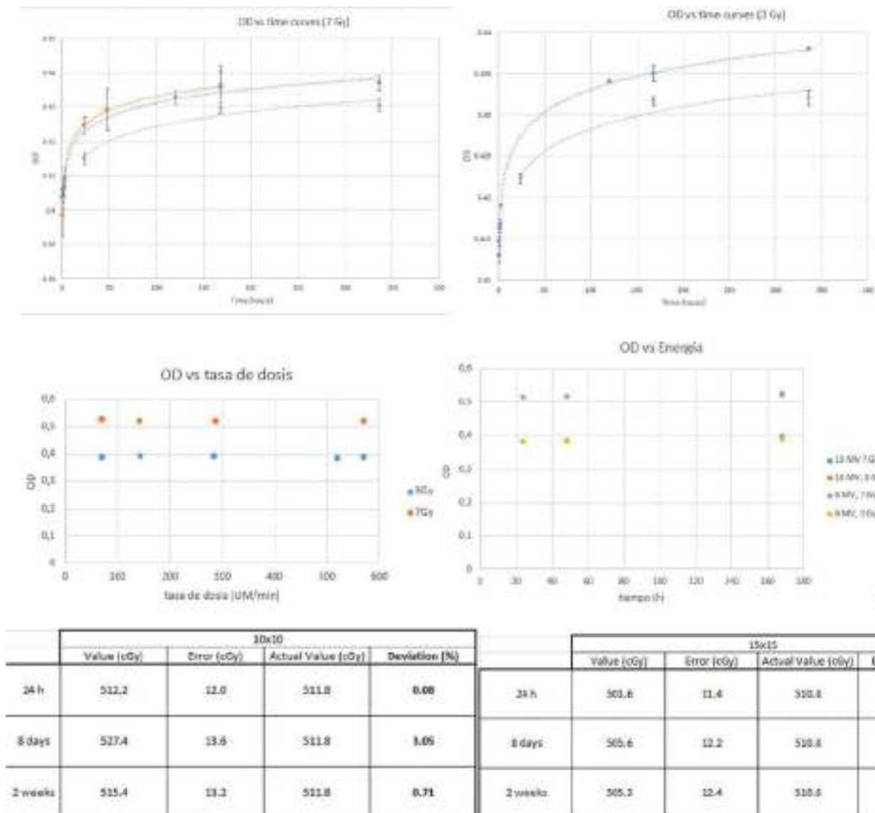
FIGURA 2: Evolución OD respecto al tiempo, la energía y la tasa de dosis (arriba). Precisión en dosimetría absoluta frente al estudio multicentro (abajo).
