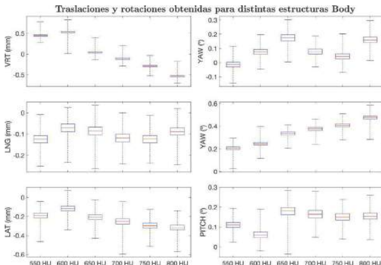
FIGURA 1: Variación de las traslaciones y rotaciones detectadas por AlignRT para las seis superficies generadas. Se muestra en rojo la mediana, en azul el primer y tercer cuartil, y en negro los valores máximo y mínimo obtenidos. En el eje x se muestran los distintos valores umbrales utilizados para generar las distintas estructuras.
