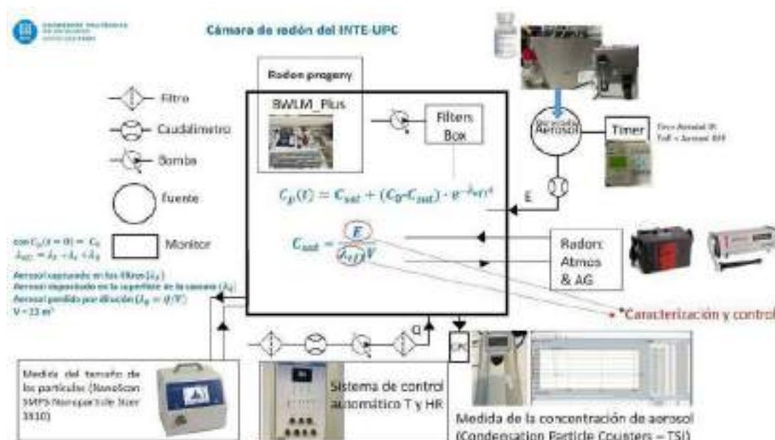
FIGURA 1. Esquema de la configuración actual de la cámara de radón tipo 'walking-in' de la UPC.
