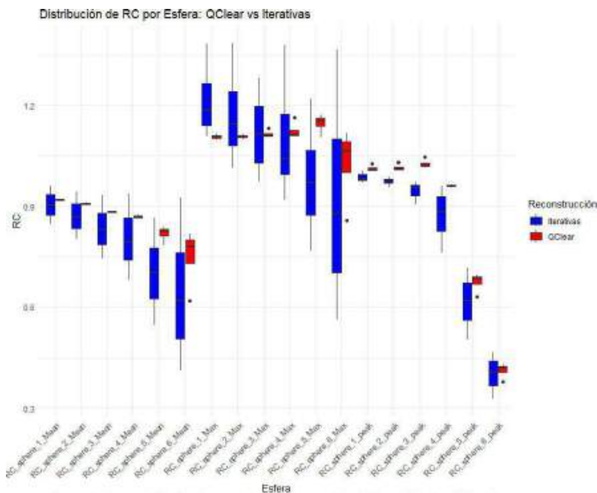
Imagen 2. Comparativa tipo de reconstrucción para cada métrica y diámetro de la esfera (Esfera 1: 37mm; Esfera 2: 28; Esfera 3: 22mm; Esfera 4: 17mm; Esfera 5: 13mm; Esfera 6: 10 mm)
