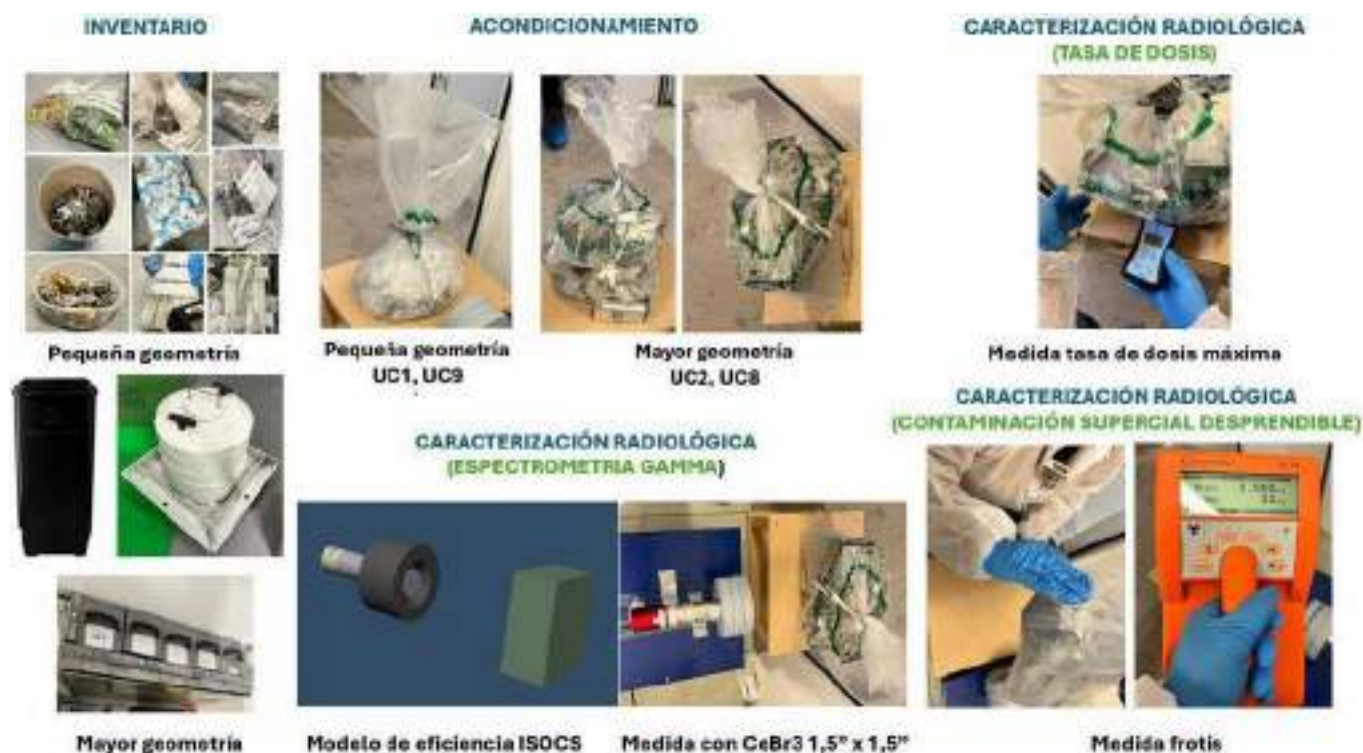
FIGURA 1.- Gestión de los residuos (acondicionamiento, caracterización radiológica: tasa de dosis, CSD y espectrometría gamma)
