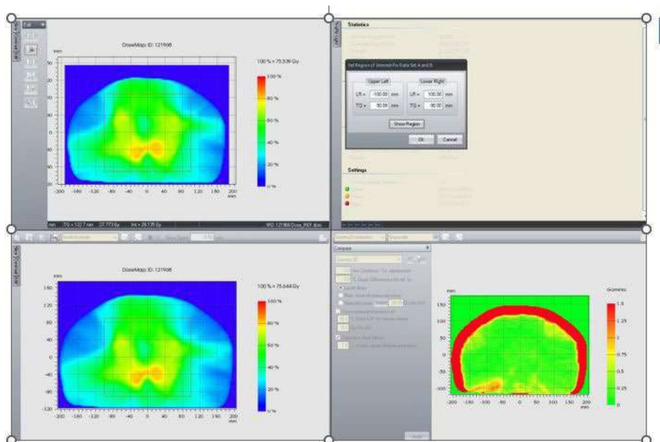
Figura 2: Región de interés en el plano transversal para realizar la evaluación del índice gamma 3D.
