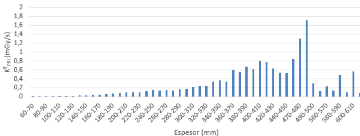
FIGURA 1. Tasa de kerma en punto de referencia intervencionista, \dot{K}_{PRI} , frente espesor equivalente de paciente para todos los eventos de irradiación.
