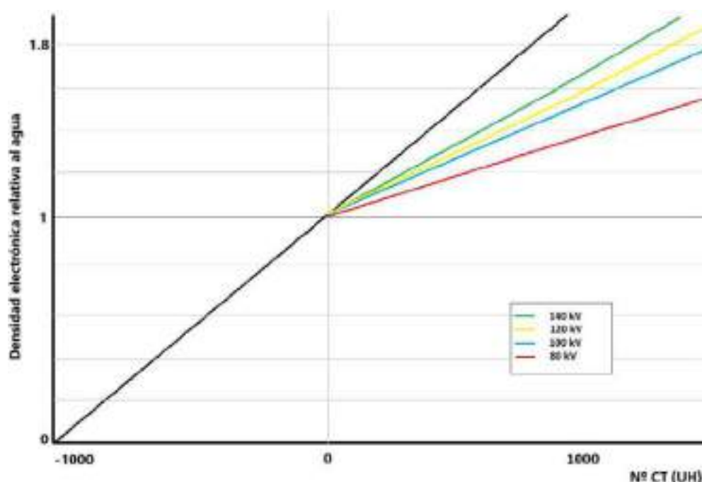
Imagen 1: curva de calibración DirectDensity vs curvas de calibración convencionales dependientes del voltaje.
