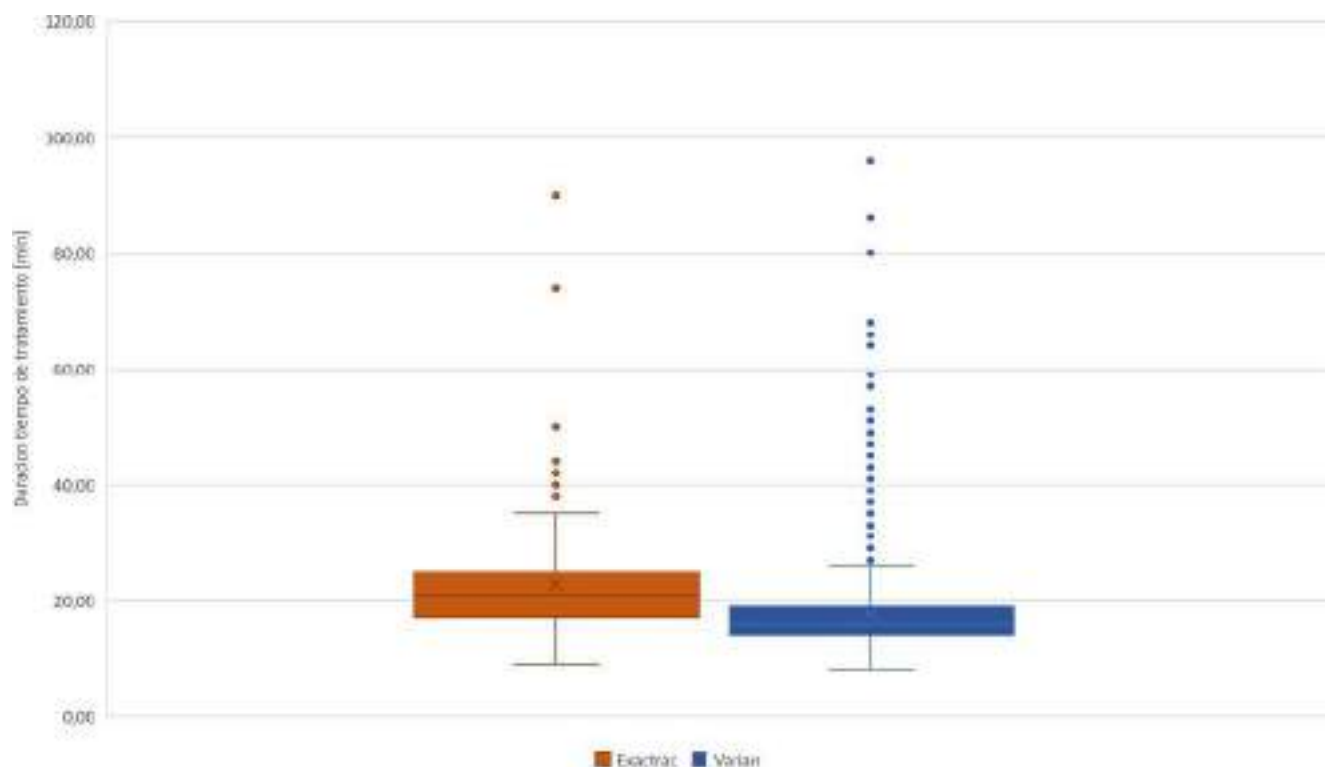
Figura 2: Duración de los tiempos de tratamiento de pacientes en formato de cajas y bigotes. Varian es el sistema RGSC de Varian y Exactrac es el sistema Exactrac Dynamic (Brainlab).
