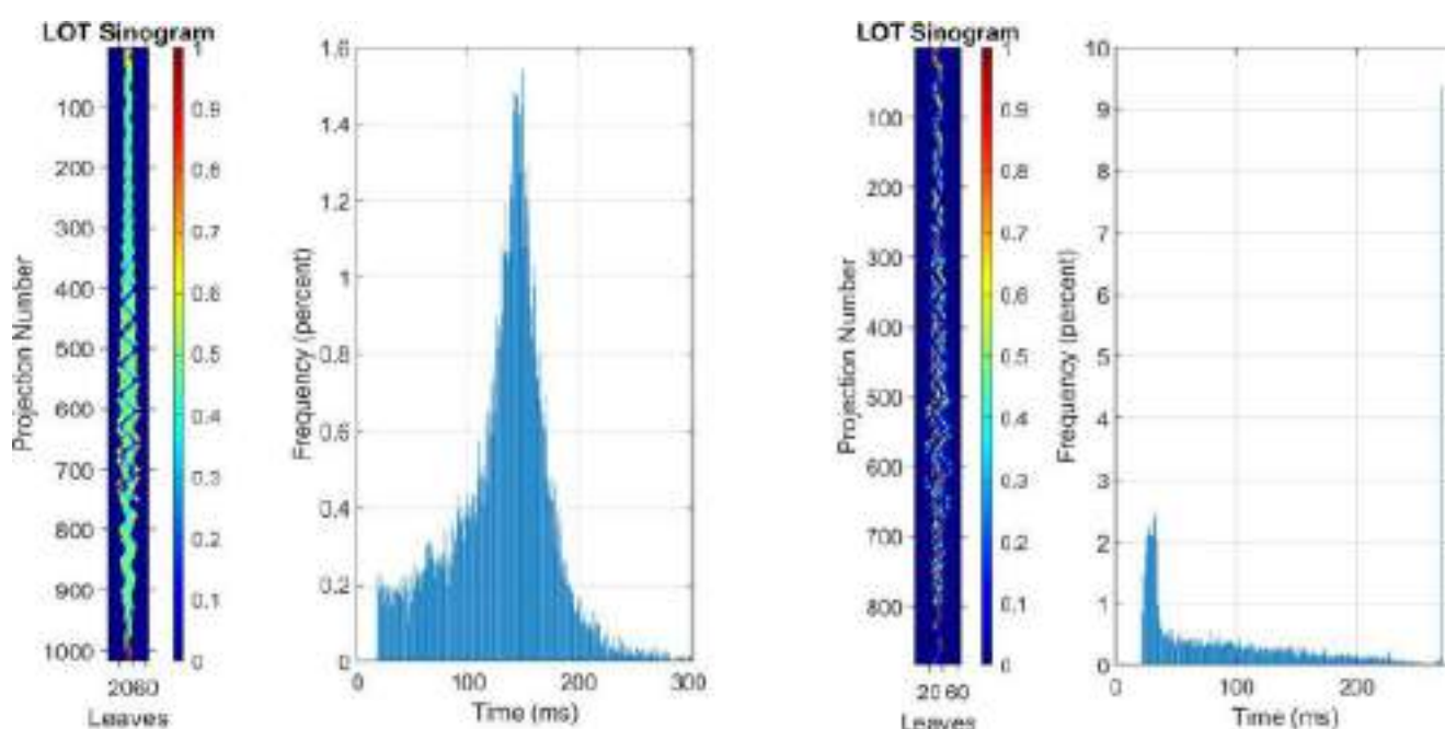
FIGURA 2: Sinograma e histograma del porcentaje de tiempo de apertura de las láminas (LOT) de planes de tratamiento típicos de Precision (izquierda) y RayStation (derecha).
