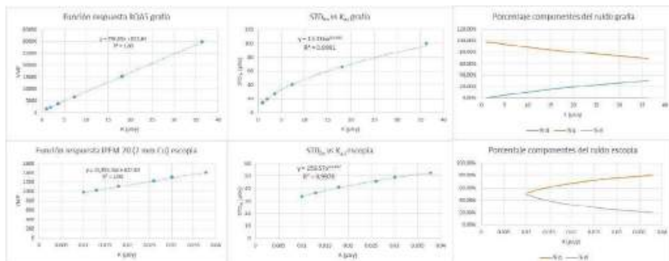
FIGURA 1. Funciones respuesta y análisis del ruido en modo gráfia y en modo escopía.
