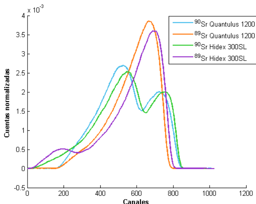
FIGURA 1. Espectros normalizados de ^{90}\text{Sr} en equilibrio con ^{90}\text{Y} y de ^{89}\text{Sr} para 1220 Quantulus TM y Hidex 300 SL.
