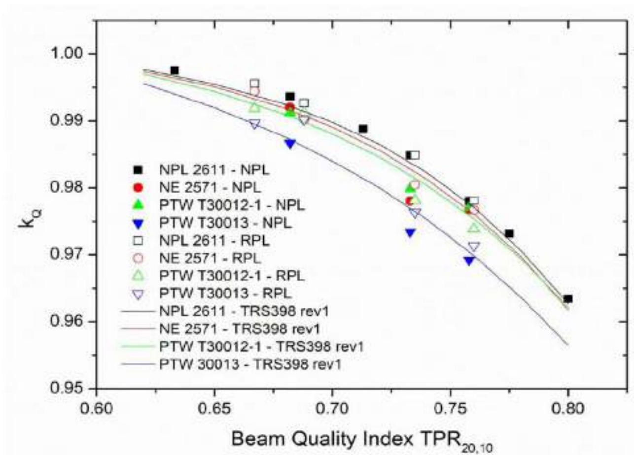
FIGURA 2 Factores correctores de calidad de haz como función del TPR 2010 medido en el NPL y en el RPL Discusión
