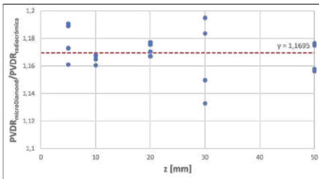
Figura 2. Relación entre PVDR a distintas profundidades para microDiamond (resolución 1 \mu\text{m} ) y radiocrómica (resolución 600 dpi = 40 \mu\text{m} ).
