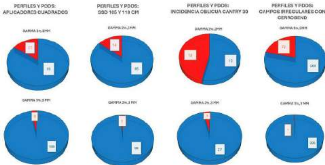
Fig. 2: Número total de medidas de perfiles (inplane, crossplane y diagonales) y PDDs comparadas con el TPS, clasificadas según las pruebas realizadas y el criterio de paso gamma aplicado. En azul o rojo si cumplen o no el criterio respectivamente.
