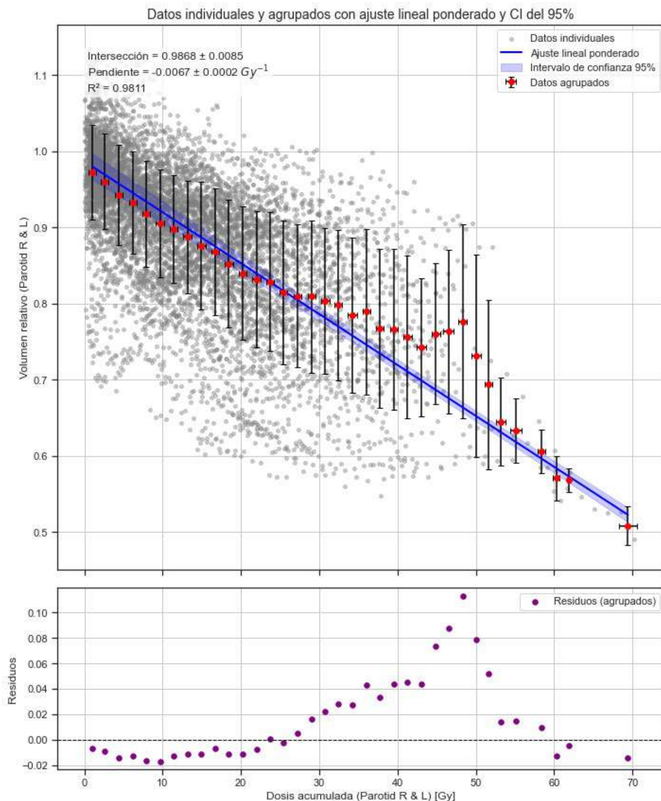
FIGURA 2: Dosis media acumulada relativa frente al desplazamiento relativo del CM para las GP. El análisis de residuos no mostró desviaciones sistemáticas significativas.
