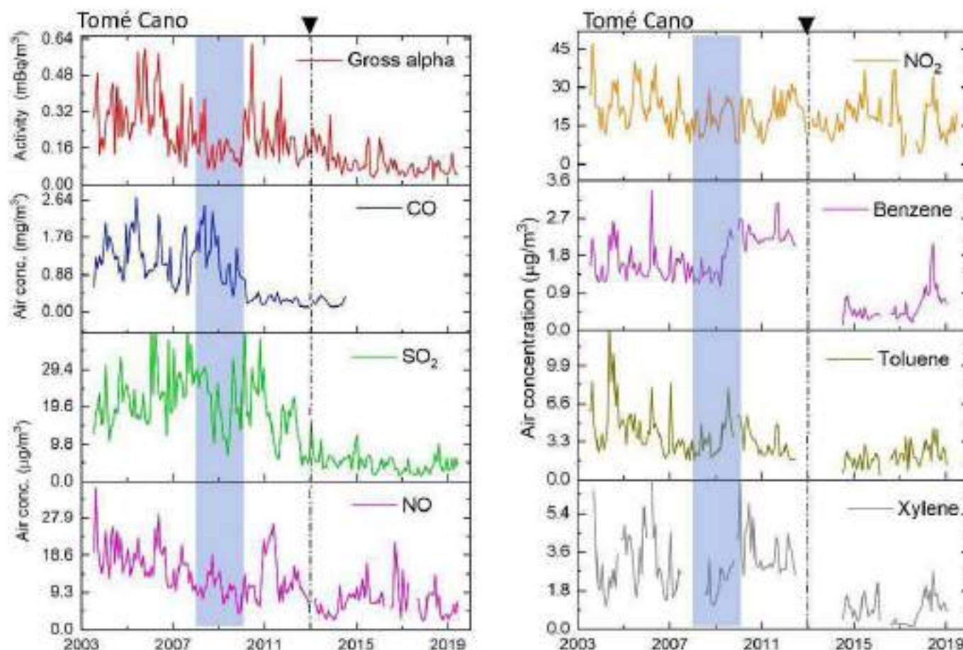
FIG. 2. Variaciones mensuales de actividad alfa total y contaminantes antropogénicos. Triángulo marca el año 2013, cuando la refinería cesó su actividad. La línea de contorno azul indica el período atribuido a la crisis económica global de 2008.
