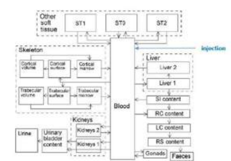
Figura 1.- Modelo biocinético de los lantánidos
