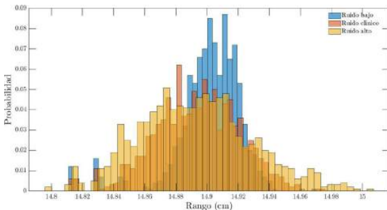
FIGURA 2: Distribución de probabilidad del rango (cm) en cerebro para valores de ruido clínicos (naranja), bajo (azul) y alto (amarillo).
