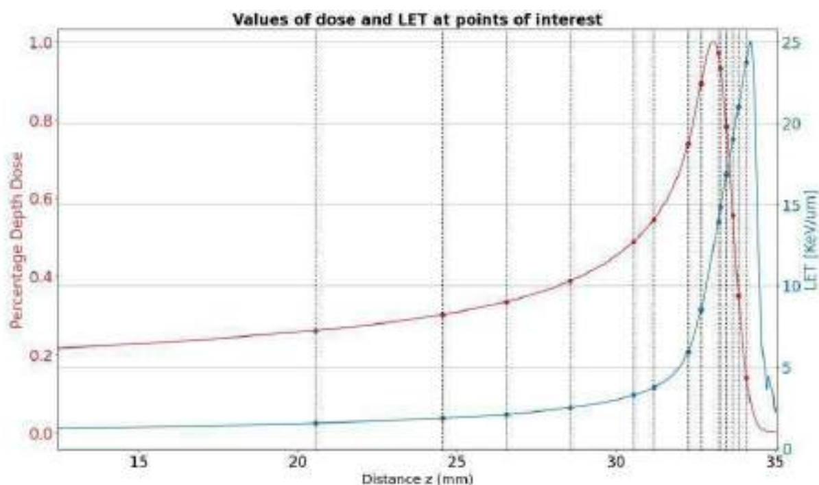
Figura 1. Simulación MC con Gamos/Geant4 para un haz de protones de 70.2 MeV del sistema ProBeat-CR en la CUN y material PMMA. La curva roja representa el PDD, mientras que la curva azul representa los valores de LETd considerando exclusivamente protones primarios.
