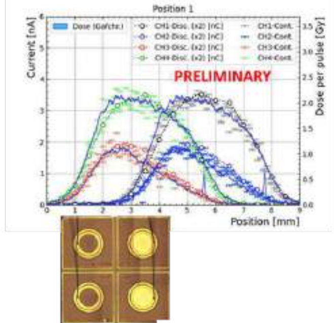
Figura 1. Izquierda: Linealidad de la sensibilidad demostrada por un diodo de SiC producido en el IMB-CNM probado con pulsos de electrones de 6 MeV [3]. Derecha: Perfil de un haz de protones no-homogéneo de 7 MeV obtenido con una matriz de 2x2 píxeles.
