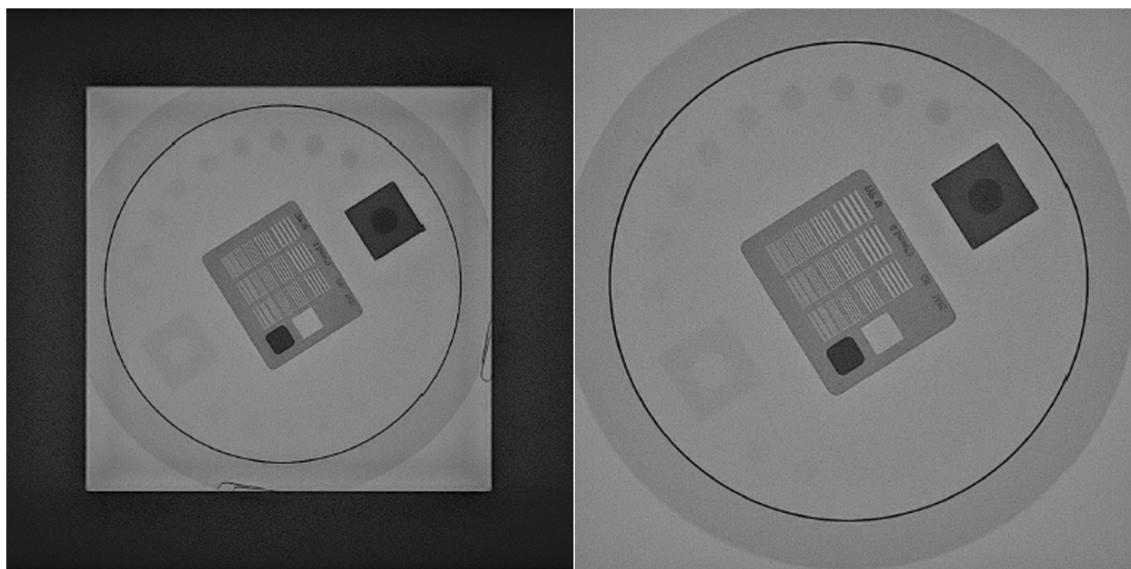
Figura 1. Imagen del maniquí TOR 18FG con la lupa de 42 cm y colimación manual a 37 cm (izquierda) y con la lupa de 37 cm sin colimación manual (derecha).
