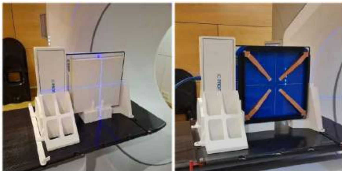
Figura 1: Dispositivo experimental para medidas con build-up de agua sólida (izquierda) y en superficie, con cuñas de cobre (derecha).
