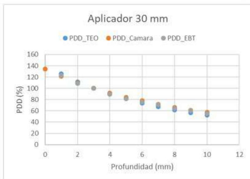
FIGURA 1. En el grafico superior se muestra como se obtiene el perfil plano en la posición 1121 mm. En el gráfico inferior se muestra la comparación de los porcentajes de dosis en profundidad (PDD) determinados experimentalmente frente al modelo para el tamaño de aplicador de 30 mm.
