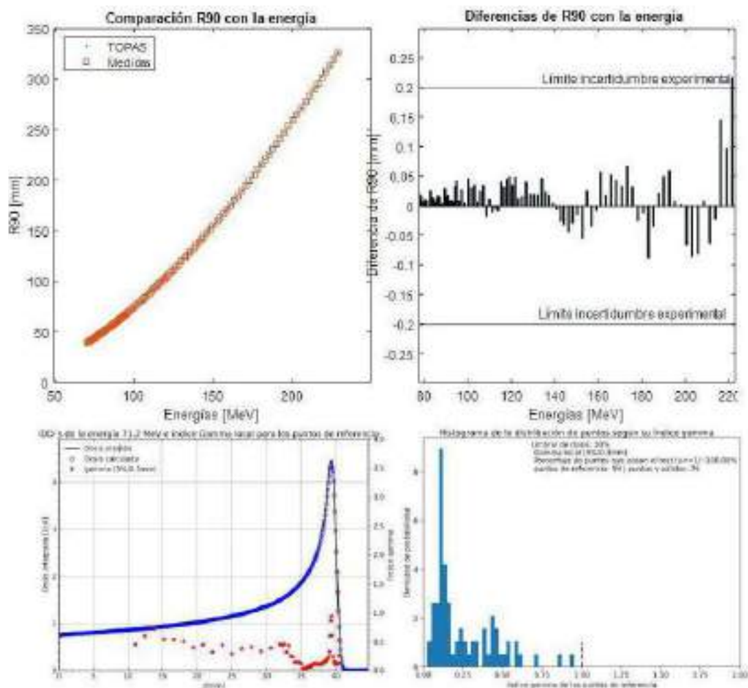
Fig1: (Arriba) Comparación de parámetros R90 en función de la energía. (Abajo) Ejemplo de test gamma para la energía de 71.2 MeV
