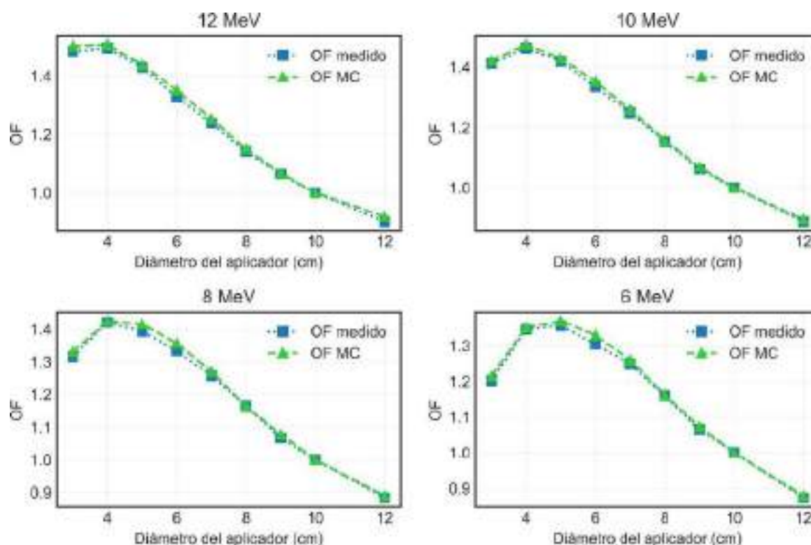
FIG. 2 Comparación de factores de salida (OF) determinados experimentalmente y calculados por Monte Carlo para aplicadores no biselados.
