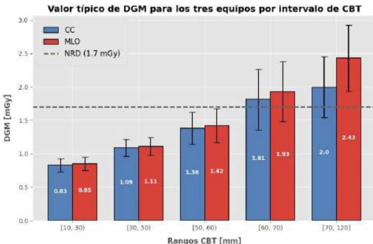
FIGURA 2. DGM típico para cada proyección en los tres equipos por intervalos de CBT.
