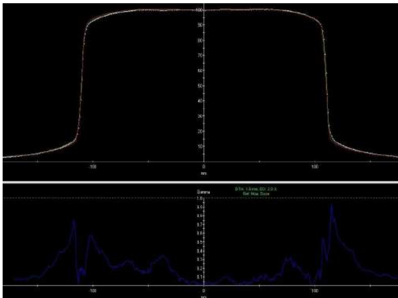
Imagen2: Comparación gamma 2% 1mm de perfiles X a profundidad 10cm de un campo 20x15cm 2 entre un campo calculado en Eclipse y otro medido en cuba de agua.
