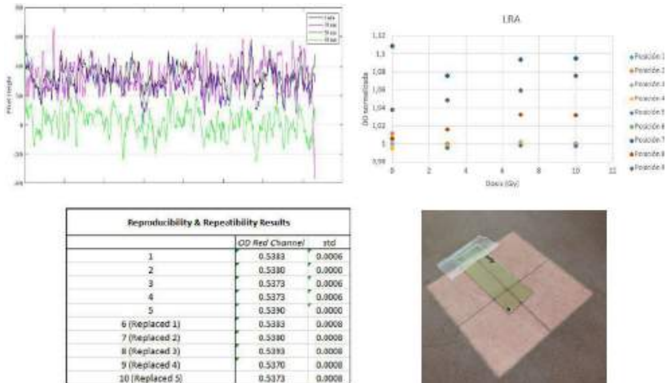
FIGURA 1: Warm up, LRA (arriba). Repetibilidad y set up (abajo).
