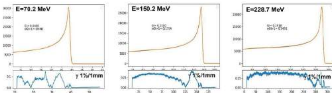
Fig. 2. Perfiles en profundidad en agua
