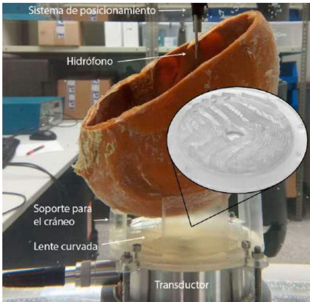
FIGURA 1: Montaje experimental para validación de la lente holográfica.
