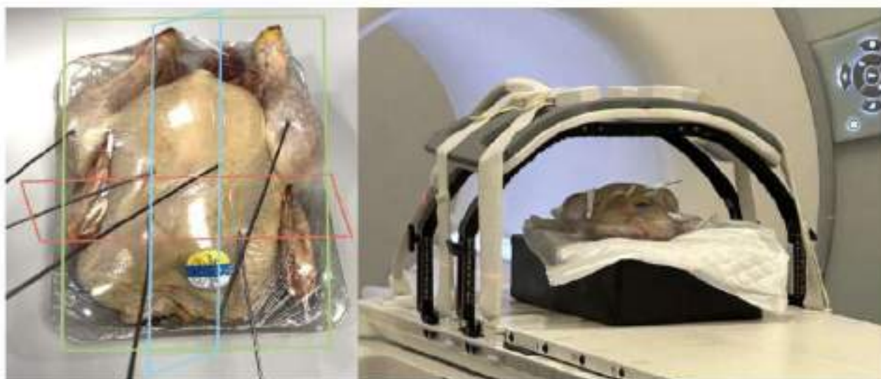
Figura 1. Izquierda: agujas insertadas en diferentes direcciones: eje axial (rojo), sagital (azul) y coronal (verde). Derecha: montaje para el estudio de RM.
