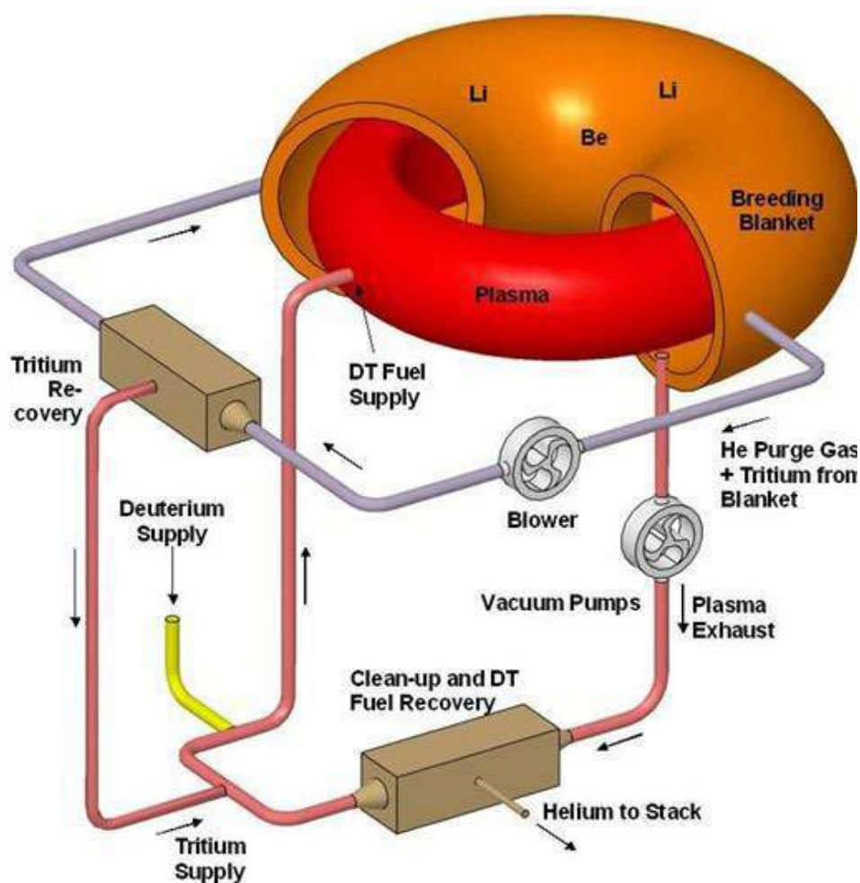
FIGURA 1.- Esquema del lazo cerrado del combustible de ITER [1].
