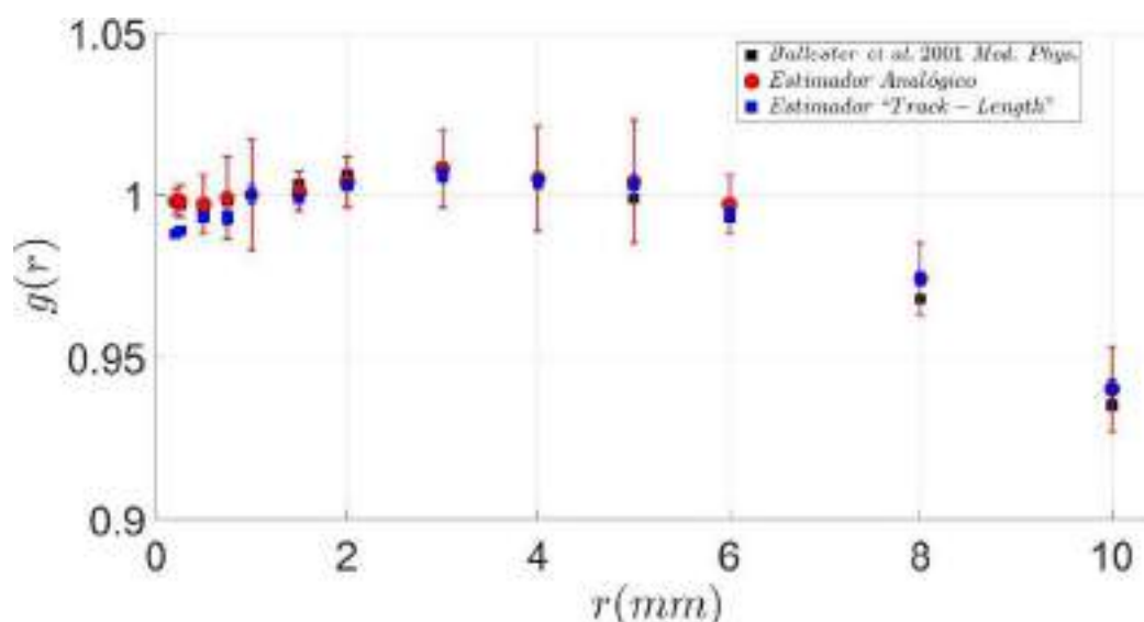
FIGURA 1: Valores de referencia de la función radial g(r) (cuadrados negros), de la fuente Ir-192 GammaMed Plus, frente a los calculados con el estimador analógico (círculos rojos) y el estimador “track-length” (cuadrados azules).
