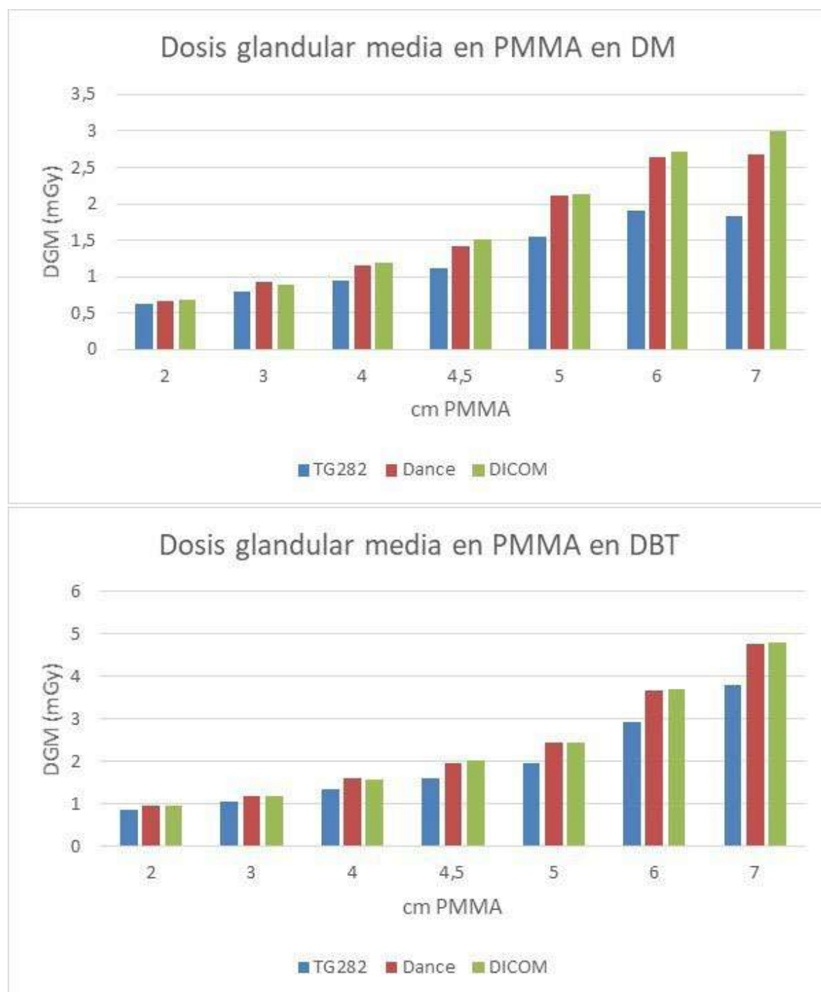
FIGURA 1. Dosis glandular media para diferentes espesores de PMMA
