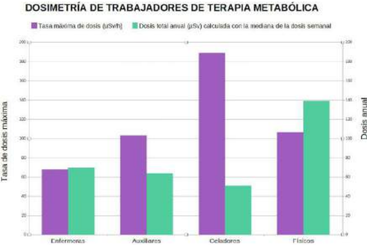
Gráfica 1. Tasas máximas y estimación de dosis total anual de los trabajadores.
