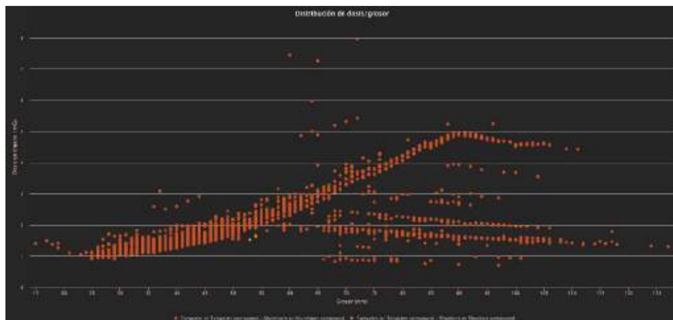
FIGURA 1: DGM (en y) frente grosor de la mama (en x). Imagen extraída de Qaelum.
