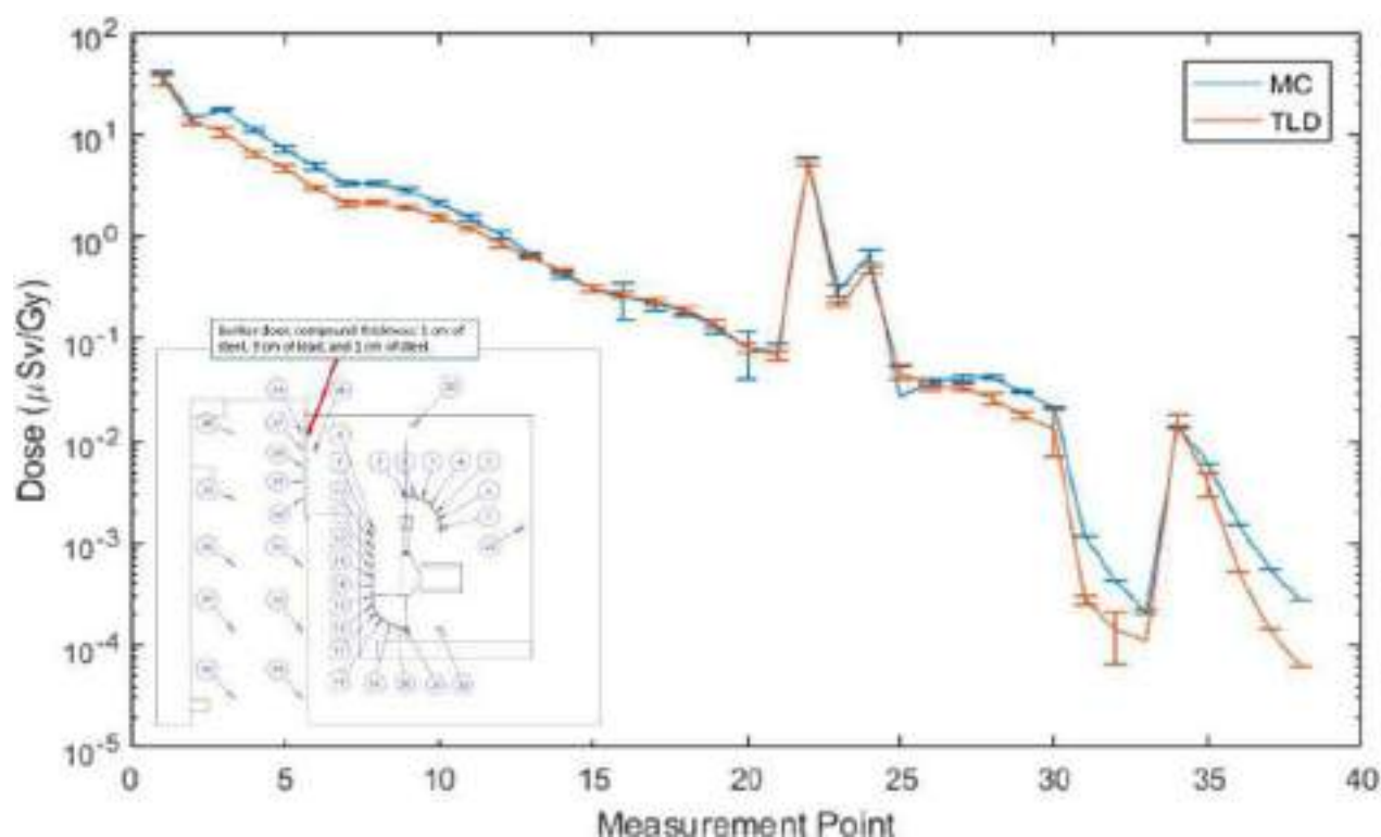
Figura-1. Tasa de dosis en el entorno del acelerador medidas y calculadas con GAMOS (MC).
