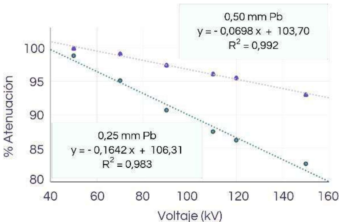
FIGURA 1: Porcentaje de atenuación para dos delantales de distintos espesores (0,25 mm y 0,5 mm) en función de diversos voltajes, con el correspondiente ajuste lineal.
