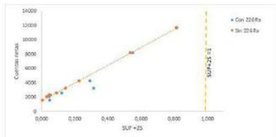
Figura 1. Cumplimiento de los NL ( \text{Bq}\cdot\text{g}^{-1} ) – criterio aceptación SUF +2S
