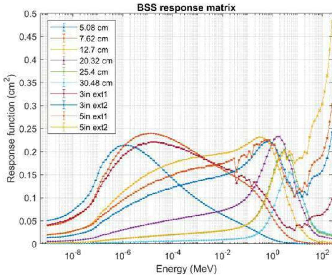
FIGURA 1: Matriz respuesta del EBSS. Respuesta en unidades de área respecto a la energía, en MeV, en escala logarítmica.
