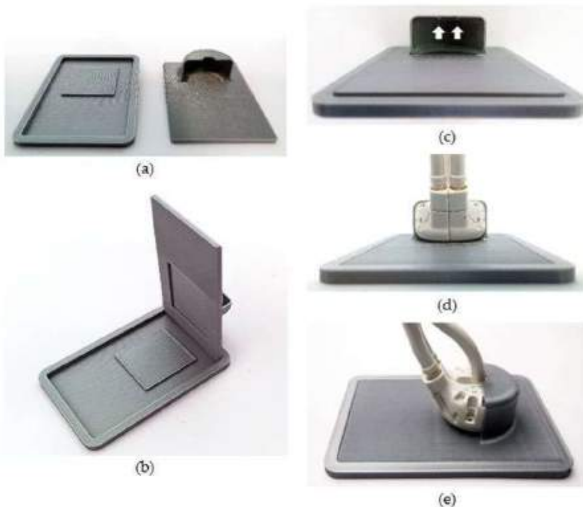
Figura 1: Fotos del soporte 3D para el aplicador Venezia™ con ovoides de 22 mm de diámetro. (a) y (b) muestran las dos piezas que lo componen, y el alojamiento para la película radiocrómica cuadrada. (c) Las flechas blancas indican los anclajes coincidentes con dos de los orificios del ovoide lunar de 22 mm. (d) y (e) muestran el aplicador en su alojamiento.
