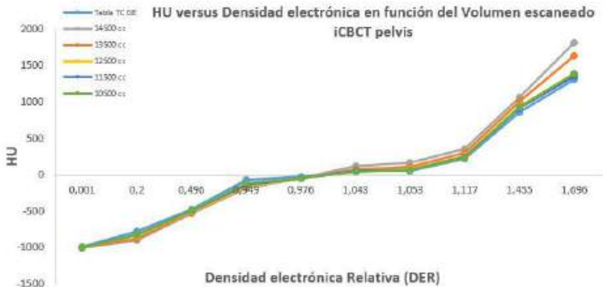
Figura1: Relación entre las Unidades Hounsfield (HU) y la densidad electrónica Relativa (DER) obtenidas para el protocolo de CBCT de "pelvis iterativo". Se escanea el maniquí CIRS de densidades envuelto en distintas capas de bolus de densidad equivalente a agua con el fin de variar el volumen escaneado. La curva azul "Tabla TC GE" corresponde a la tabla de calibración obtenida en el TC de planificación. La curva amarilla "12500 cc" corresponde al volumen escaneado equivalente al paciente estándar en los tratamientos de la patología de próstata.
