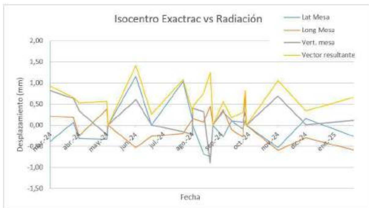
Fig. 2. Distancias entre el isocentro del RxETD y el isocentro de radiación en las tres direcciones del espacio y su vector resultante.
