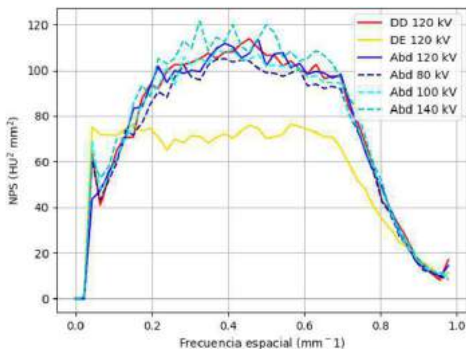
Figura 1. NPS de las imágenes de abdomen a diferentes kV y las imágenes DE y DD a 120 kV.
