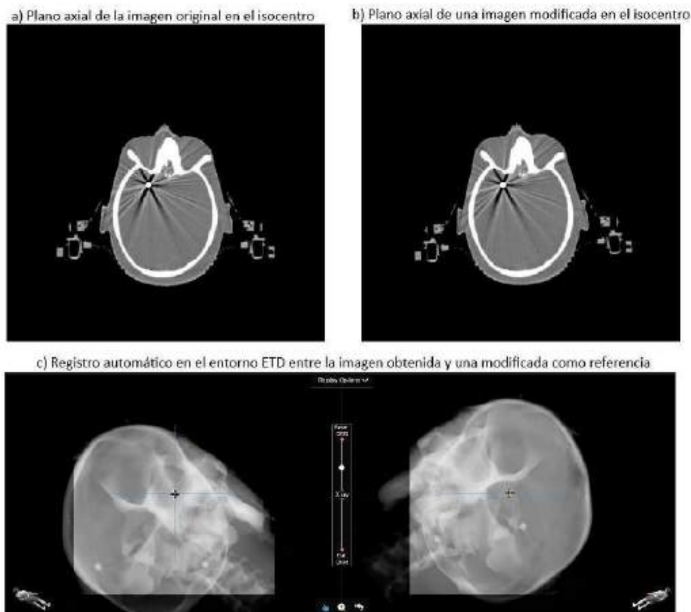
Figura 1. Ilustración del maniquí usado. a) Imagen TC original de un corte axial del maniquí en el isocentro. b) La misma imagen con una rotación aplicada digitalmente. c) Interfaz de ETD en el momento que aplica el registro automático entre las 2 imágenes de las proyecciones oblicuas de rayos X que adquiere, y la imagen que tiene de referencia.
