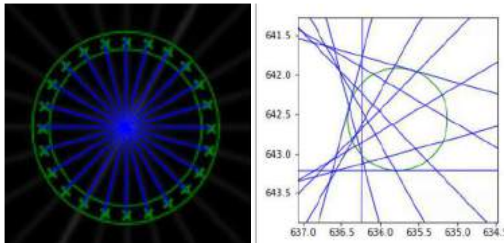
FIGURA 1. A) Líneas generadas al unir puntos contrapuestos de la región de análisis en la imagen “de estrella”. B) Zoom en la intersección de dichas líneas con el círculo de radio mínimo dibujado en verde.
