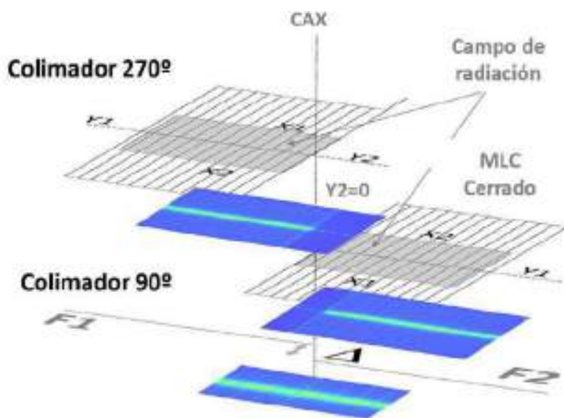
Figura 1. Esquema de irradiación del método propuesto.
