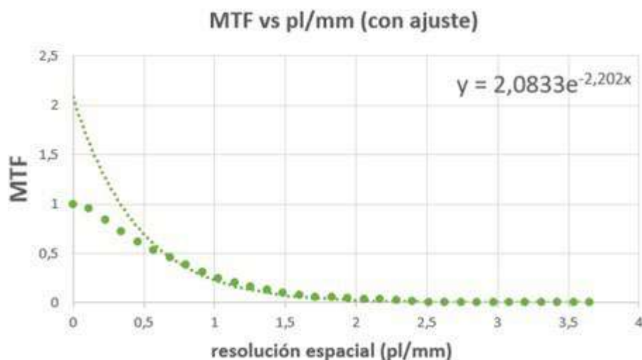
Figura 1: Representación gráfica de la MTF con ajuste exponencial
