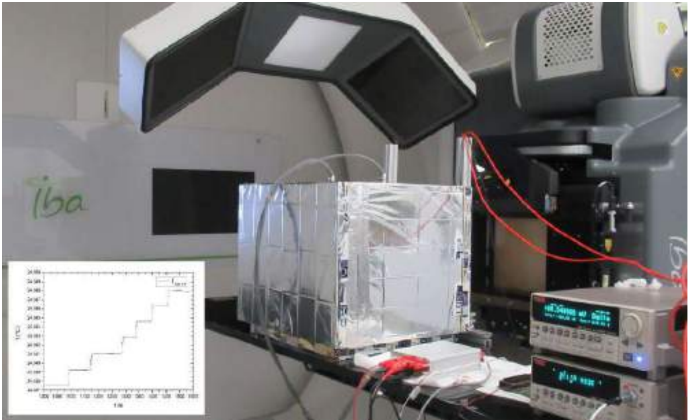
FIGURA 1: Montaje del calorímetro en una sala de protonterapia y ejemplo de medidas.
