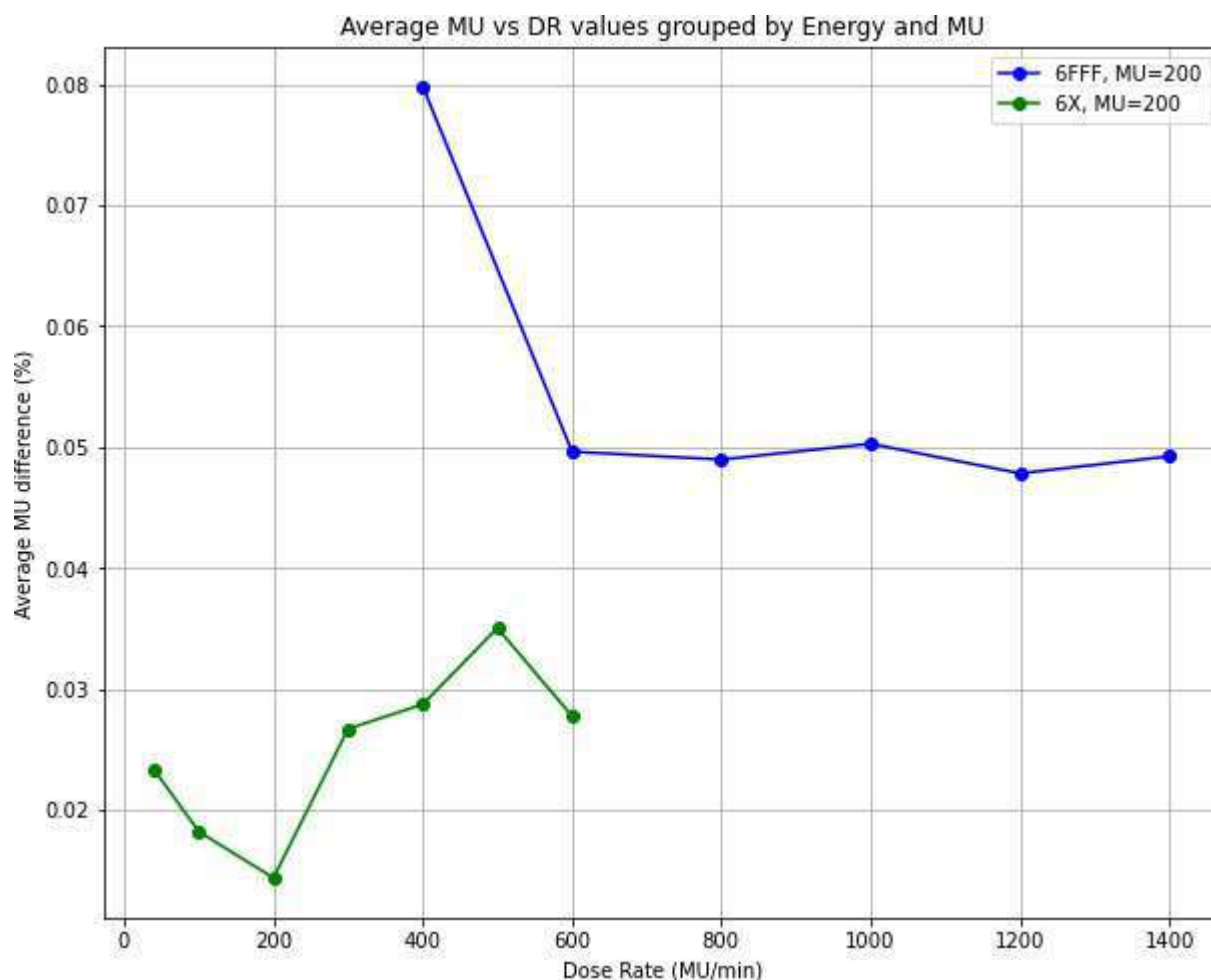
FIGURA 1. Diferencia entre unidades monitor impartidas y esperadas, para cada tasa de dosis y energía.
