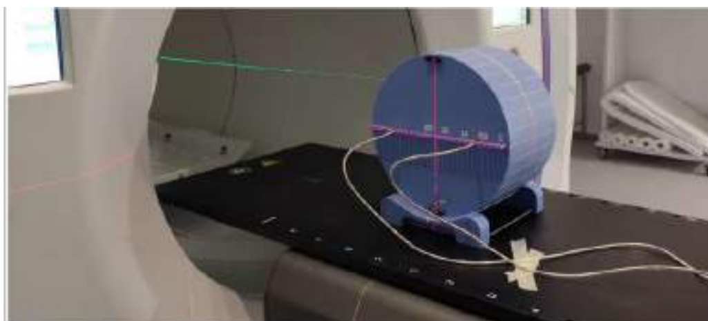
Figura 1: Montaje utilizado para la prueba siguiendo la referencia [2]
