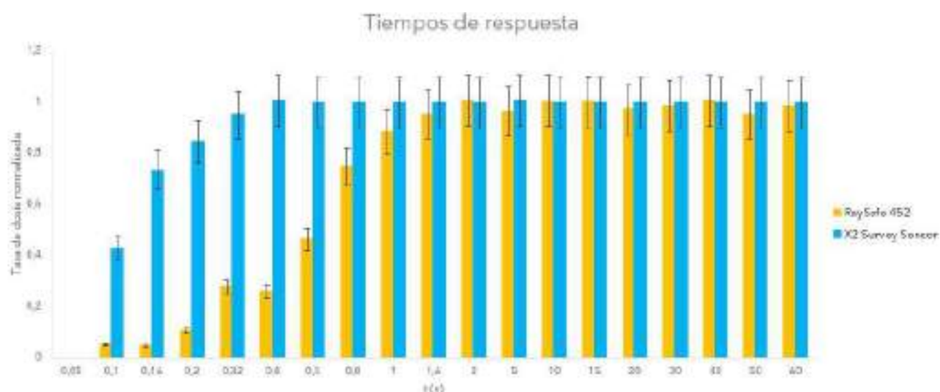
Fig. 1 Se muestran las tasas normalizadas medidas con ambos detectores para distintos tiempos de adquisición.
