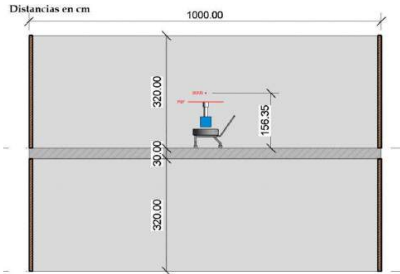
Figura 1: Montaje experimental, medidas de la sala, ubicación del origen y del espacio de fases (PSF).
