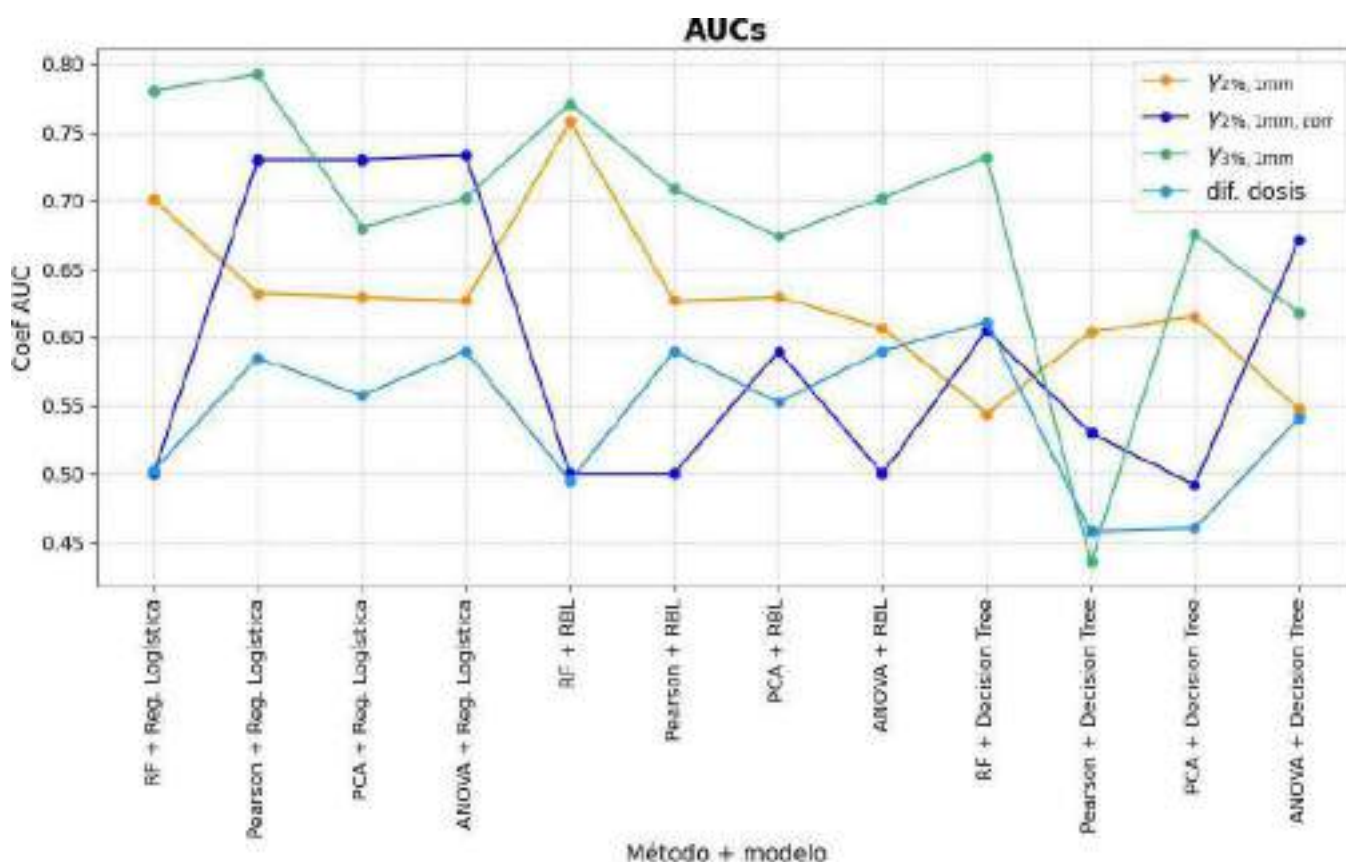
Figura 1. Comparación de AUC para cada métrica y modelo.
