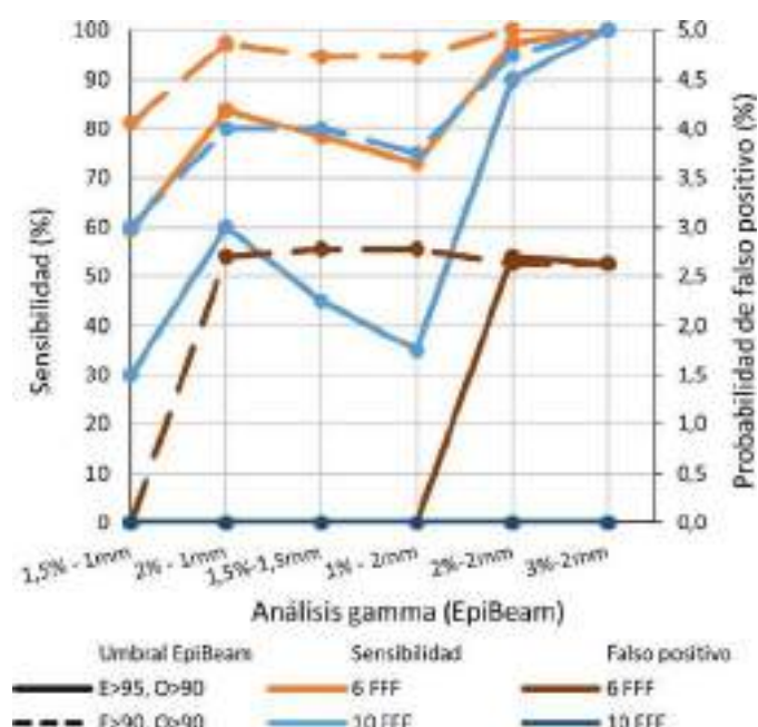
FIGURA 1. Sensibilidad y falsos positivos de la comparación de los análisis gamma con EpiBeam respecto a los resultados con Octavius 1500.
