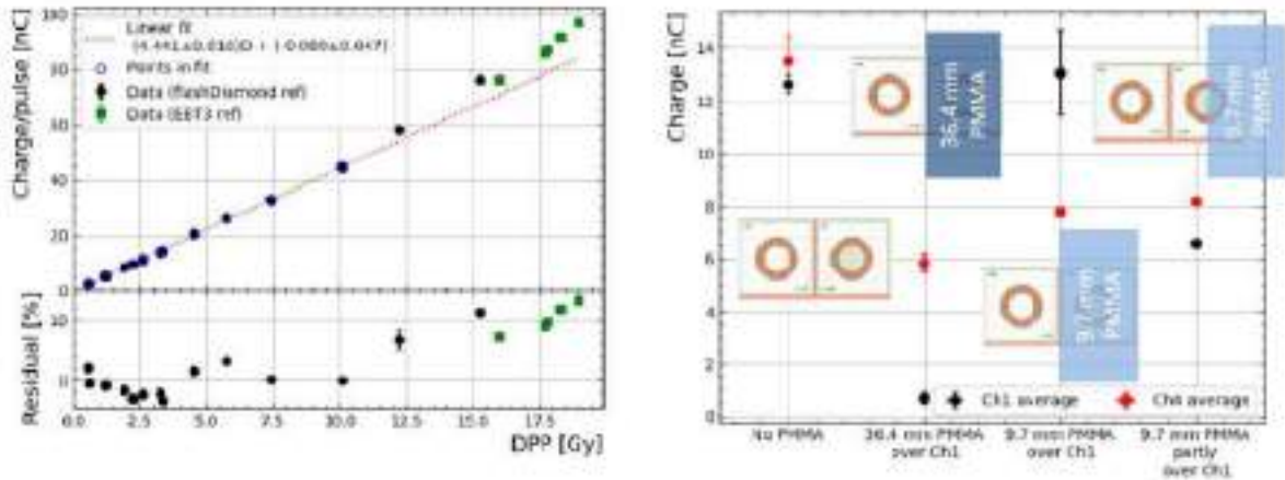
Figura 2. Izquierda: carga por pulso registrada en el SiC-2mm en función de la dosis por pulso. Derecha: carga colectada por el SiC-array en una de las configuraciones experimentales.
