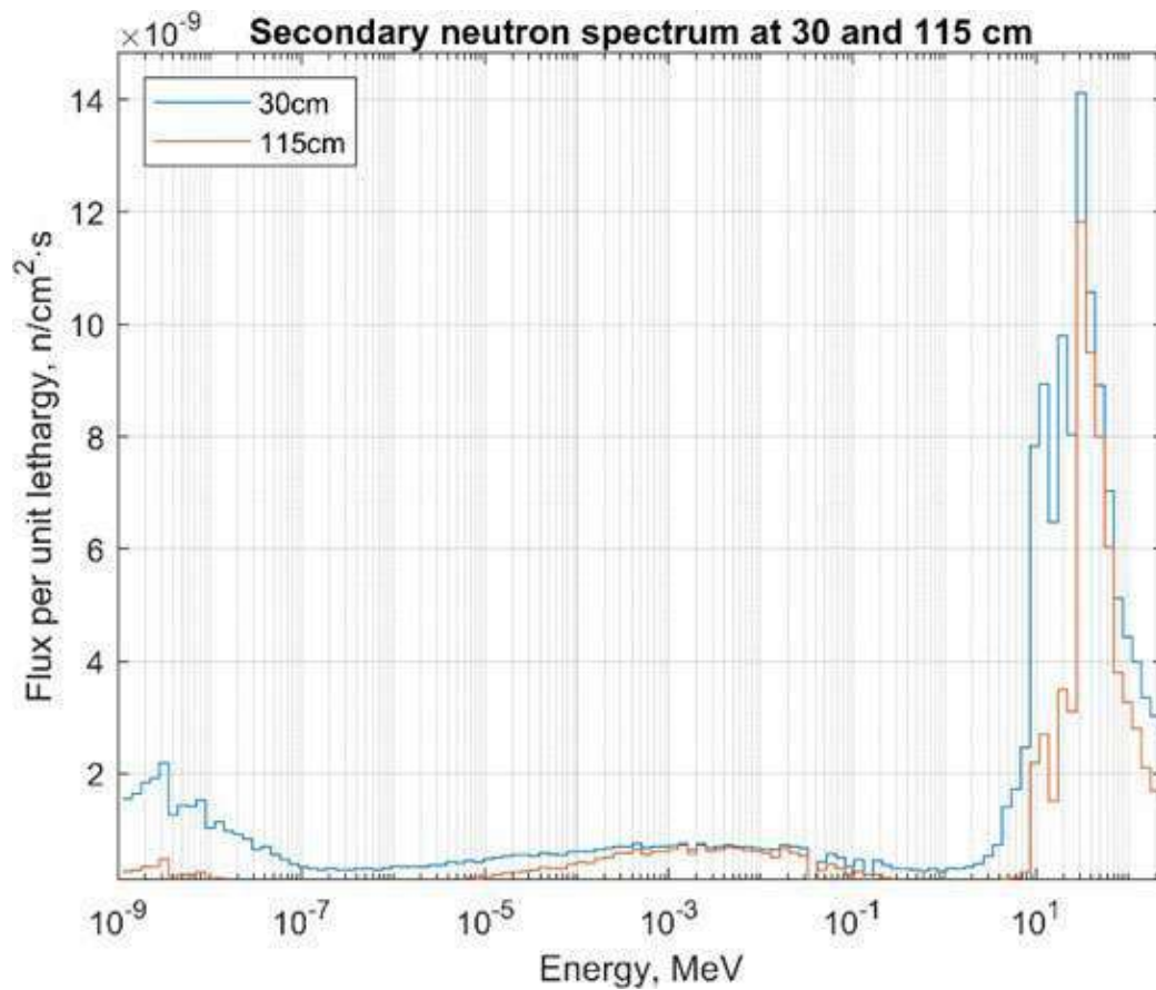
FIGURA 2: Espectro deconvolucionado utilizando el algoritmo MLEM para 30 y 115 cm de distancia de la salida del cabezal del acelerador.
