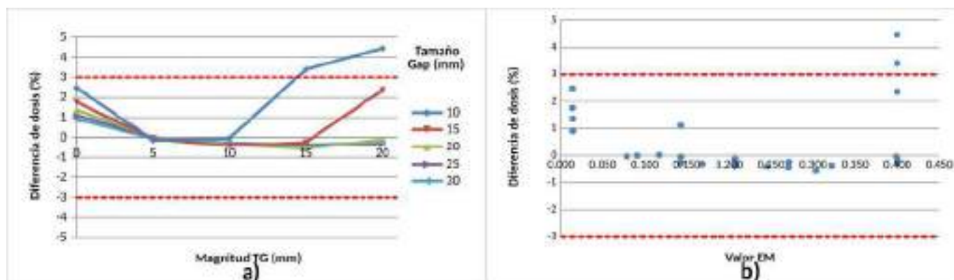
FIGURA 2: Resultados de la comparación de dosis (medida-calculada) para el haz de 6 MV con un DLG de -0.525 mm. (a) Diferencia de dosis frente al LG y el TG. (b) Diferencia de dosis frente al valor EM.
