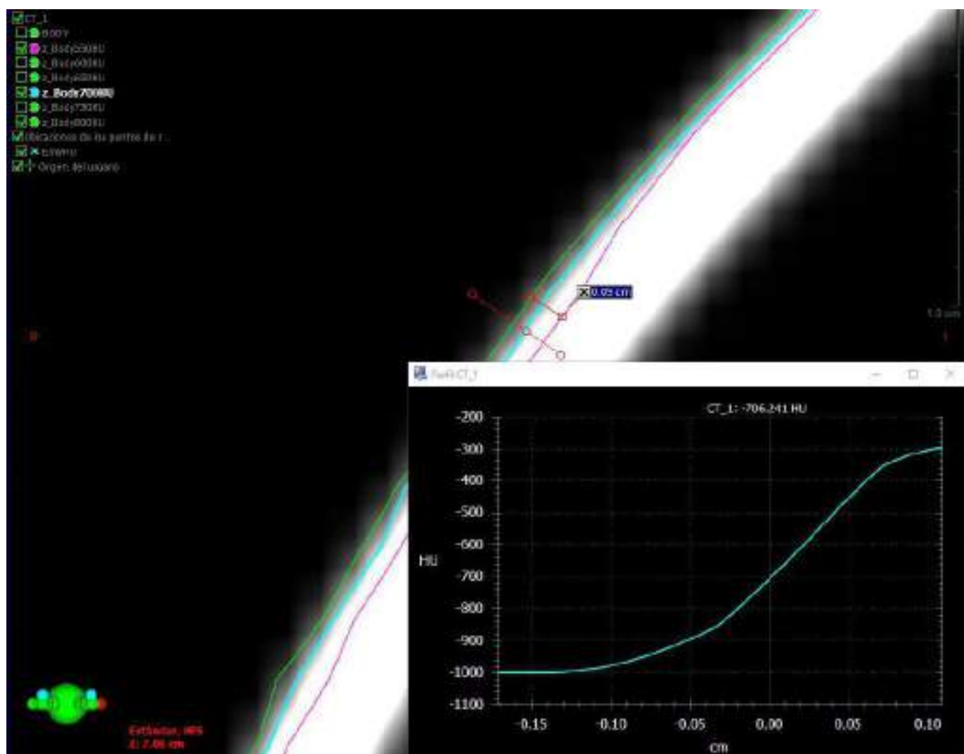
FIGURA 2: Se muestran tres de las superficies generadas. La diferencia de umbral da lugar a distintos tamaños de la superficie creada. Se muestra también un perfil del valor de HU.
