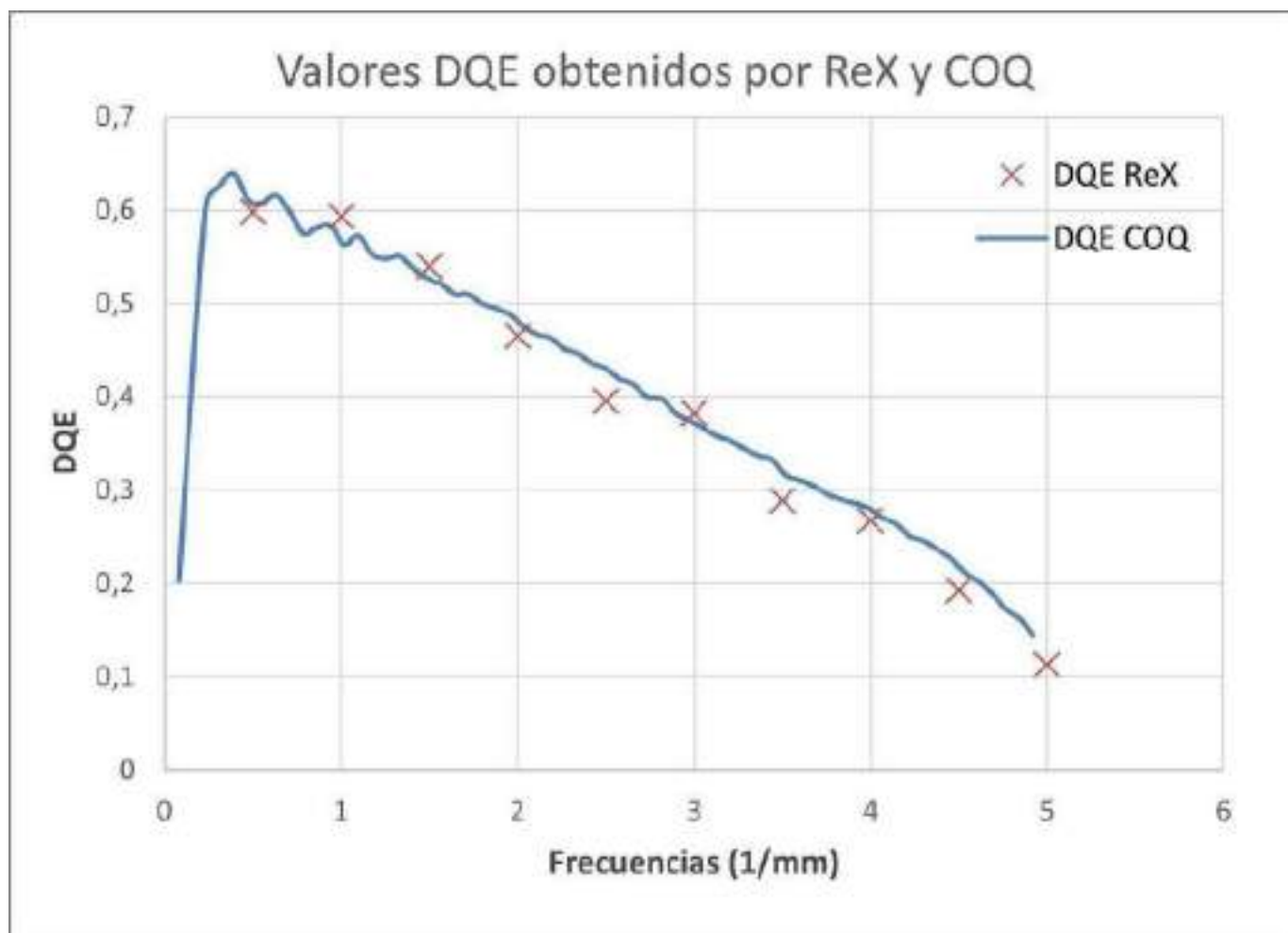
FIGURA 2. Comparación de los valores de DQE (proyección horizontal) por ReX y COQ.
