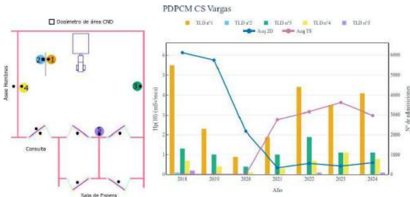
Figura. Plano de colocación de TLDs (izquierda) y evolución temporal de H_p(10) y del nº de adquisiciones (derecha) en el CS Vargas.
