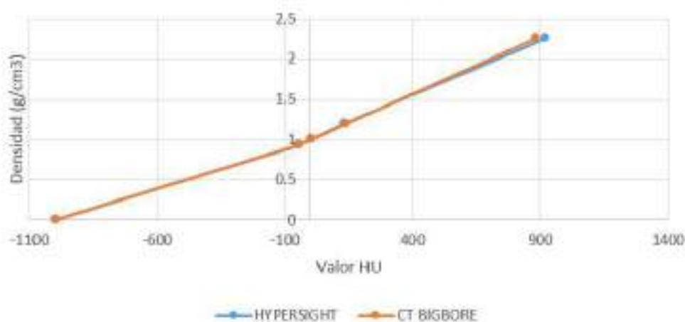
CURVA CALIBRACIÓN CT
