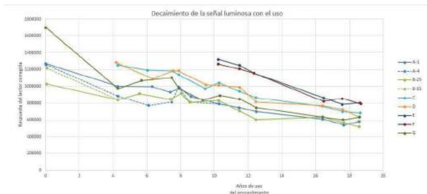
FIGURA 1. (Decaimiento de la señal para las tandas observadas. Nótese subtandas)
