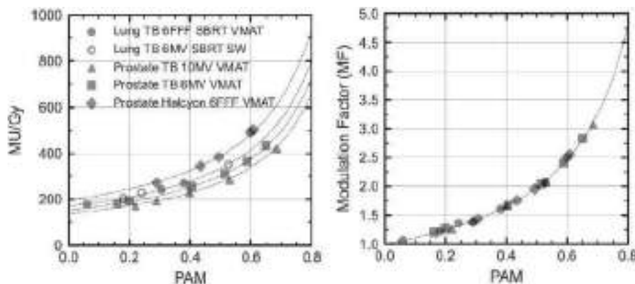
Figura 2. Izquierda: Relación entre UM y PAM para dos casos clínicos considerando diferentes energías y técnicas: Arcoterapia Volumétrica (VMAT), Sliding Windows (SW) y Arcos Conformados Dinámicos (DCA). Las líneas muestran la relación UM-PAM derivada de ecuaciones analíticas. Derecha: Factor de Modulación para los mismos planes, con la línea indicando la predicción teórica en base a las ecuaciones deducidas.
