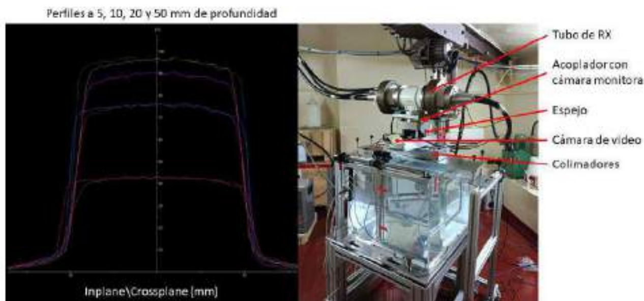
FIGURA 2.-Izq: Perfiles para el campo de 20x20 mm 2 . Dcha: Esquema del sistema colimador durante las medidas con la cuba dosimétrica de agua.
