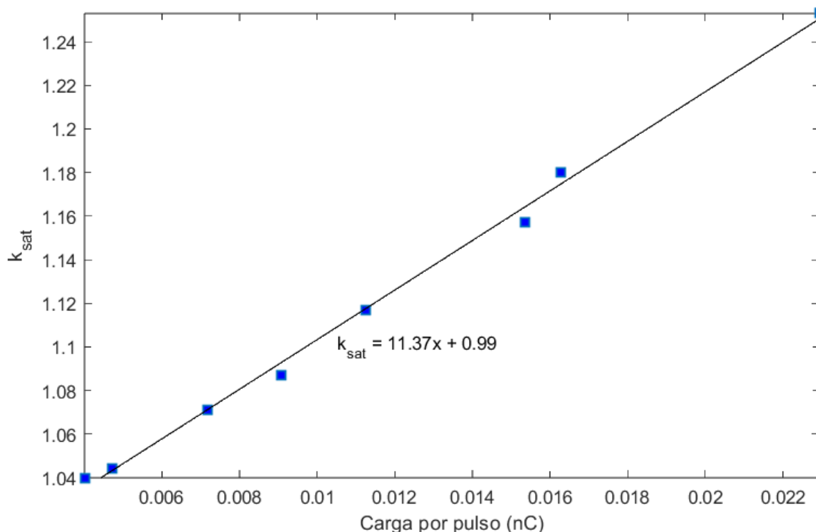
FIGURA 1: Recta de regresión para el cálculo de k_{sat} Cámara PinPoint.
