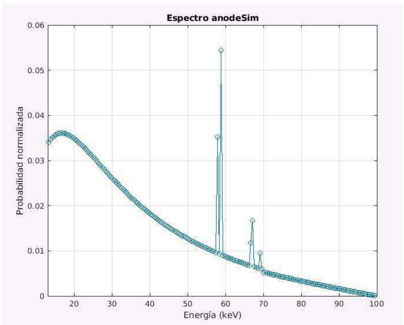
FIGURA 1: Espectro de Rayos X normalizado obtenido con penRed
