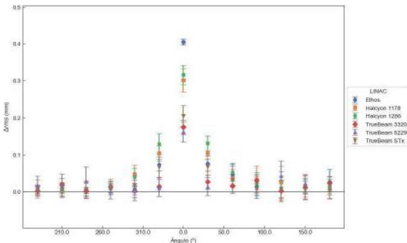
Figura 1. Diferencia en la localización del isocentro entre sentido horario y antihorario en función del ángulo de gantry y para cada LINAC.
