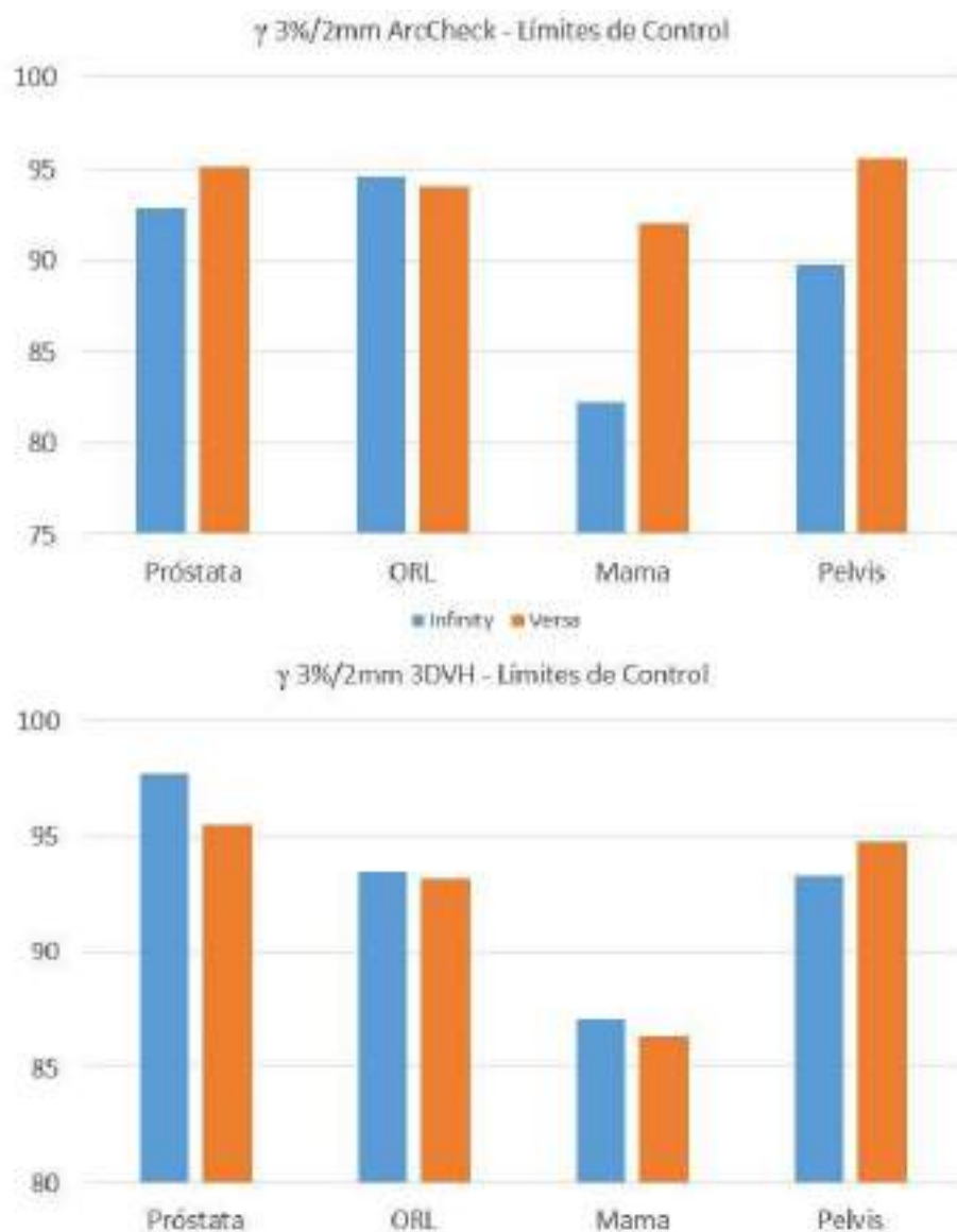
Figura 1. Límites de Control obtenidos para el planificador Roystation para cada uno de los aceleradores y localizaciones analizadas.
