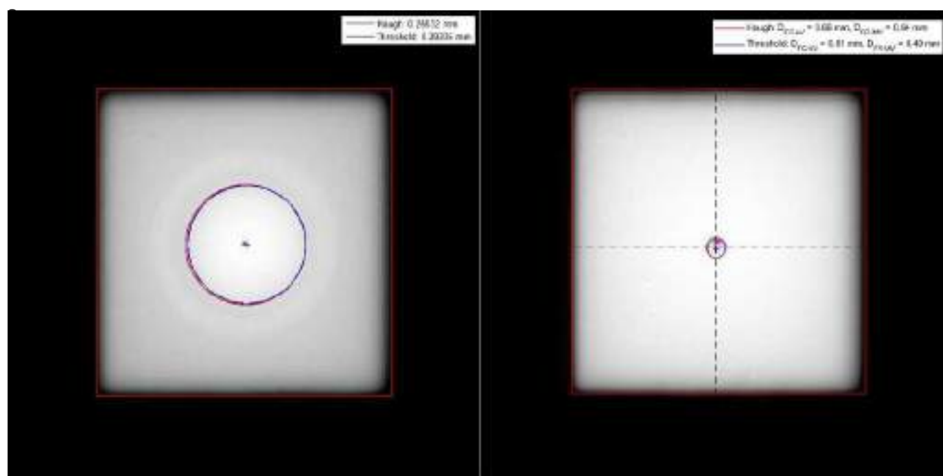
FIGURA 1: Detección del campo de radiación y del círculo central en el maniquí PG (izquierda) e IC (derecha). Los colores distinguen el método empleado.
