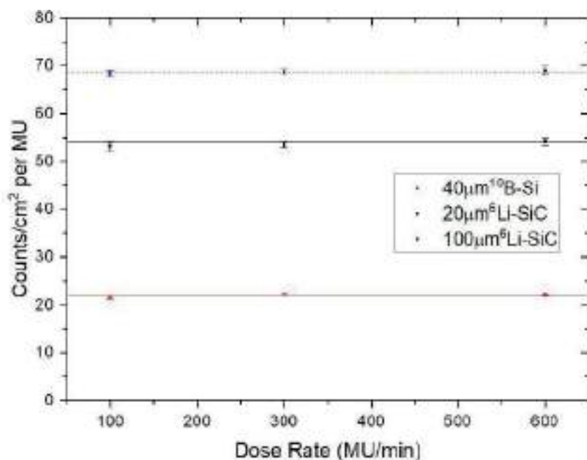
Figure 2. Cuentas por cm 2 por MU en función de la tasa de dosis.
