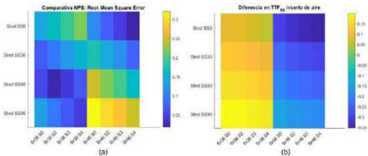
FIGURA 2. (a). Correspondencia entre curvas NPS normalizadas al máximo usando RMSE. (b) Correspondencia entre resoluciones espaciales.
