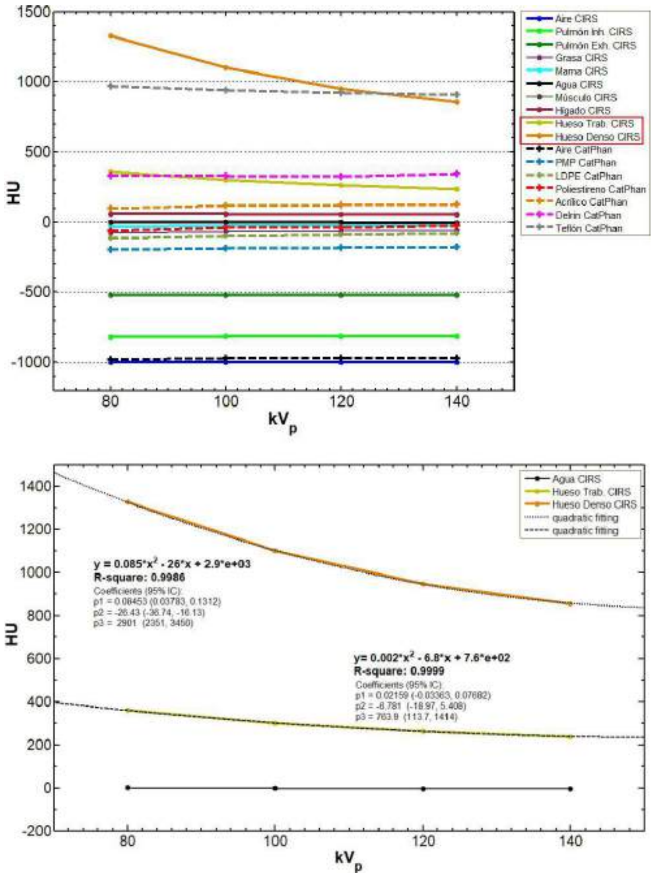
FIGURA 2. Efecto de variar el kV p sobre HU en los tejidos estudiados (arriba), y ajustes polinómicos propuestos en los casos de densidad elevada (abajo).
