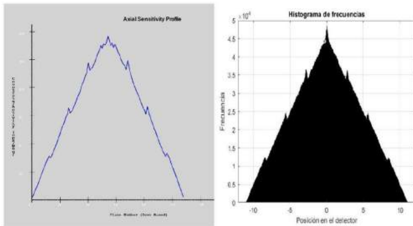
FIGURA 1. Sensibilidad obtenida en medida real (izquierda) y simulada (derecha).
