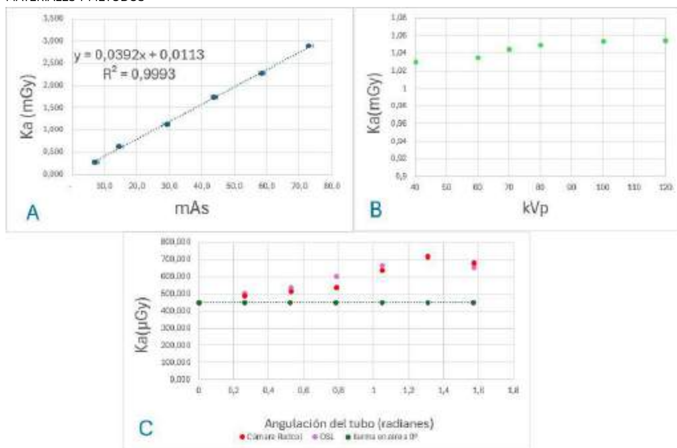
Figura 1. (A) Linealidad con la dosis. (B) Dependencia energética. (C) Dependencia angular.
