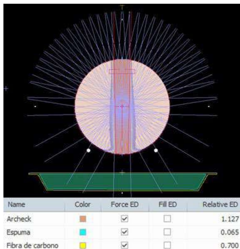
FIGURA 1. Simulación en Montecarlo de la mesa de tratamiento y el maniquí.
