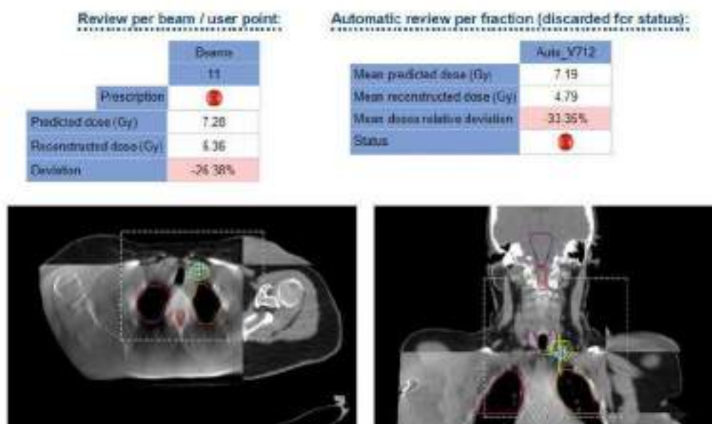
Figura 1. Caso 1: Desviaciones de una de las sesiones de tratamiento junto con el CBCT de esa sesión
