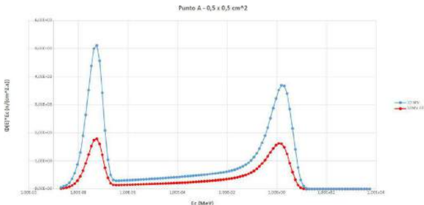
FIGURA 2. Espectro de fluencia de neutrones para un campo de 0.5x0.5 cm 2 .
