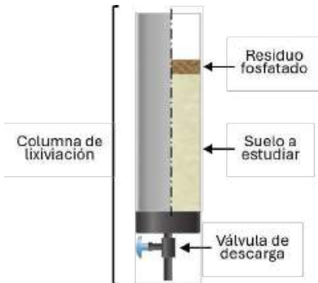
FIGURA 1. Esquema columnas de lixiviación.
