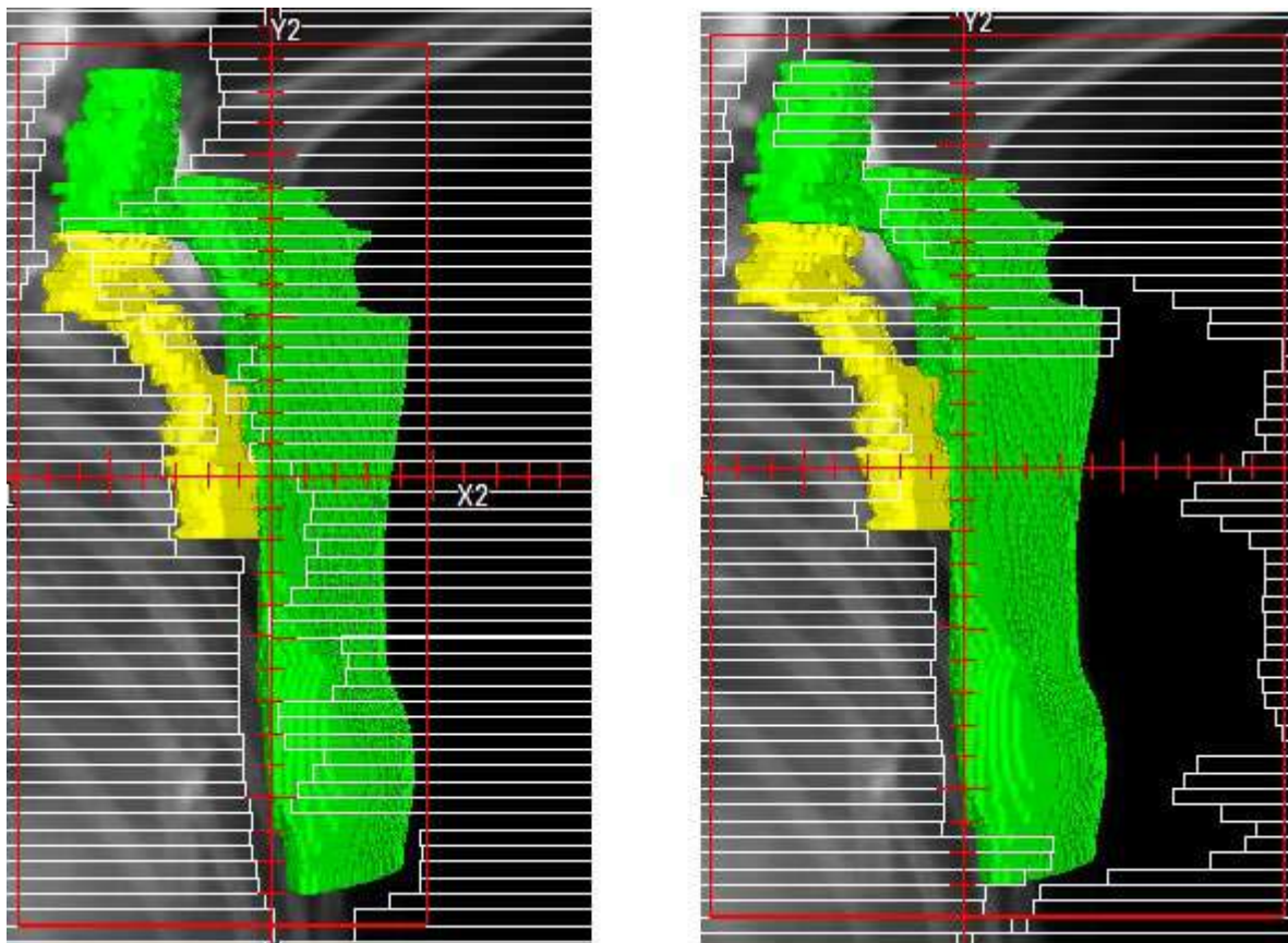
FIGURA 2: Conformación de los campos de tratamiento en un punto de control. A la izquierda, utilizando la estrategia habitual; a la derecha, empleando el método propuesto en este trabajo.
