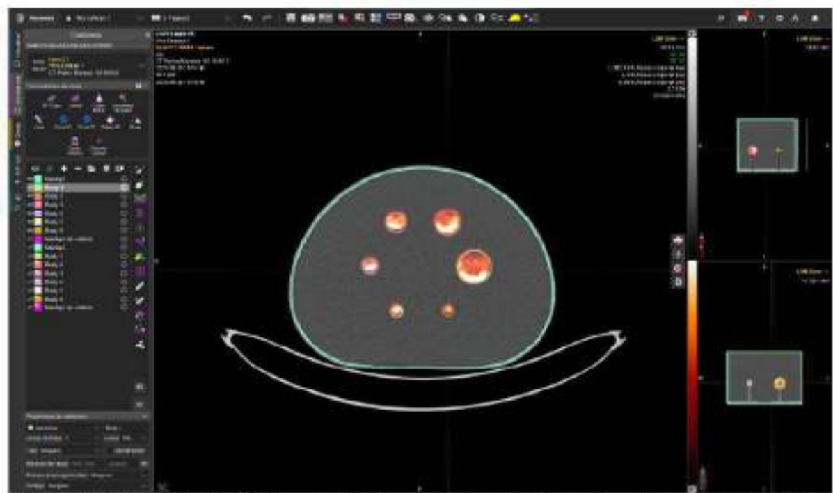
Figura 1. Fusión en MIM NM+CT del maniquí de esferas NEMA, con las esferas rellenas de una disolución de 90 Y.
