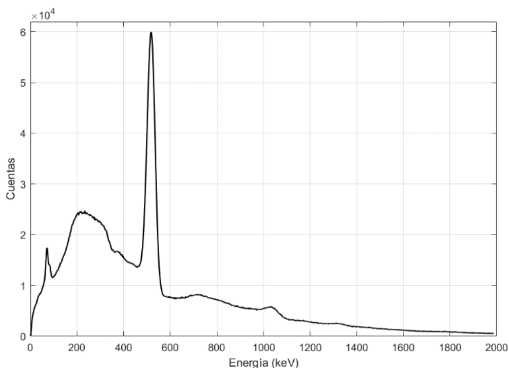
FIGURA 2: Espectro energético tomado 6 minutos tras la irradiación
