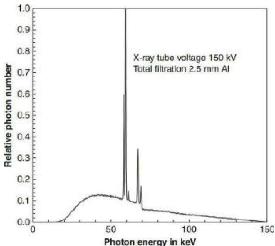
FIGURA 1. Se muestra el espectro de rayos-X obtenido del libro de Horst Aichinger [4].
