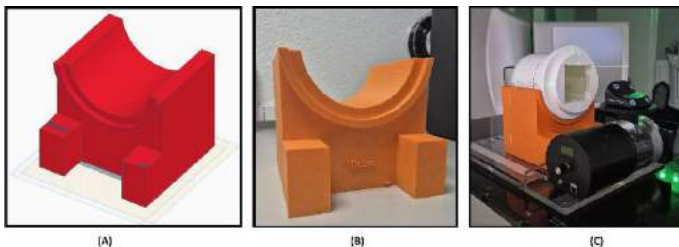
Figura1: (A) Diseño del maniquí. (B) Resultado de la impresión. (C) Montaje del sistema de imagen avanzada con maniquí.
