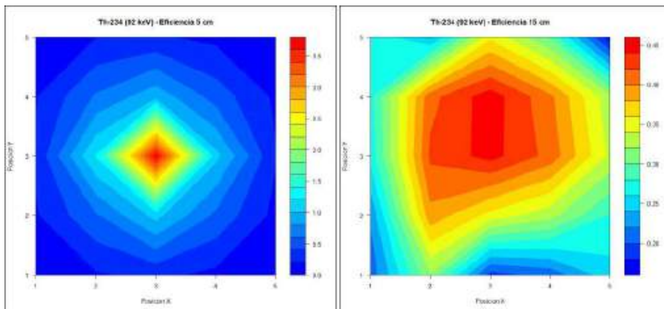
FIGURA 1. Gráficos de superficie para la eficiencia del fotopico de 92 keV del ^{234}\text{Th} para las alturas de 5 cm y 15 cm.
