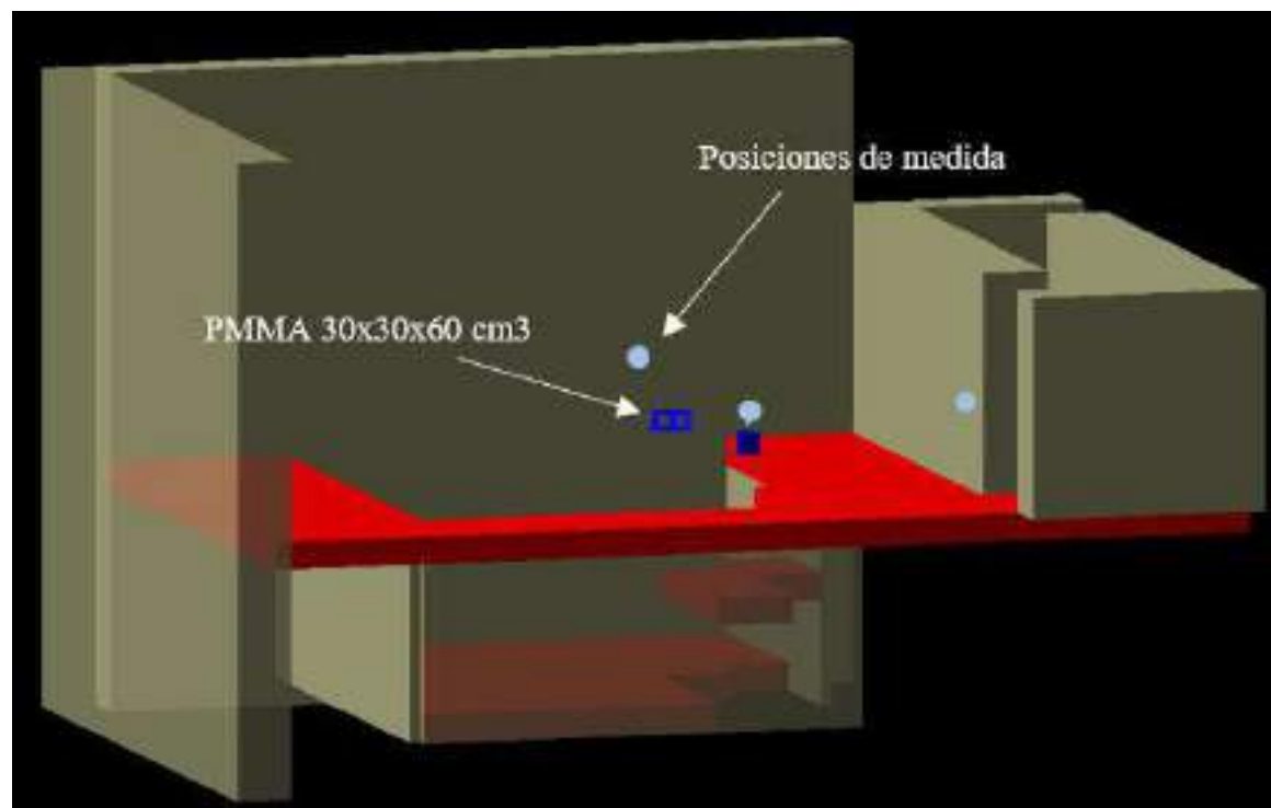
FIGURA 1. Vista esquemática del modelado de la sala de tratamiento de protonterapia en TOPAS.
