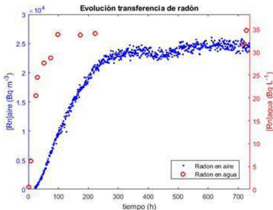
FIGURA 2. Evolución de la transferencia de radón con el tiempo.
