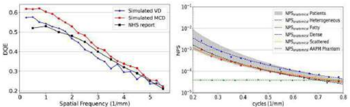
FIGURA 1: Izq-DQE para los dos códigos de detectos (VD y MCD) comparados con los valores del NHS. Dcha-Espectro de potencia radial del ruido anatómico (0.2-0.8 mm 2 ).
