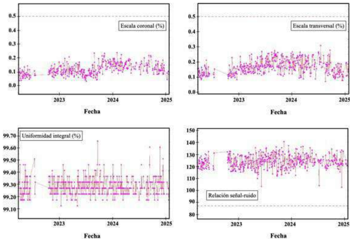
Fig. 1. Variabilidad en el tiempo de varios parámetros del QA diario de la imagen MRI en un MR-Linac.
