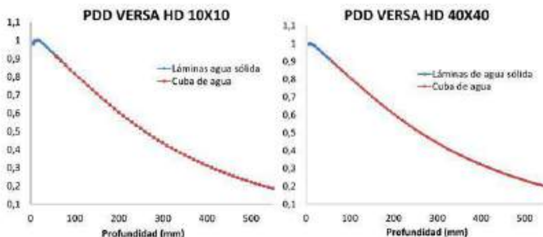
Figura 2. Curvas de PDDs. En color azul, las medidas con láminas de agua sólida y en color rojo con la cuba MP3.
