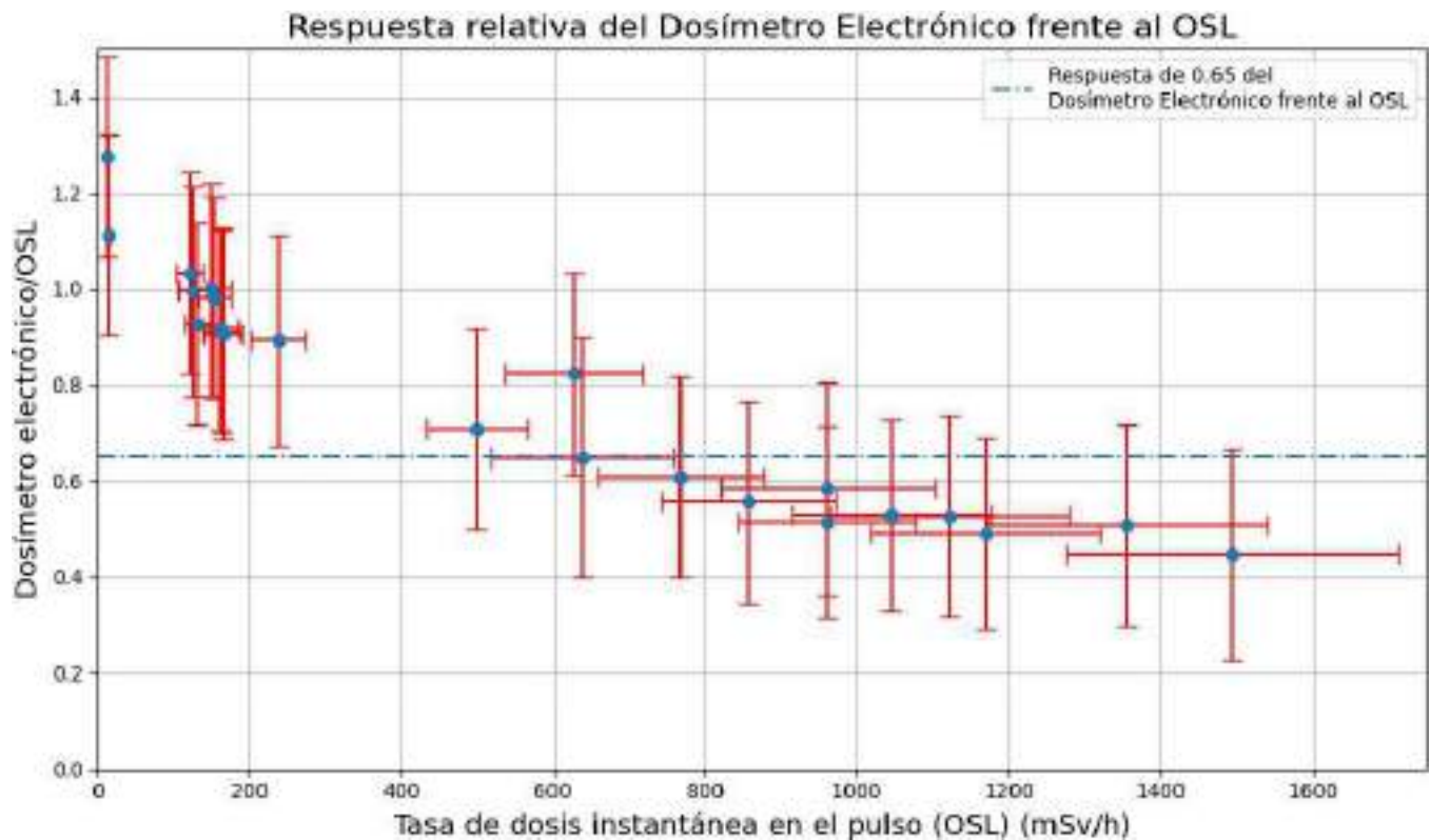
Gráfico 1. Respuesta relativa del dosímetro electrónico frente al OSL respecto a la tasa de dosis instantánea calculada del OSL. La línea punteada representa el umbral por debajo del cual las medidas no son cuantitativas.
