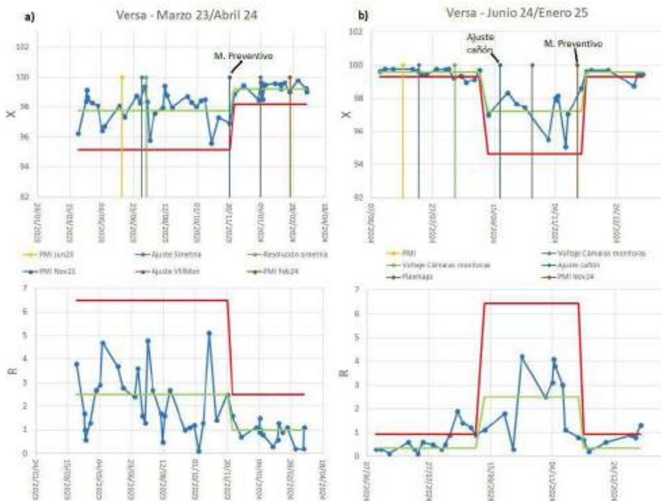
Figura 2. Gráficas de control X-R para el acelerador Versa en ambos periodos. Se observan el limite central (verde) y los limites de control inferior y superior (rojo). Se marcan en la gráfica X las intervenciones realizadas en el acelerador. Se resaltan los eventos a partir de los cuales se han producido cambios.
