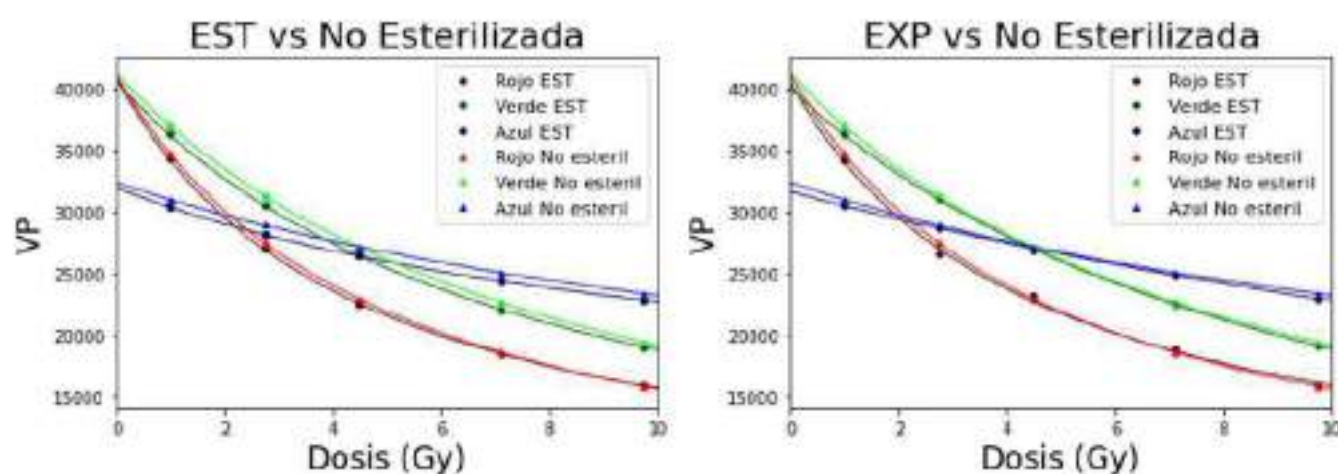
Figura 2. Comparación entre curvas de calibración obtenidas con películas esterilizadas y no esterilizadas para los tres canales del escáner (rojo, verde y azul). En la izquierda se presenta el resultado obtenido para el ciclo de esterilización estándar (EST) y en la derecha el obtenido por el ciclo de esterilización exprés (EXP). Las barras de error no se muestran para facilitar la visualización, con valores entre 30 y 40 PV.
