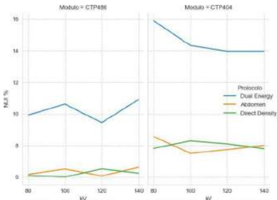
Figura 2. Non-Uniformity Index (NUI) de los protocolos DD, DE, y ABD para diferentes kilovoltajes. A la izquierda los valores de NUI para el módulo de uniformidad del Capitan y a la derecha para el módulo de materiales.
