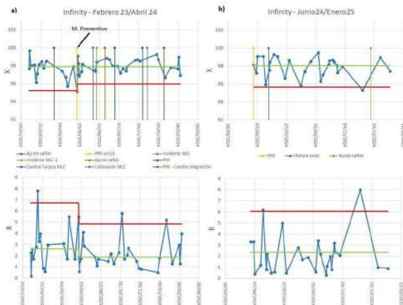
Figura 1. Gráficas de control X-R para el acelerador Infinity en ambos periodos. Se observan el límite central (verde) y los límites de control inferior y superior (rojo). Se marcan en la gráfica X las intervenciones realizadas en el acelerador. Se resaltan los eventos a partir de los cuales se han producido cambios.
