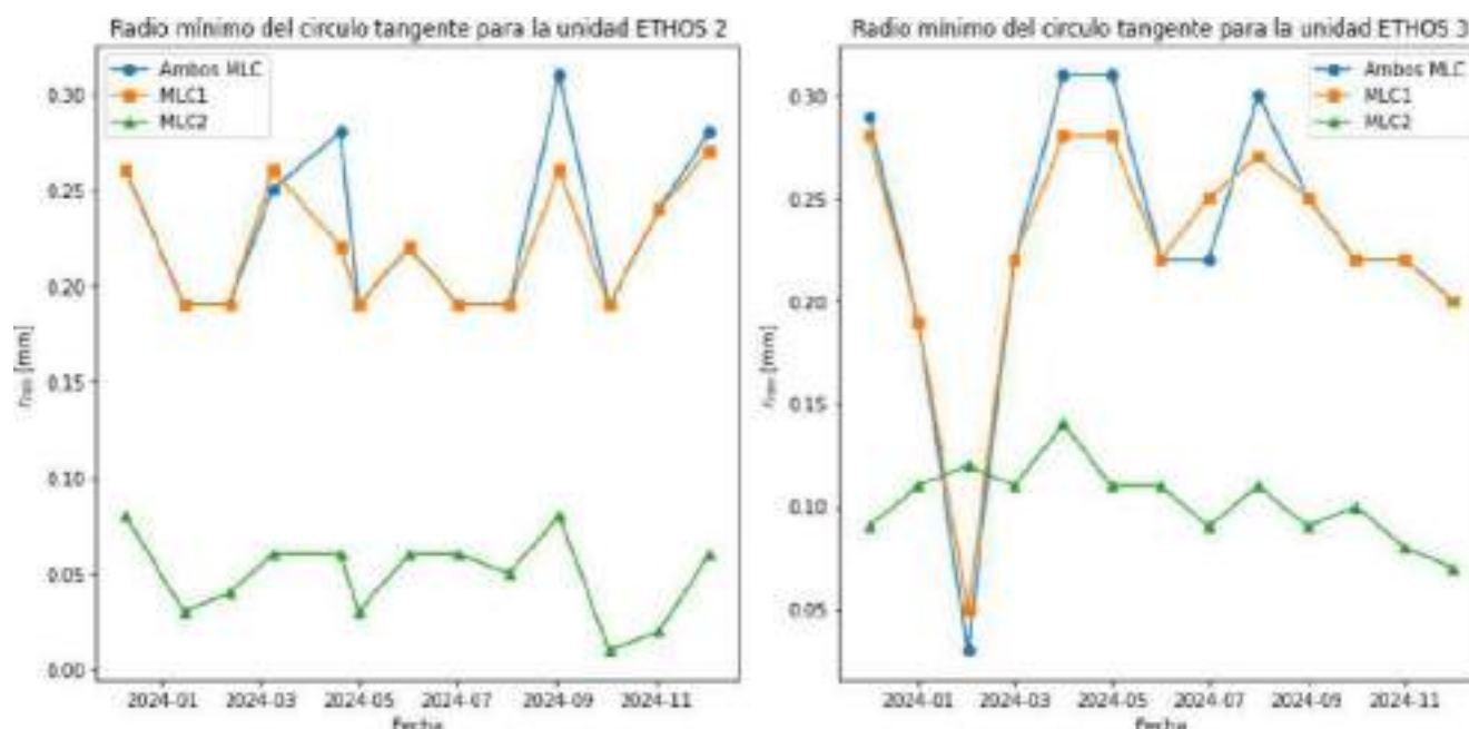
FIGURA 2. Representación gráfica de los valores del radio mínimo del círculo tangente a lo largo de un año para dos unidades de tratamiento ETHOS diferentes.
