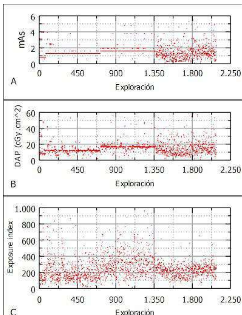
FIGURA 2: Evolución temporal del DAP, mAs e IE en función del número de exploración. La fecha de introducción del S-AEC corresponde con la marca 1350 en el eje X
