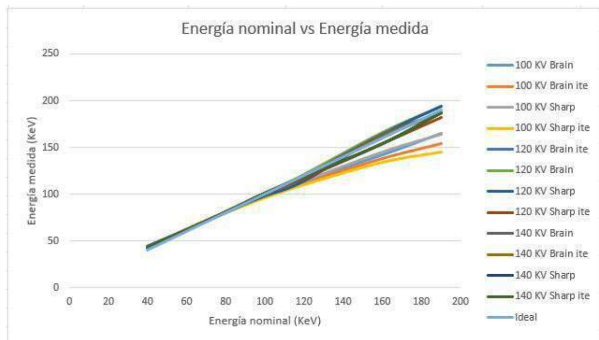
Gráfico 1: Relación entre Energía nominal frente a la energía medida
