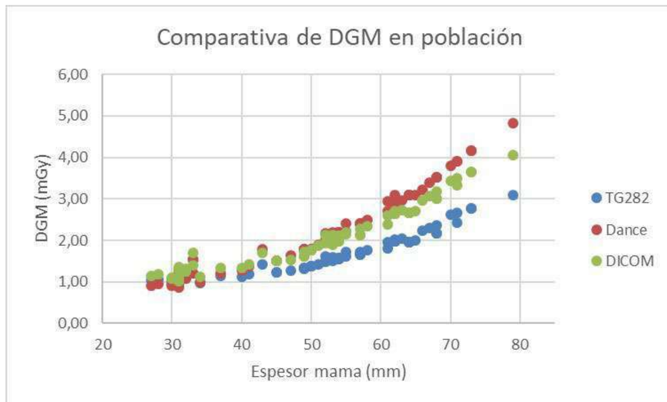
FIGURA 2. Comparativa de DGM en la población para DBT y proyección craneocaudal
