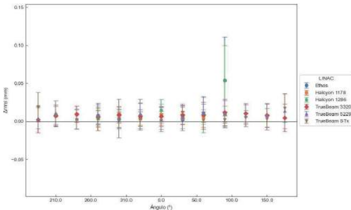
Figura 2: Diferencia en la localización del isocentro entre sentido horario y antihorario en función del ángulo de colimador y para cada LINAC.
