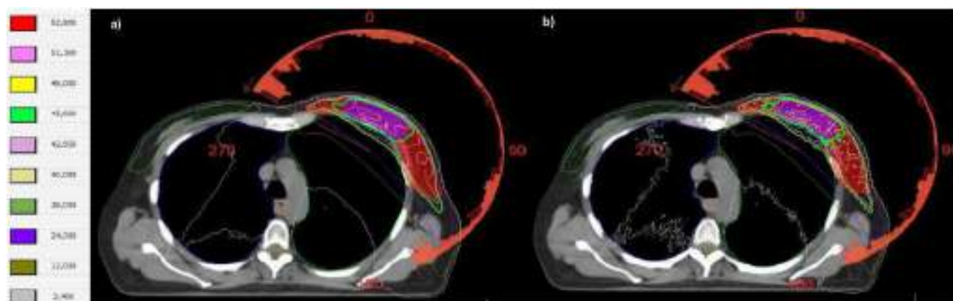
FIGURA 2: a) y b) diferencia de indicadores dosimétricos relativos a incertidumbre 1% (PTV y mama contralateral respectivamente). c) Índice gamma de verificación pretratamiento frente a incertidumbre.
