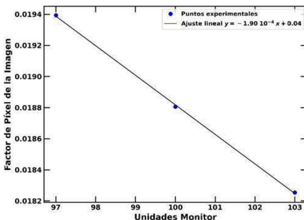
Fig. 1. Curva de calibración EPID.
