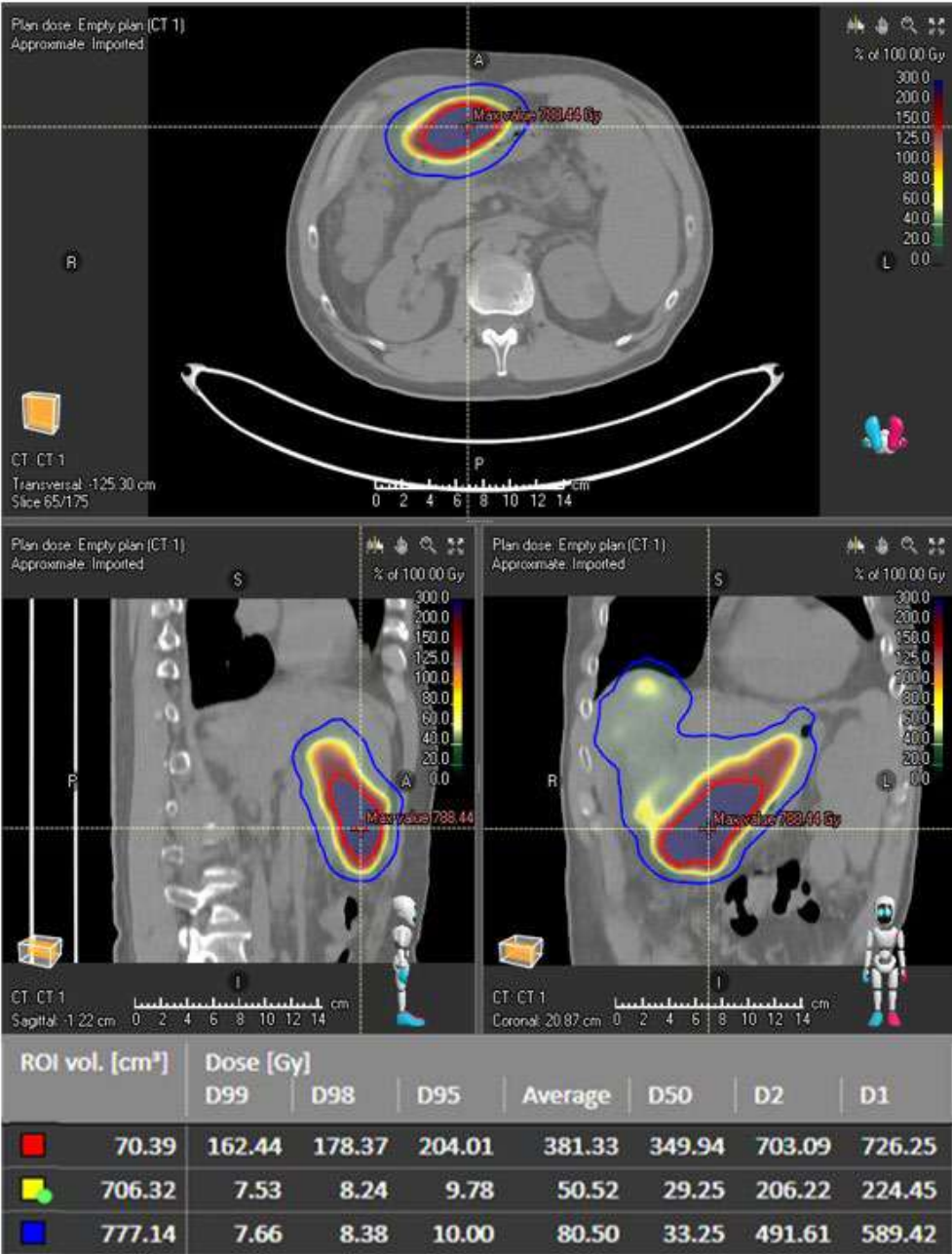
Figura 1: Distribución de dosis en el planificador Raystation.
