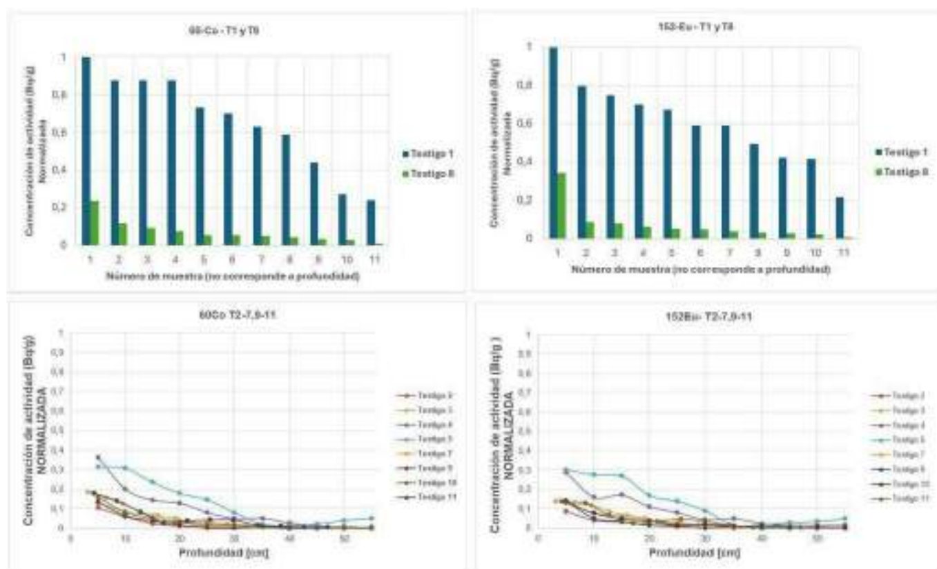
FIGURA 2 Resultados de los testigos de hormigón
