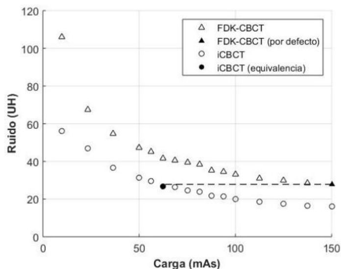
Figura 1. Caracterización del ruido de imagen (UH) basado en la carga (mAs) utilizando el maniquí Catphan para los dos algoritmos de reconstrucción.
