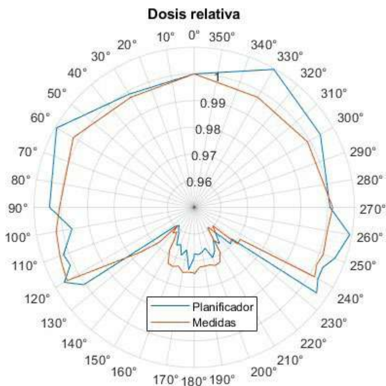
FIGURA 2. Dosis relativa en función del ángulo de incidencia.
