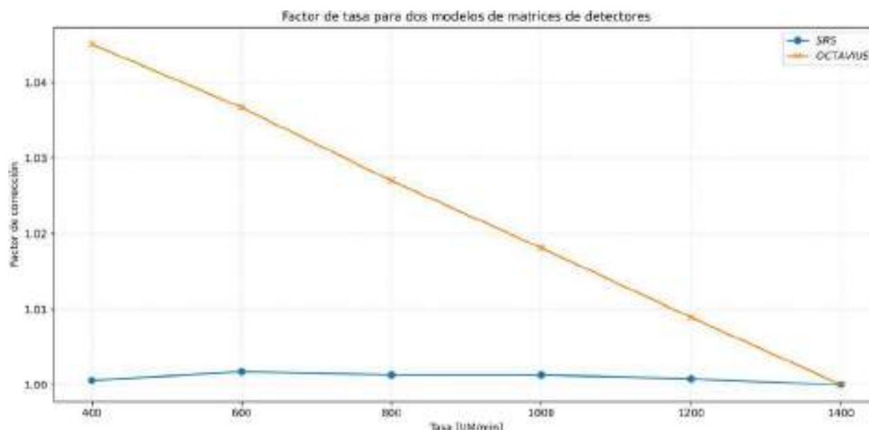
FIGURA 1: Factor de corrección de ambas matrices de detectores entre las lecturas a tasa de 1400 UM/min y valores menores.
