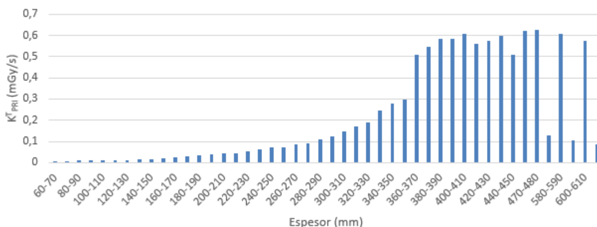
FIGURA 2. Tasa de kerma en punto de referencia intervencionista, \dot{K}_{PRI} , frente espesor equivalente de paciente para baja tasa y 7.5 pulsos/s.
