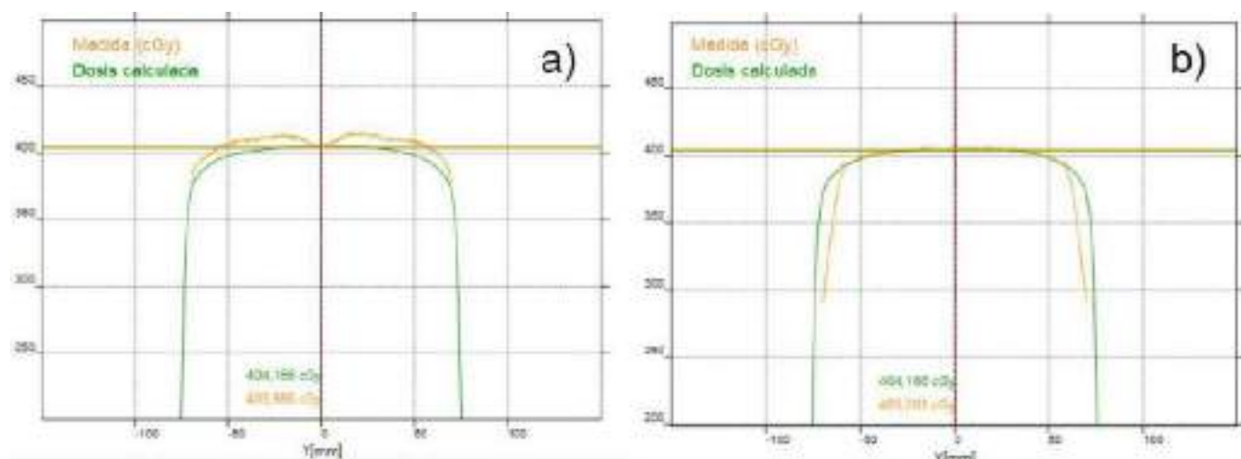
FIGURA 1. Perfil Y para 6X, aplicando la corrección de uniformidad de: a) fábrica b) usuario.
