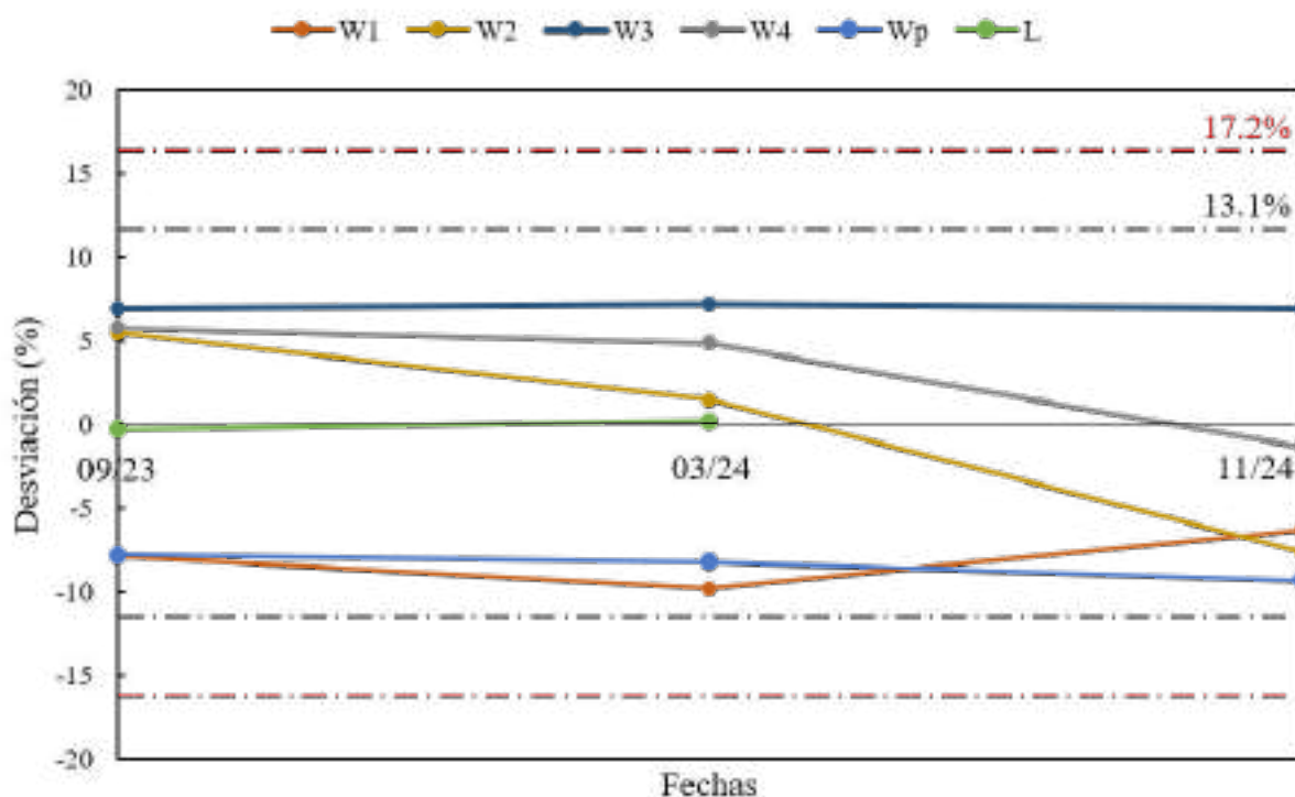
FIGURA 2. Evolución temporal de los resultados de la verificación de detectores.
