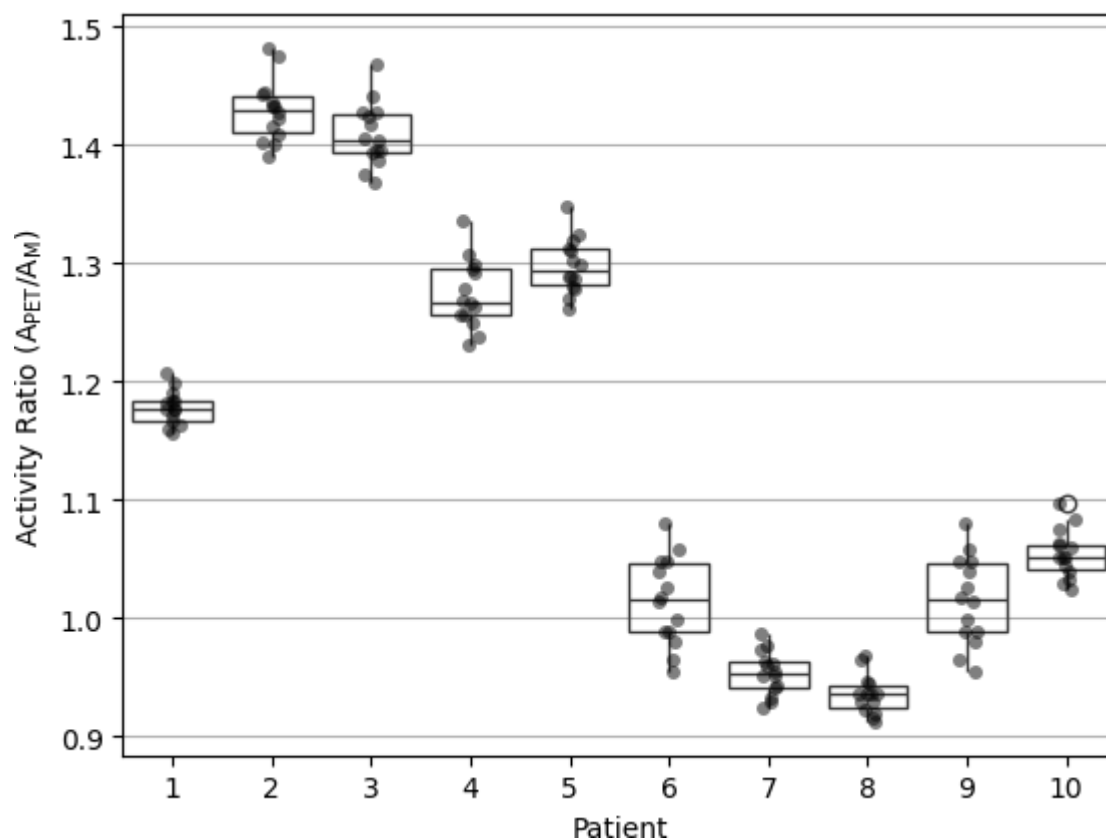
FIGURA 1: Distribución de los cocientes APET/AM para 10 pacientes. 1-6 corresponden a esferas de resina, 7-10 a vidrio.
