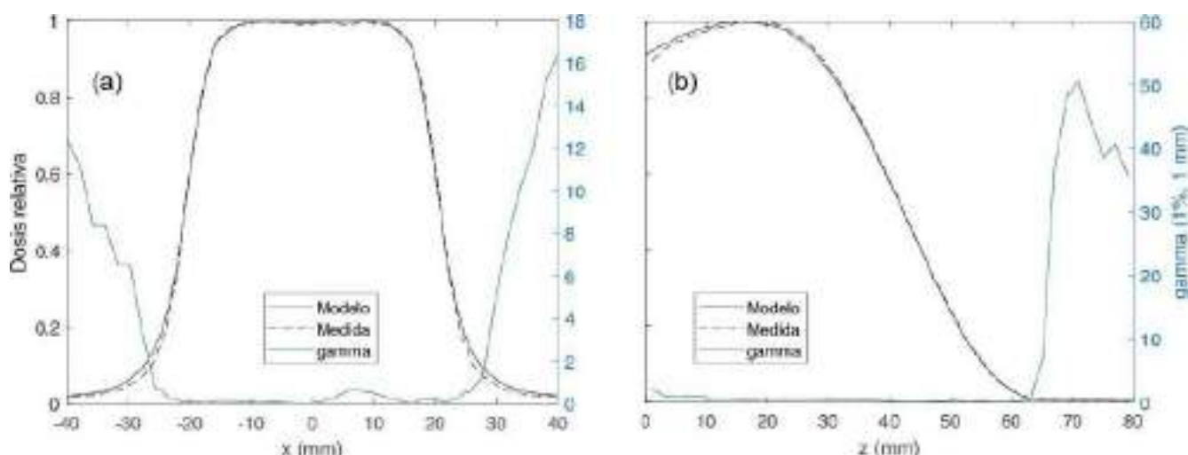
FIGURA 1: Comparación y análisis gamma de TPD (a) y PDD (b) para el aplicador de 4 cm, bisel 0° y energía 12 MeV.
