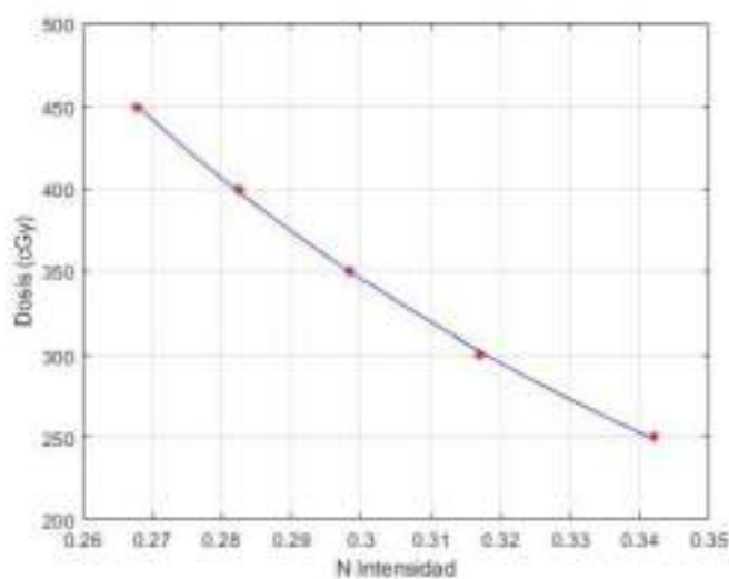
Figura 1. Película radiocrómica utilizada, programa y curva ajustada.
