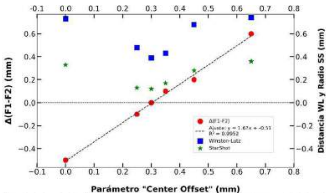
Figura 2. Resultados obtenidos para las diferentes pruebas. En el eje izquierdo \Delta representa el valor del desplazamiento de la semi-hendidura F1 respecto de F2 (método propuesto, círculo). En el eje derecho se muestran los valores de la distancia entre isocentro mecánico y de radiación el test de Winston-Lutz (cuadrado) y el radio del círculo obtenido con la prueba de estrellas de colimador (estrella).
