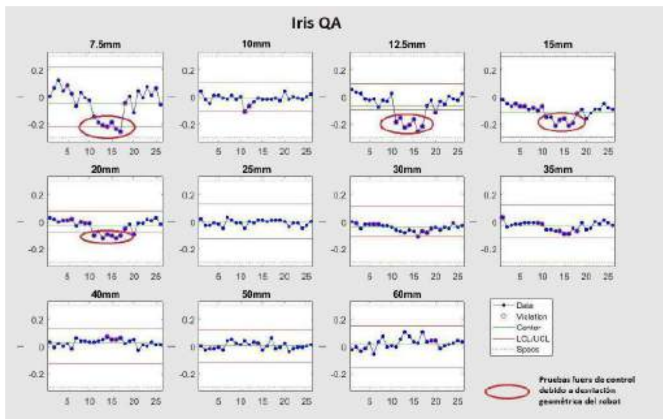
Figura 1. Gráficos de control de la prueba Iris QA. Se pueden ver resaltadas las pruebas fuera de control que eran causadas por una desviación geométrica del equipo.
