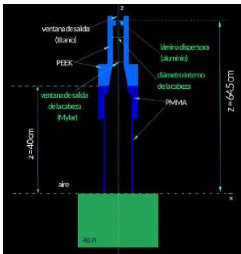
FIG. 1 Esquema de la geometría modelada del acelerador Liac HWL.
