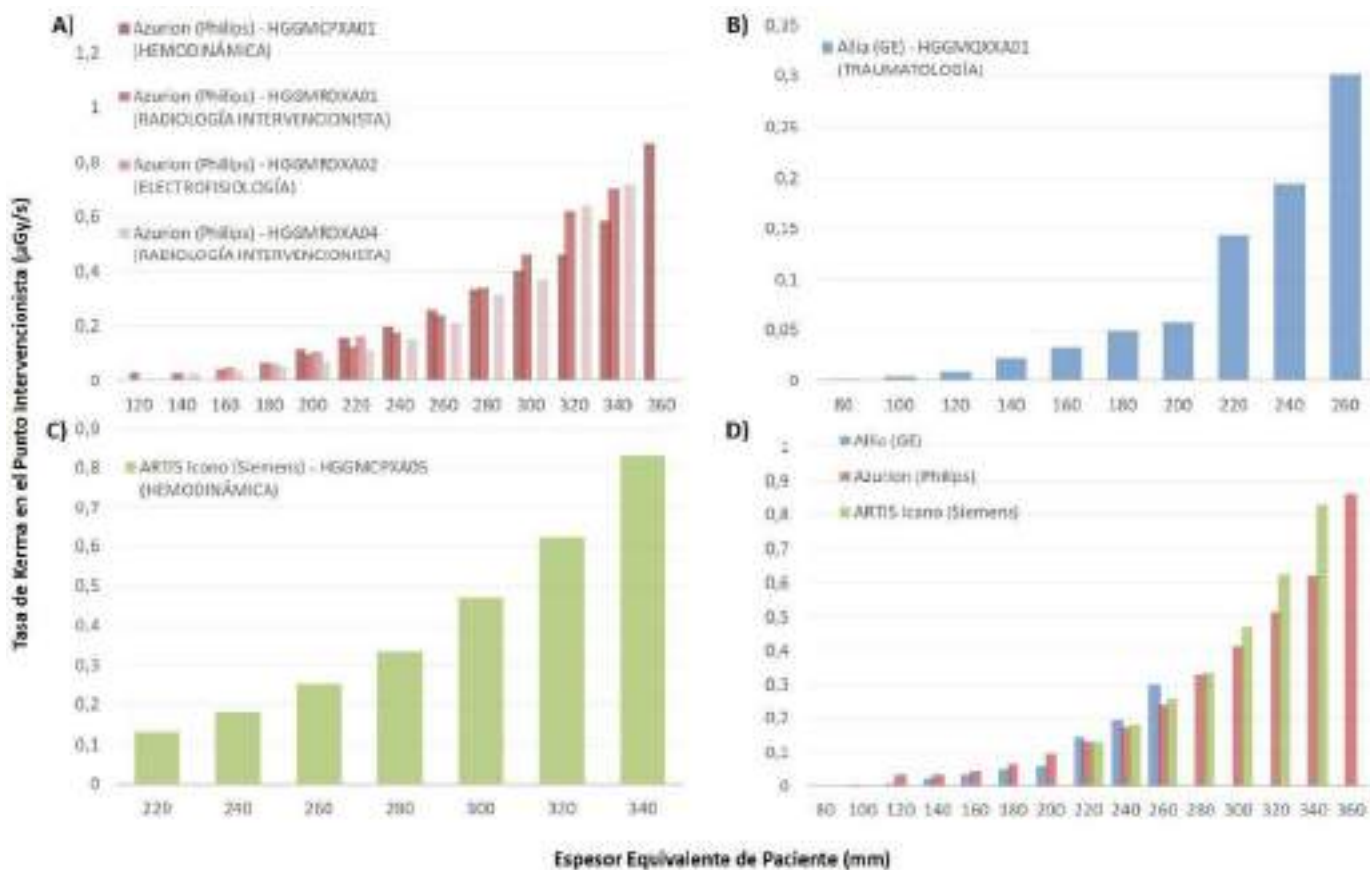
FIGURA 1. \dot{K}_{a,r}(d) de los tres modelos considerados (en abscisas se indica el centro de cada intervalo): A) Azurion (Philips), B) Allia (GE), C) ARTIS Icano (Siemens), D) total agrupado por fabricante.
