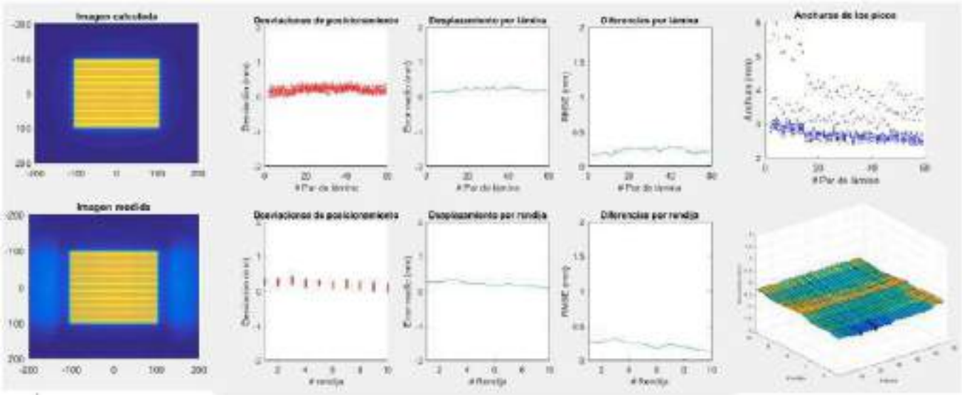
FIGURA 1. Resultados de la rutina de Matlab para el Fence Test.
