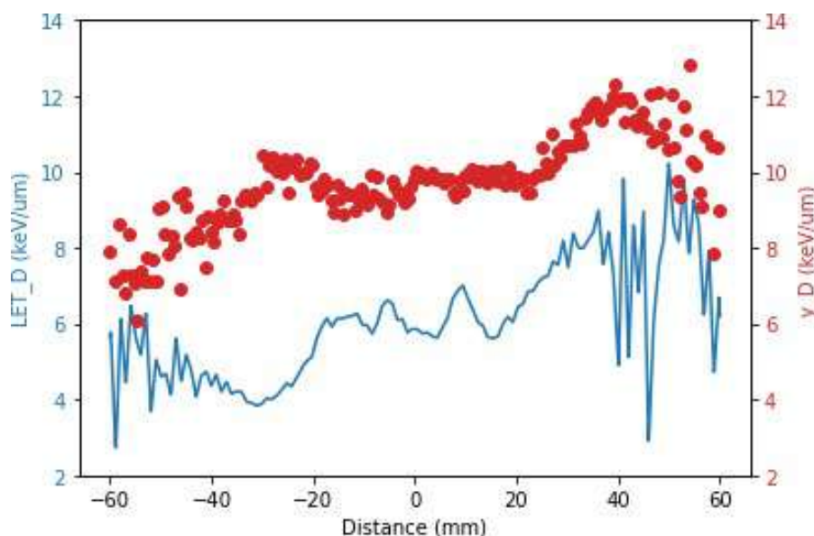
Fig 2. Comparación de los valores de LET_D simulados en el paciente por RayStation (azul) con los valores experimentales de baryD en los microdetectores de silicio (rojo) para la dosis distal del 75%.
