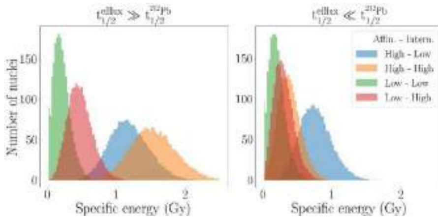
FIGURA 1. Distribución de energía específica en las células para diferentes perfiles cinéticos, para un tiempo de excreción mucho mayor o mucho menor que la semivida del Pb-212.
