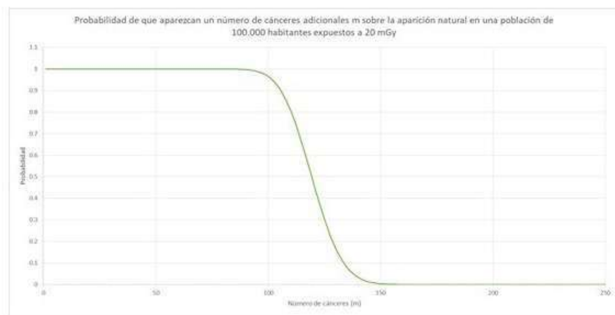
FIGURA 1.- Probabilidad de que aparezcan un número de cánceres m sobre la natural en una población de 100.000 personas, con características similares a la española, expuestas a 20 mGy.
