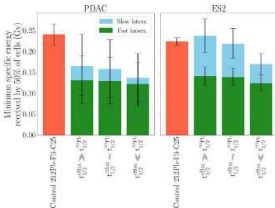
FIGURA 2. Energía específica mínima absorbida por el 50% de las células en varios escenarios simulados los dos experimentos simulados con TOPAS.
