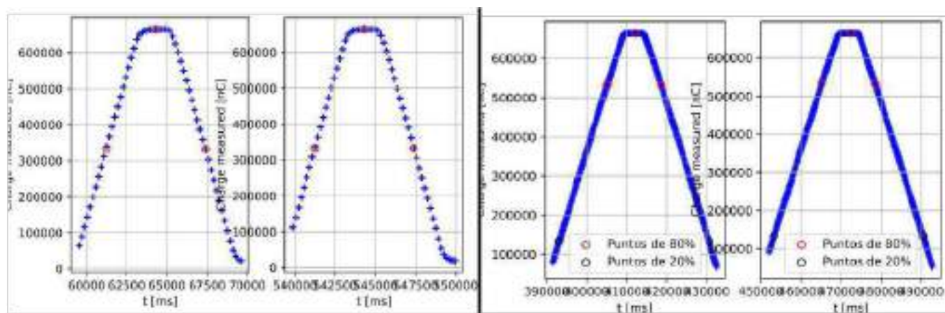
Imagen 2: dos de las gráficas generadas por el programa. Gráfica de Precisión temporal (a la izquierda pico A y a la derecha, el G) a la izquierda y Barrido de mordaza (a la izquierda pico D, y a la derecha pico E) a la derecha.
