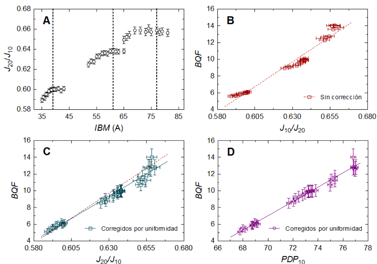
Figura 1. (A) Valores del cociente J_{20}/J_{10} determinados a partir de las curvas de rendimiento en profundidad en agua en función de la corriente de bending magnet del acelerador; las líneas de trazos verticales indican el valor de la corriente de funcionamiento usual. (B) Valores del factor de calidad obtenidos mediante el dispositivo QuickCheck frente al cociente J_{20}/J_{10} cuando no se realiza corrección por uniformidad, junto con el ajuste lineal a los datos experimentales. (C) Valores del factor de calidad frente al cociente J_{20}/J_{10} cuando se hace corrección por uniformidad, junto con los ajustes lineales a los datos experimentales con y sin corrección por uniformidad (líneas continua y de trazos, respectivamente). (D) Valores del factor de calidad frente al rendimiento a 10 cm en agua corregidos por la falta de uniformidad y ajuste lineal a los datos experimentales.
