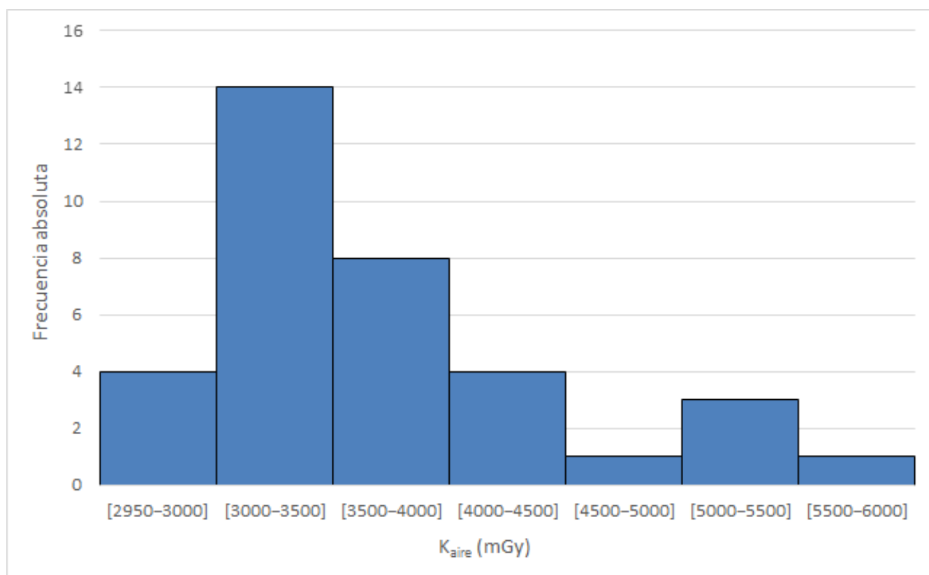
FIGURA 2. Histograma del kerma en aire registrado en las intervenciones que superaron el NN.
