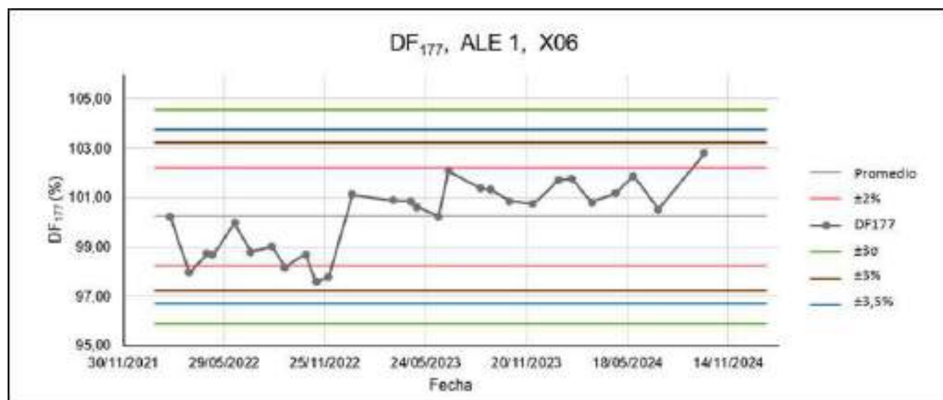
FIGURA 1: Datos del acelerador 1 para DF177, medida con energía de 6 MV.
