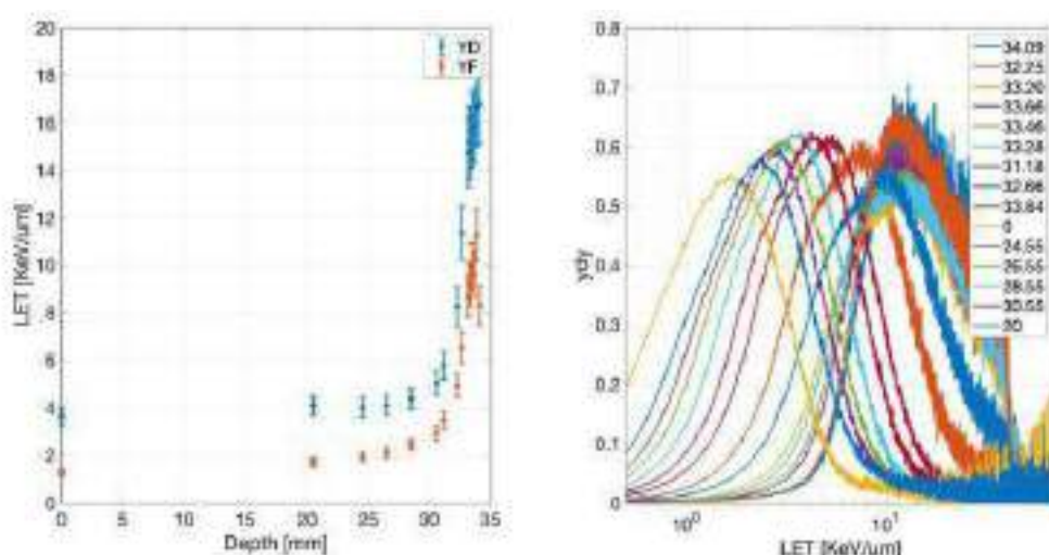
Figura 2. Medidas obtenidas con el detector microdosimétrico MicroPlus Probe con un haz de protones de 70.2MeV del sistema ProBeat-CR en la CUN utilizando bloques de PMMA. A) Valor medio de LET en función de la profundidad de PMMA atravesada. En azul, los valores correspondientes a la energía lineal promedio dosimétrica. En rojo, los valores correspondientes a la energía lineal promedio estadística. B) Espectro microdosimétrico ( y \cdot dy ) en función de LET. El color de la curva corresponde a la profundidad de PMMA atravesada (mm)
