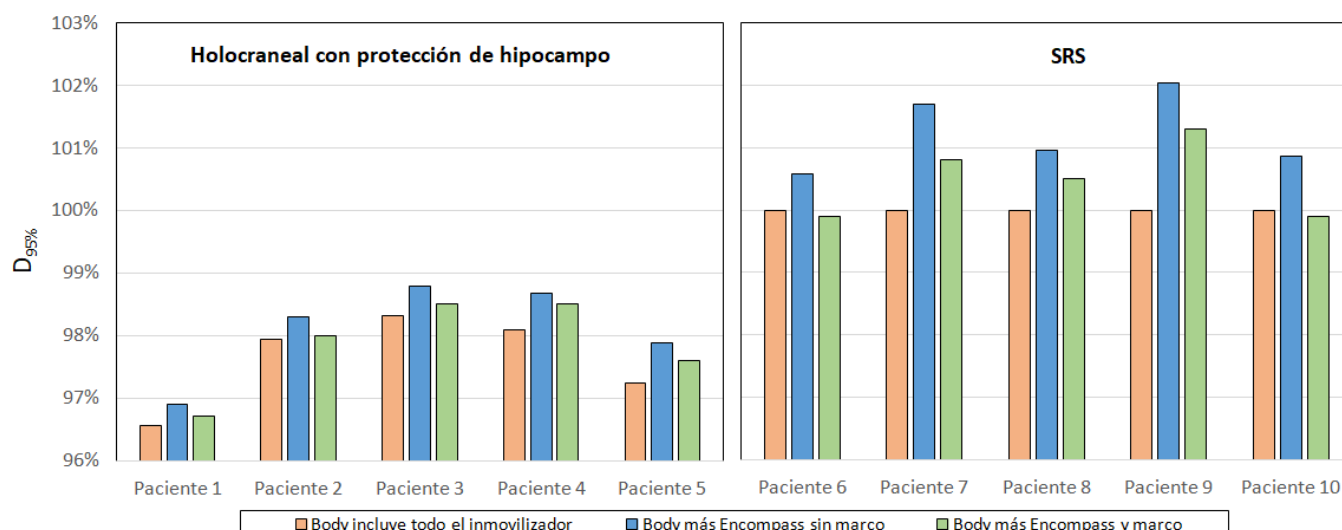
Figura 2. D_{95\%} para cada uno de los casos analizados. Izquierda: Casos de WBHP. Derecha: Casos de SRS
