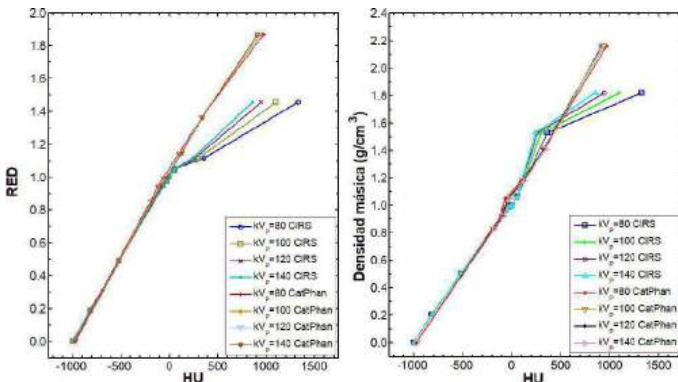
FIGURA 1. Relaciones HU-RED (izquierda) y HU-densidad másica (derecha) obtenidas por maniqué, variando exclusivamente el kV_p .
