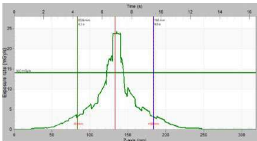
Figura 1: Perfil de dosis medido con la sonda CT Dose Profiler. Colimación=20 mm y Pitch=0,969.
