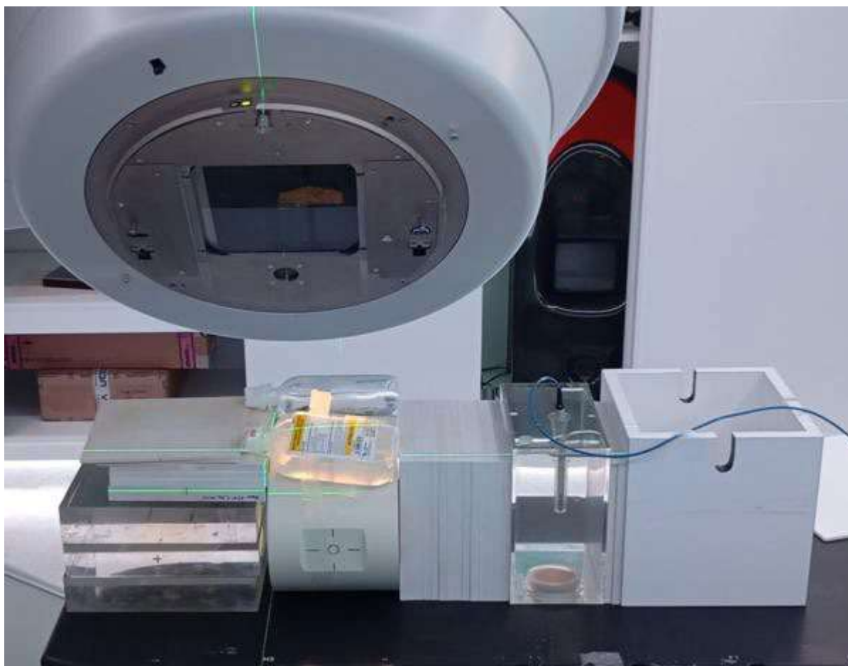
Figura1: Configuración experimental para simular la anatomía de la paciente con maniqués de PMMA y RW3.
