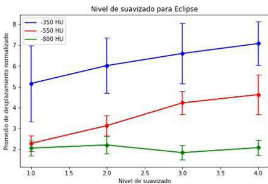
FIGURA 2: Análisis del suavizado para tres umbrales de HU (-350HU, -550HU y -800HU) utilizados para generar el BODY en Eclipse.
