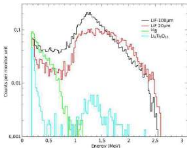
Figure 1. Comparativa de los espectros obtenidos para diferentes capas de conversión con el detector SiC.
