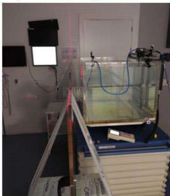
Figura 2. Montajes experimentales
